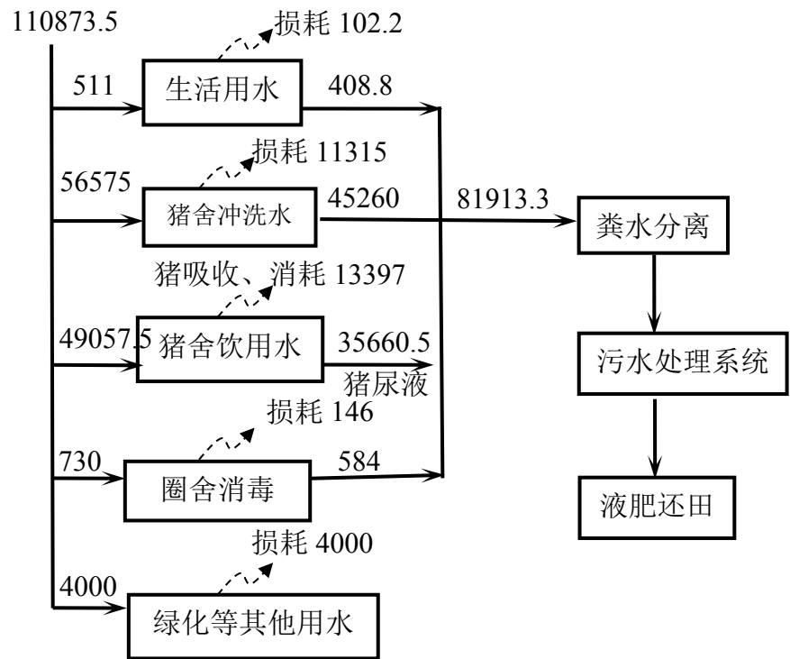
图 3.1-1 项目水量平衡图(单位: m³/a)
