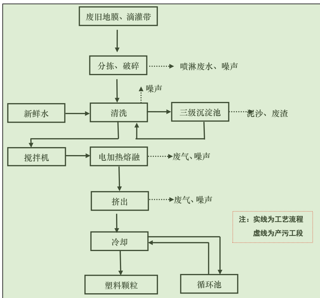
图 3.3-1 本项目造粒生产线工艺流程及产污环节
