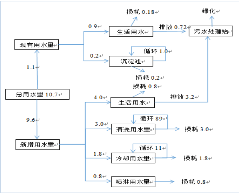
图3.5-1 全厂水平衡图
