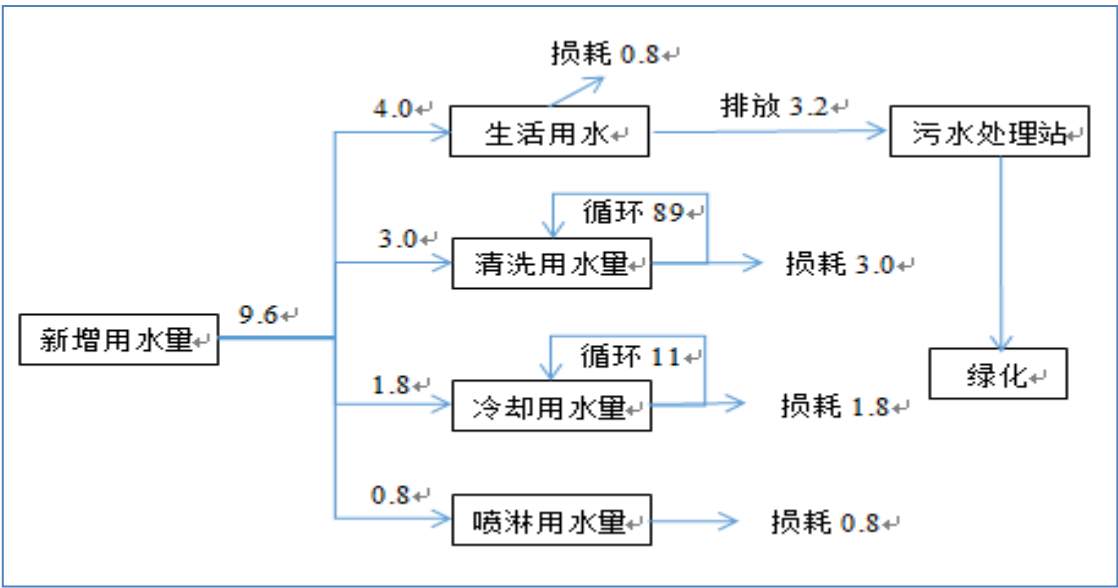
图 3.3-2 项目水平衡图
