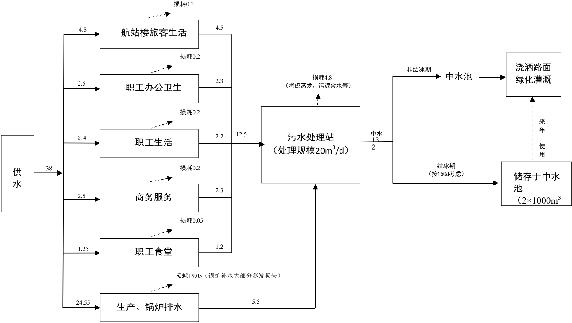
图 2.4-1 机场目标年水平衡图 ( \text{m}^3/\text{d} )
