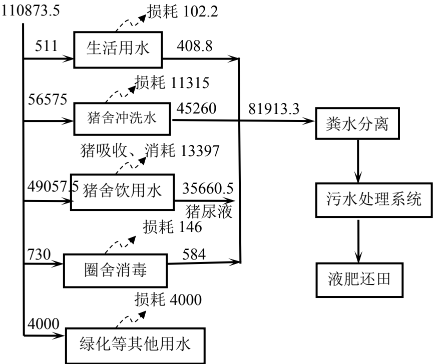
图 3.1-1 项目水量平衡图(单位: m³/a)
