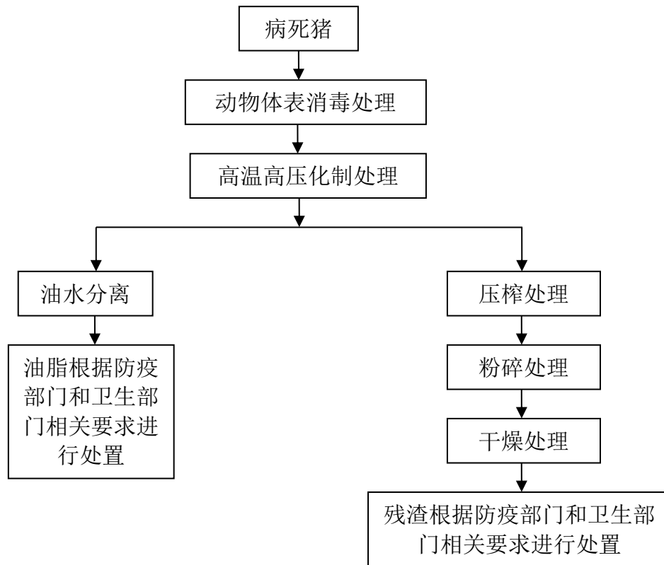
图3.1-7 项目病、死猪尸体无害化处理工艺图
