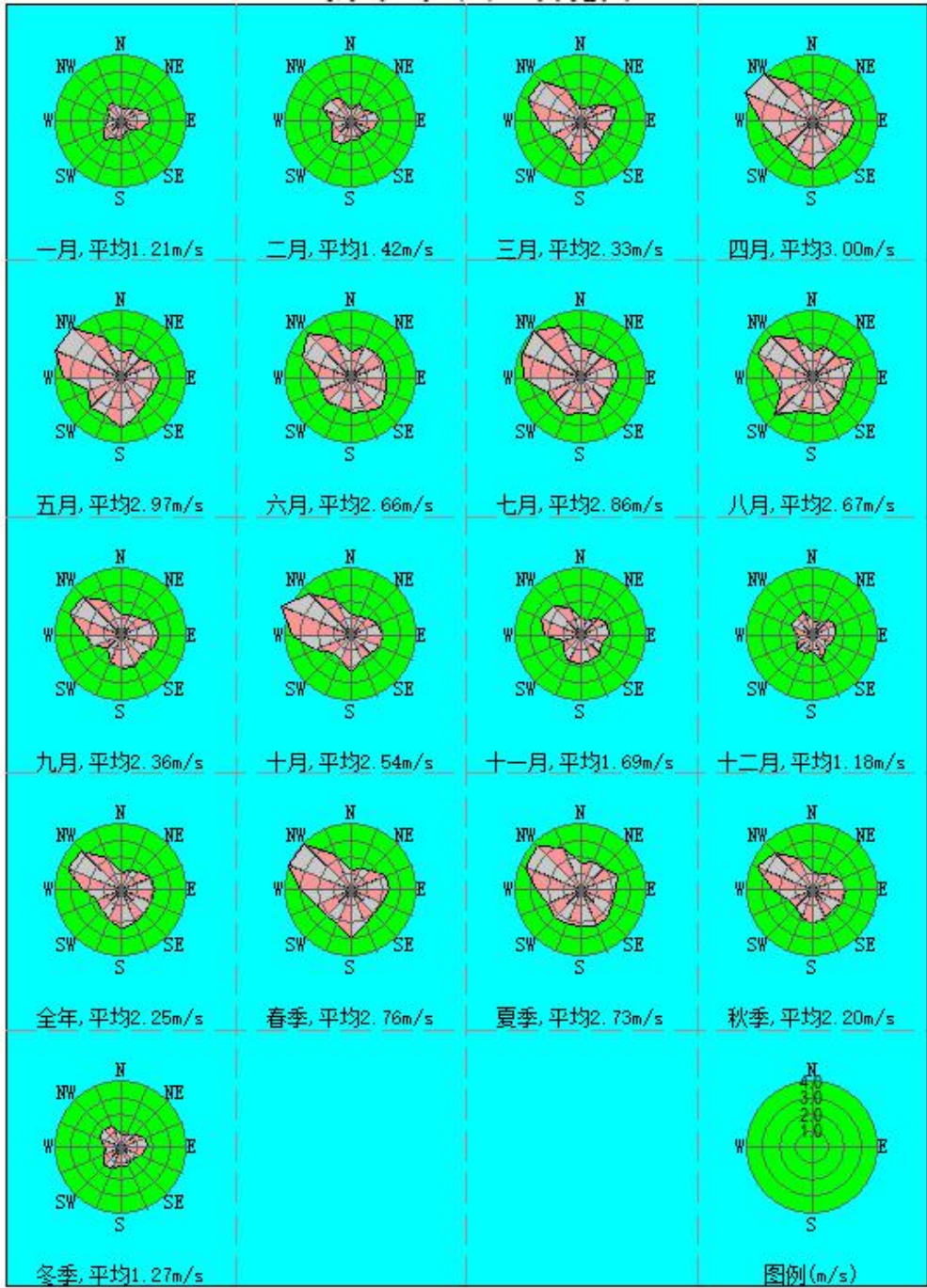
图 5.2-4 2018 年克拉玛依风速玫瑰图
