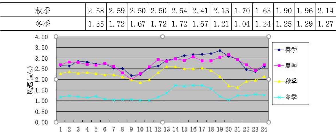
图 5.2-3 季小时风速的月变化图
