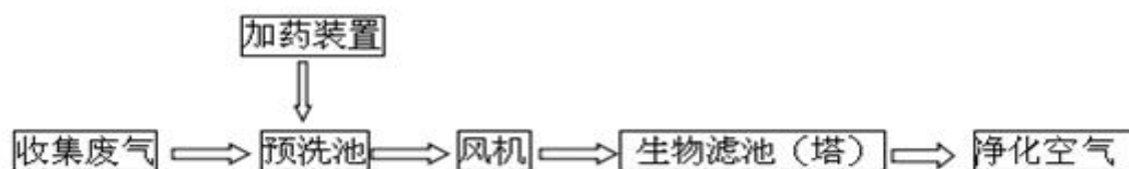
图 3.2-2 离子除臭法工艺流程图
