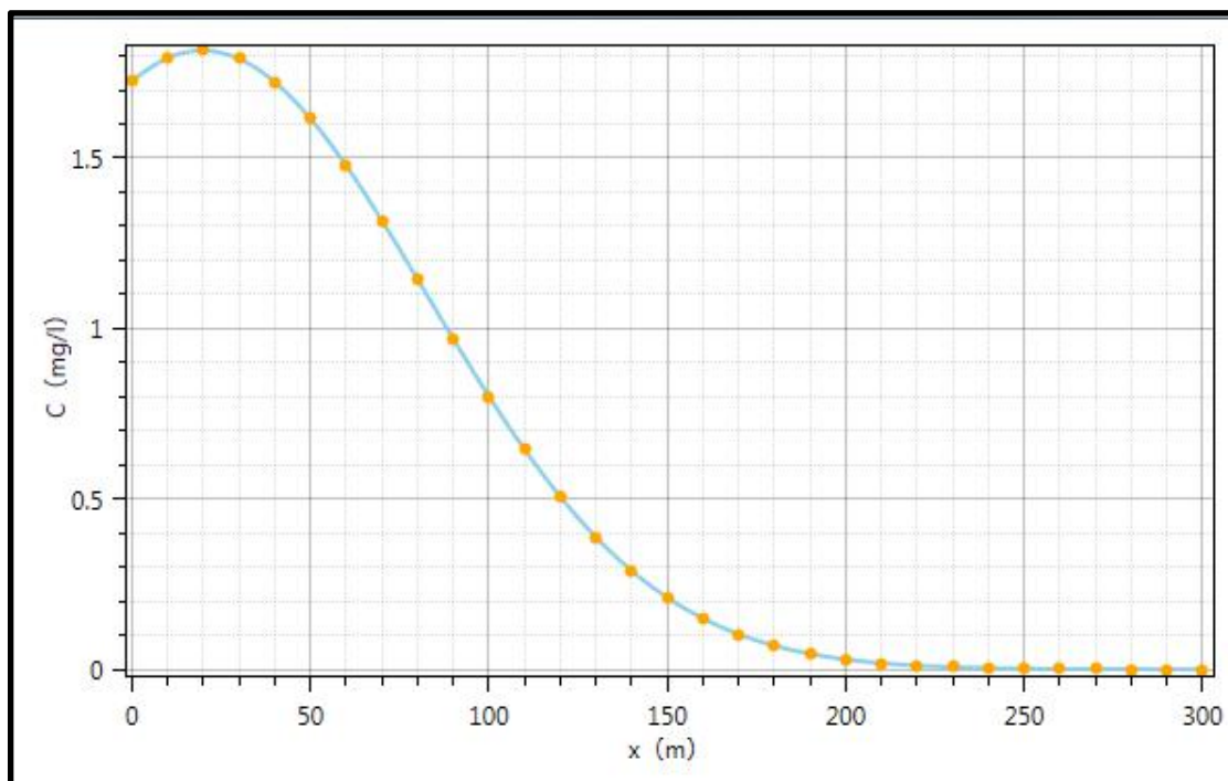
图 6.2-10 事故泄漏时 氨氮 365d 后浓度变化趋势图
