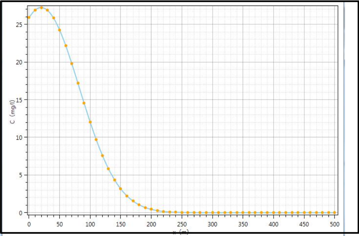
图 6.2-5 事故泄漏时 COD365d 后浓度变化趋势图
