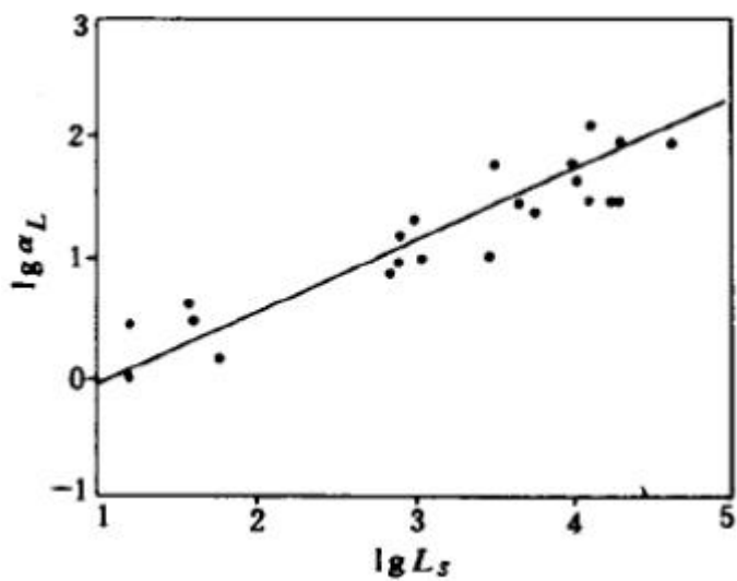
6.2-2 孔隙介质数值模型的 lg α L—lgLs
