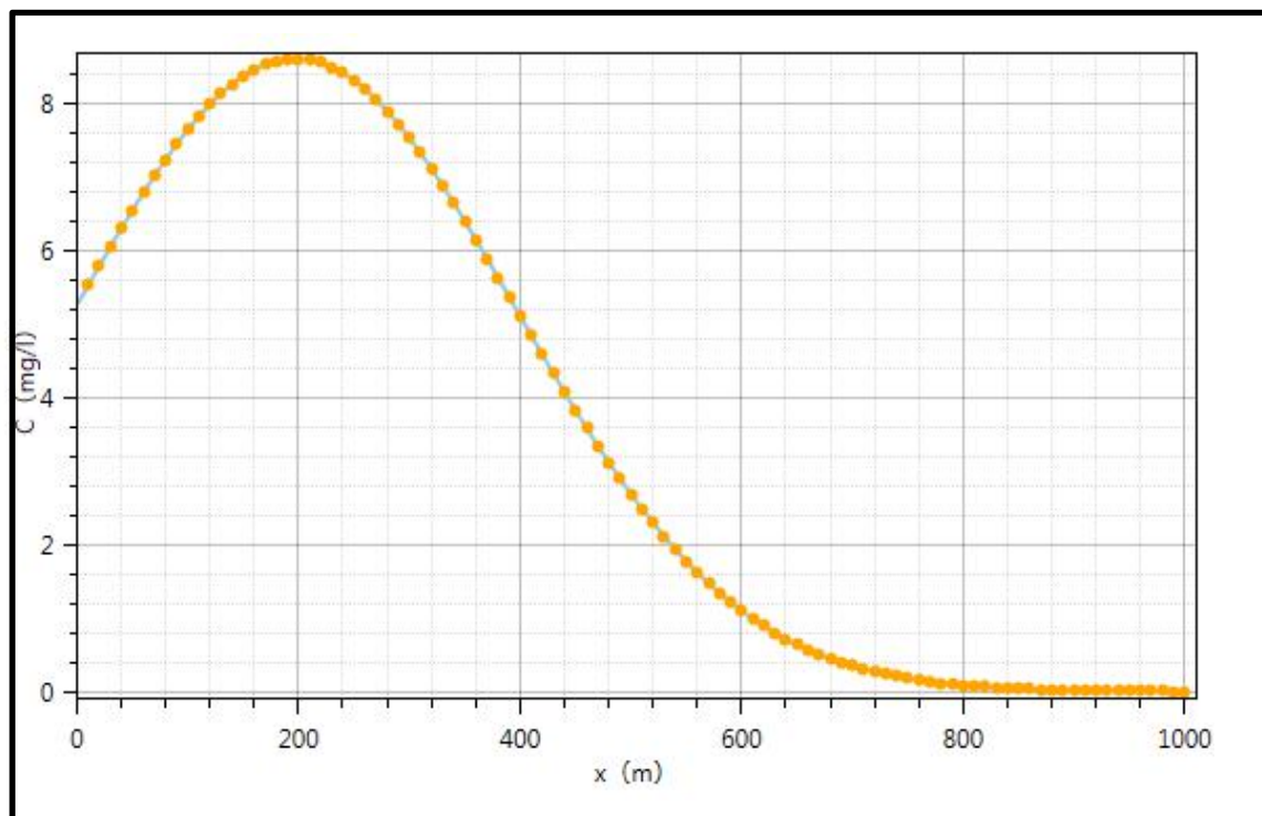
图 6.2-7 事故泄漏时 COD3650d 后浓度变化趋势图
