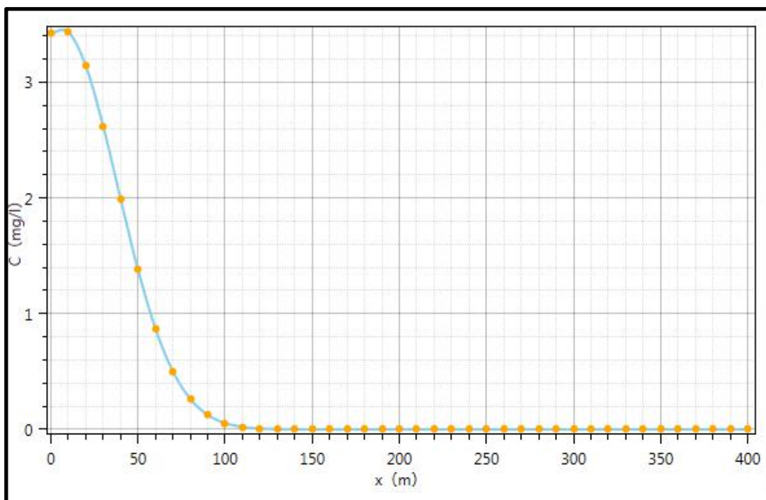
图 6.2-9 事故泄漏时 氨氮 100d 后浓度变化趋势图
