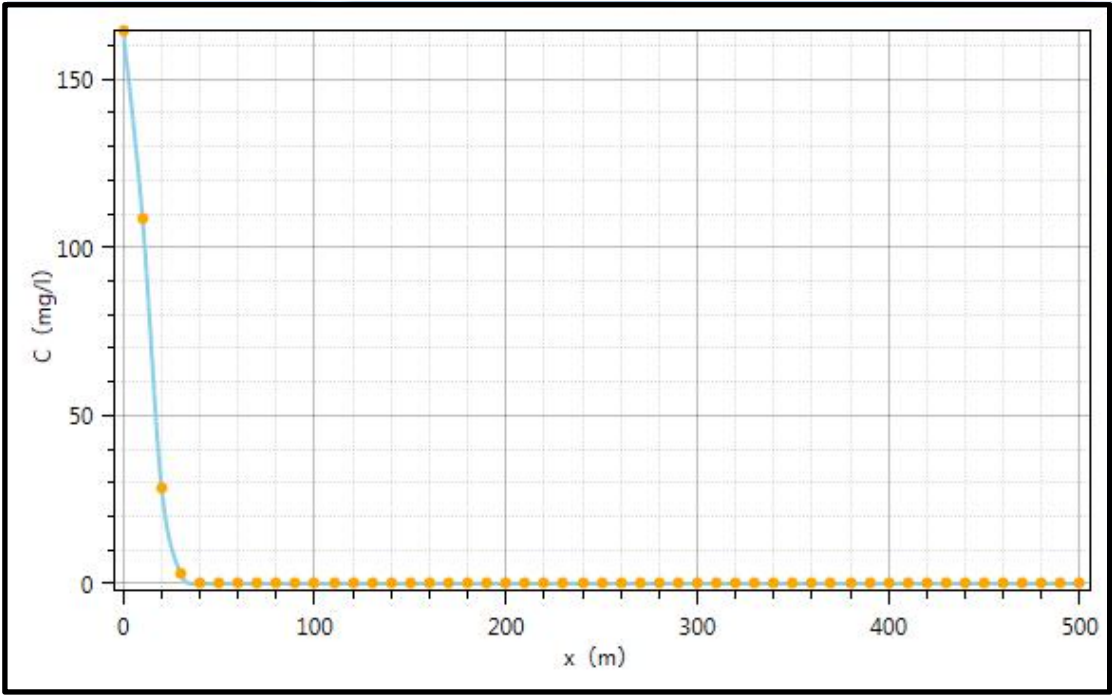
图 6.2-3 事故泄漏时 COD 30d 后浓度变化趋势图
