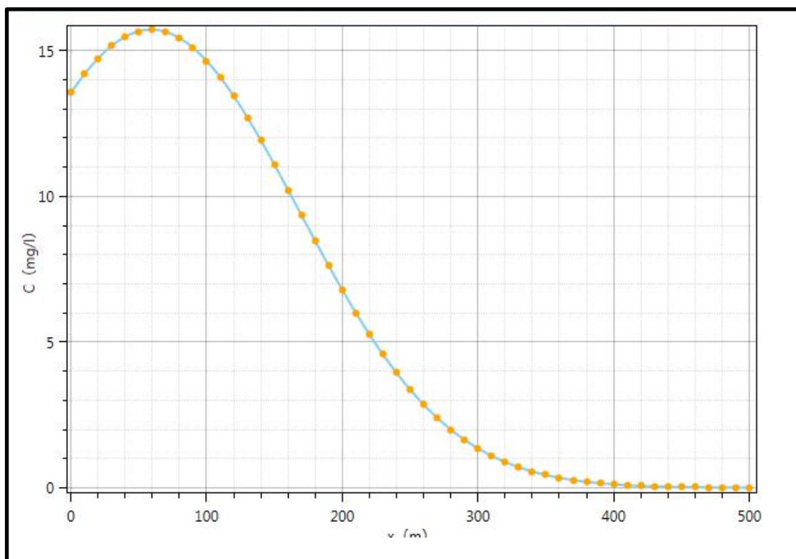
图 6.2-6 事故泄漏时 COD1095d 后浓度变化趋势图
