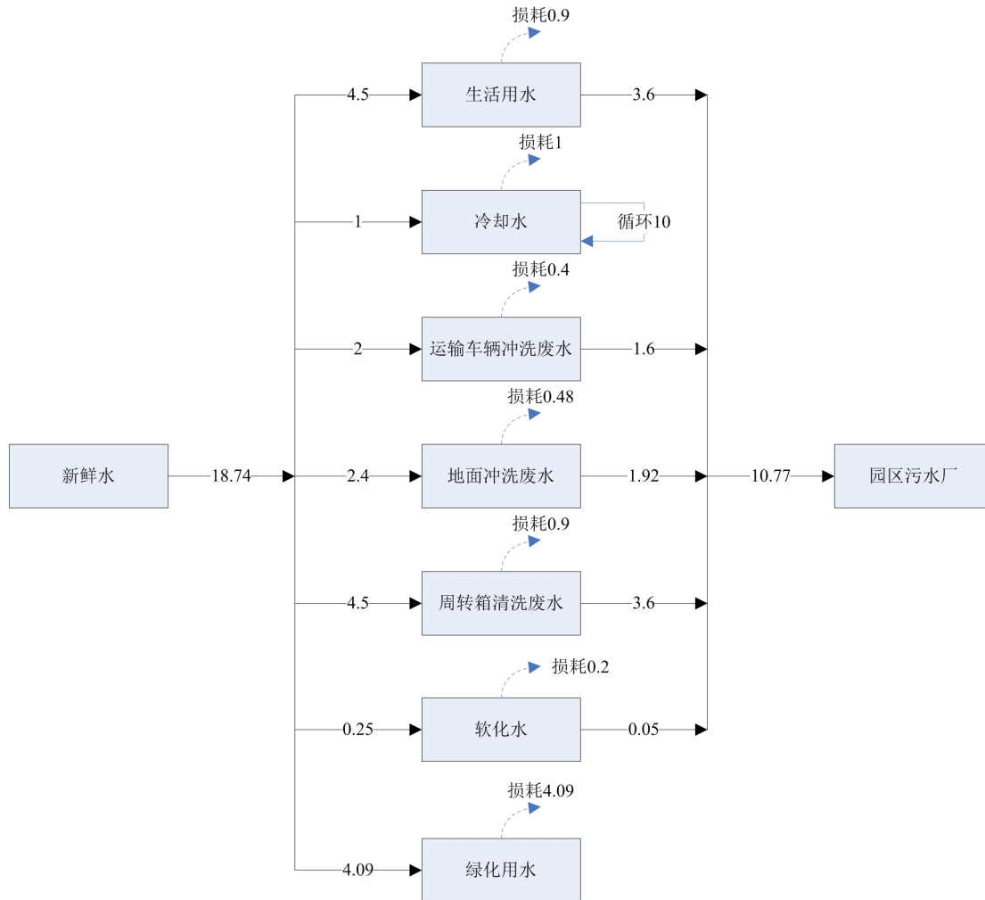
图 3.1-2 项目给排水平衡图 单位: m 3 /d
