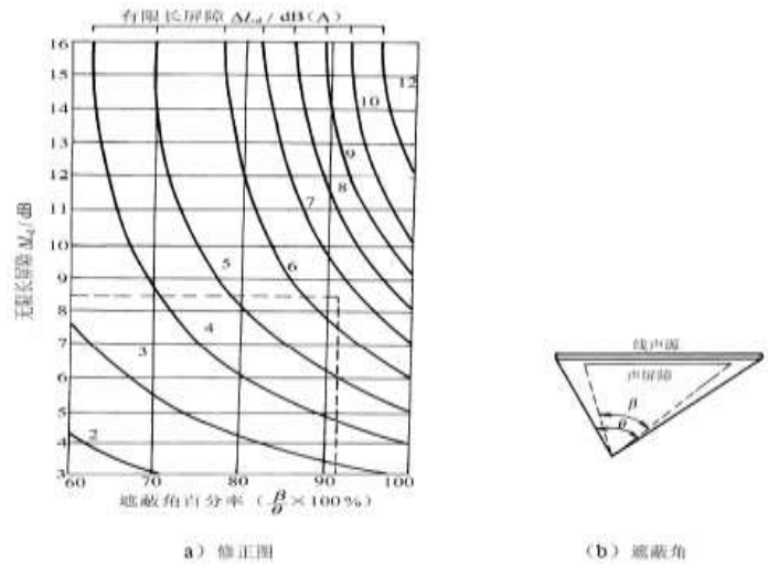
图 5.2-2 有限长声屏障及线声源的修正图
