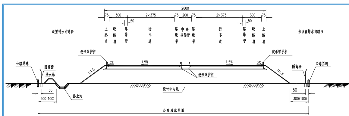
图 3.1-2 路基标准横断面图
