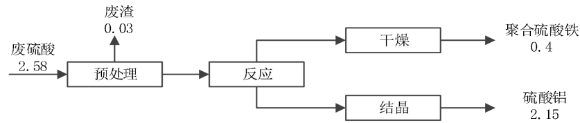
图 5.12-7 砷平衡一览表 单位：kg/a
