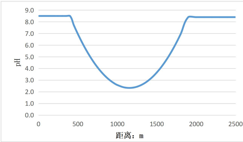
图 8.2-6 事故泄露后 7300dpH 污染锋面运移图
