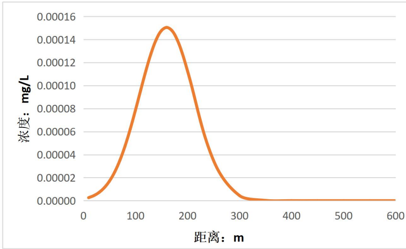
图 8.2-8 事故泄露后 1000d 汞污染锋面运移图
