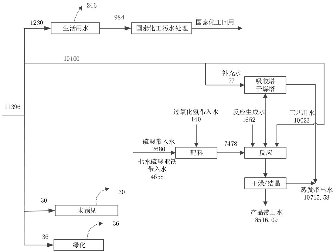
图 5.12-8 全厂水平衡表 单位：t/a
