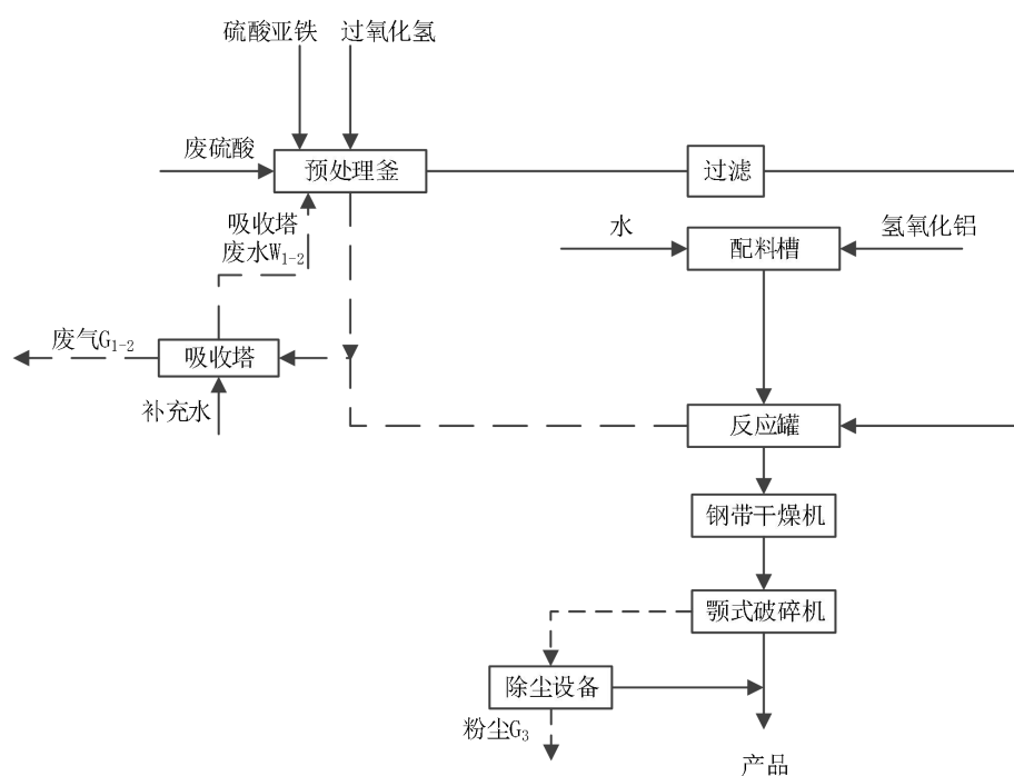
图 5.11.3 变更后新增硫酸铝主要生产流程及产污节点
