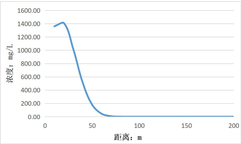
图 8.2-1 事故泄露后 100d 硫酸污染锋面运移图
