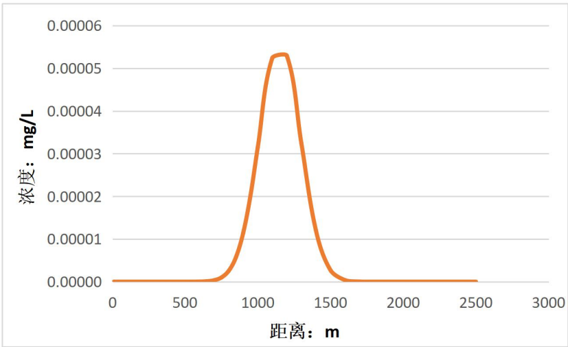
图 8.2-9 事故泄露后 7300d 汞污染锋面运移图
