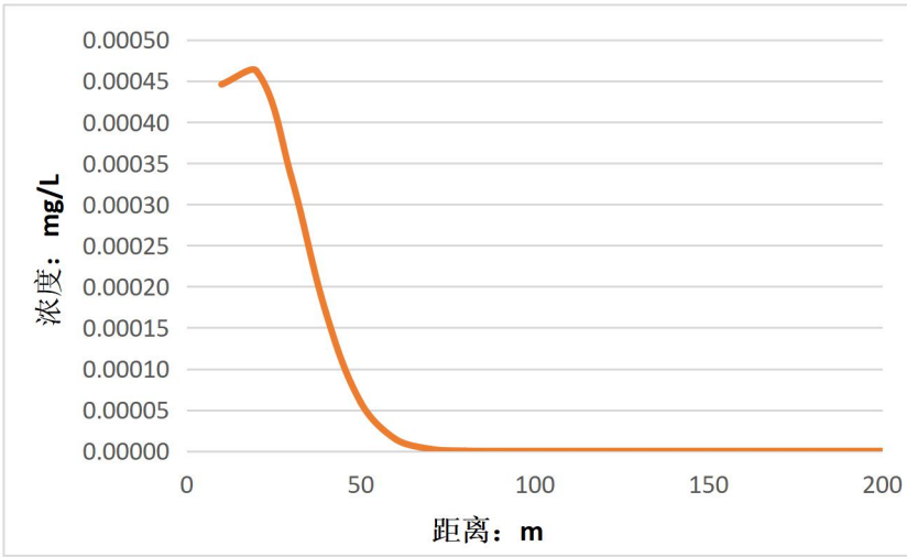
图 8.2-7 事故泄露后 100d 汞污染锋面运移图
