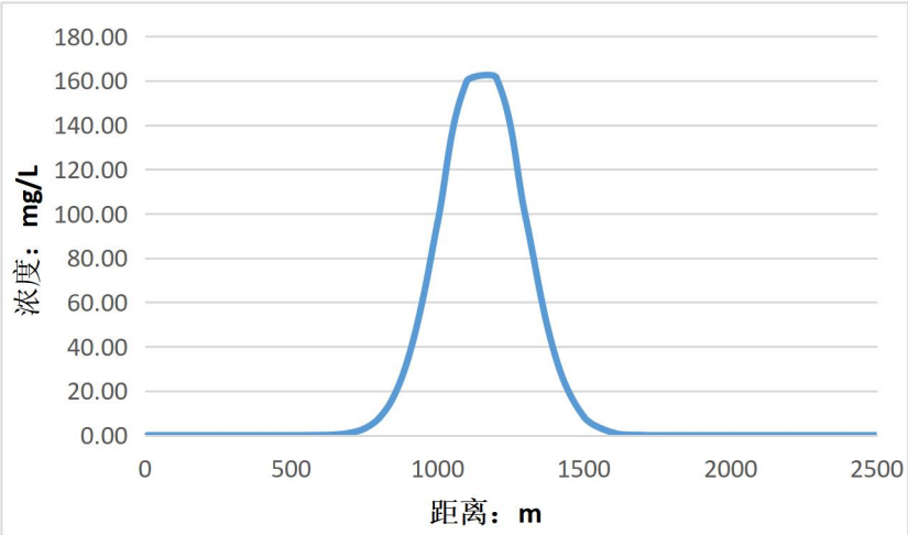
图 8.2-5 事故泄露后 7300d 硫酸污染锋面运移图
