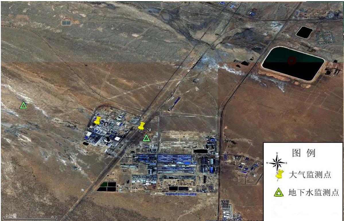
图 6.3-1 环境空气及地下水环境监测布点图
