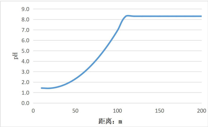
图 8.2-2 事故泄露后 100dpH 污染锋面运移图
