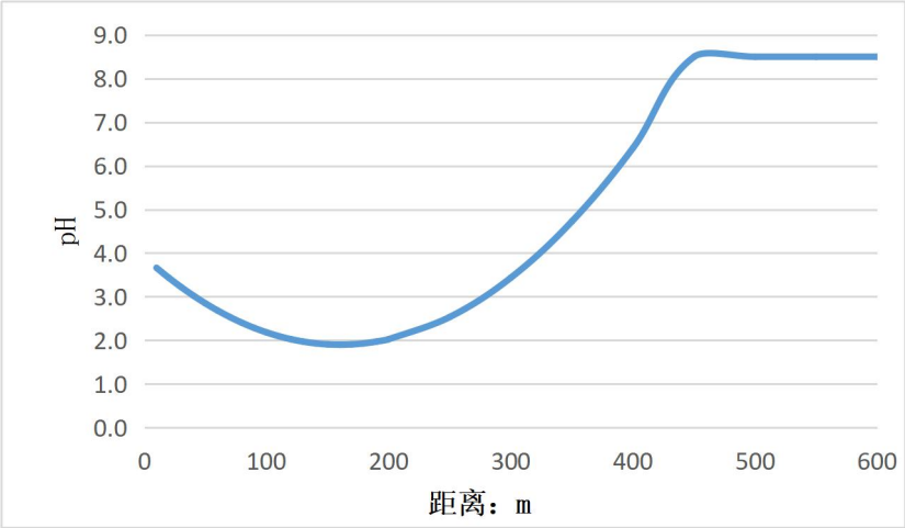
图 8.2-4 事故泄露后 1000d pH 污染锋面运移图
