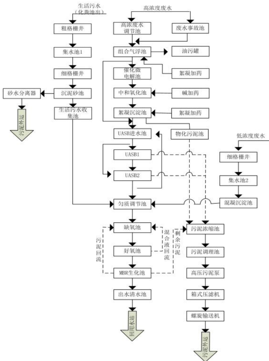
图 5.5-1 国泰化工一期项目污水处理工艺流程图
