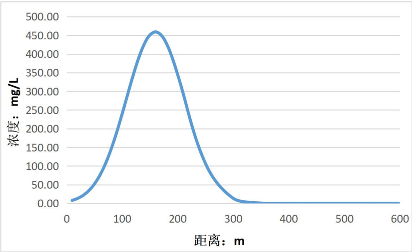
图 8.2-3 事故泄露后 1000d 硫酸污染锋面运移图
