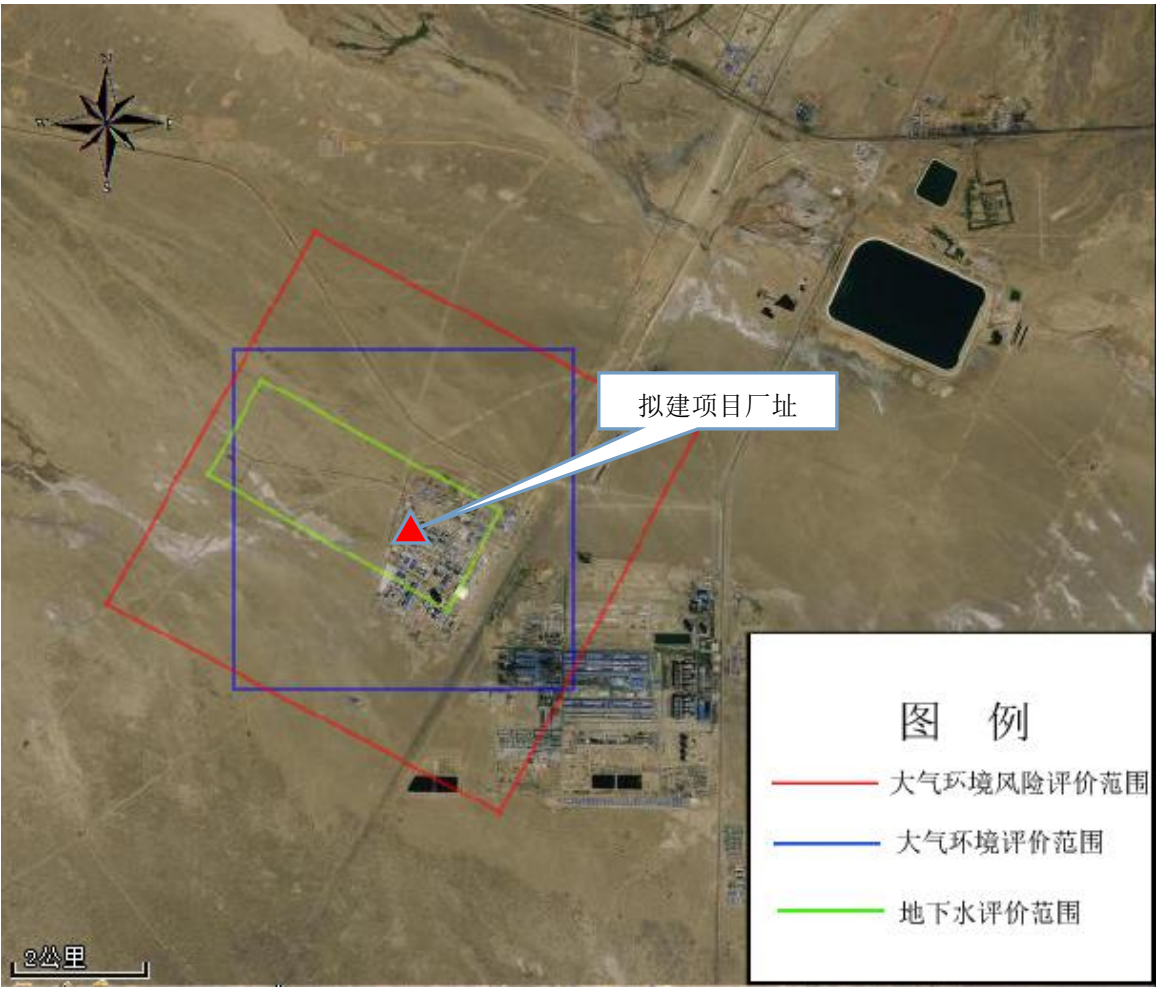
图 2.4-1 项目评价范围图
