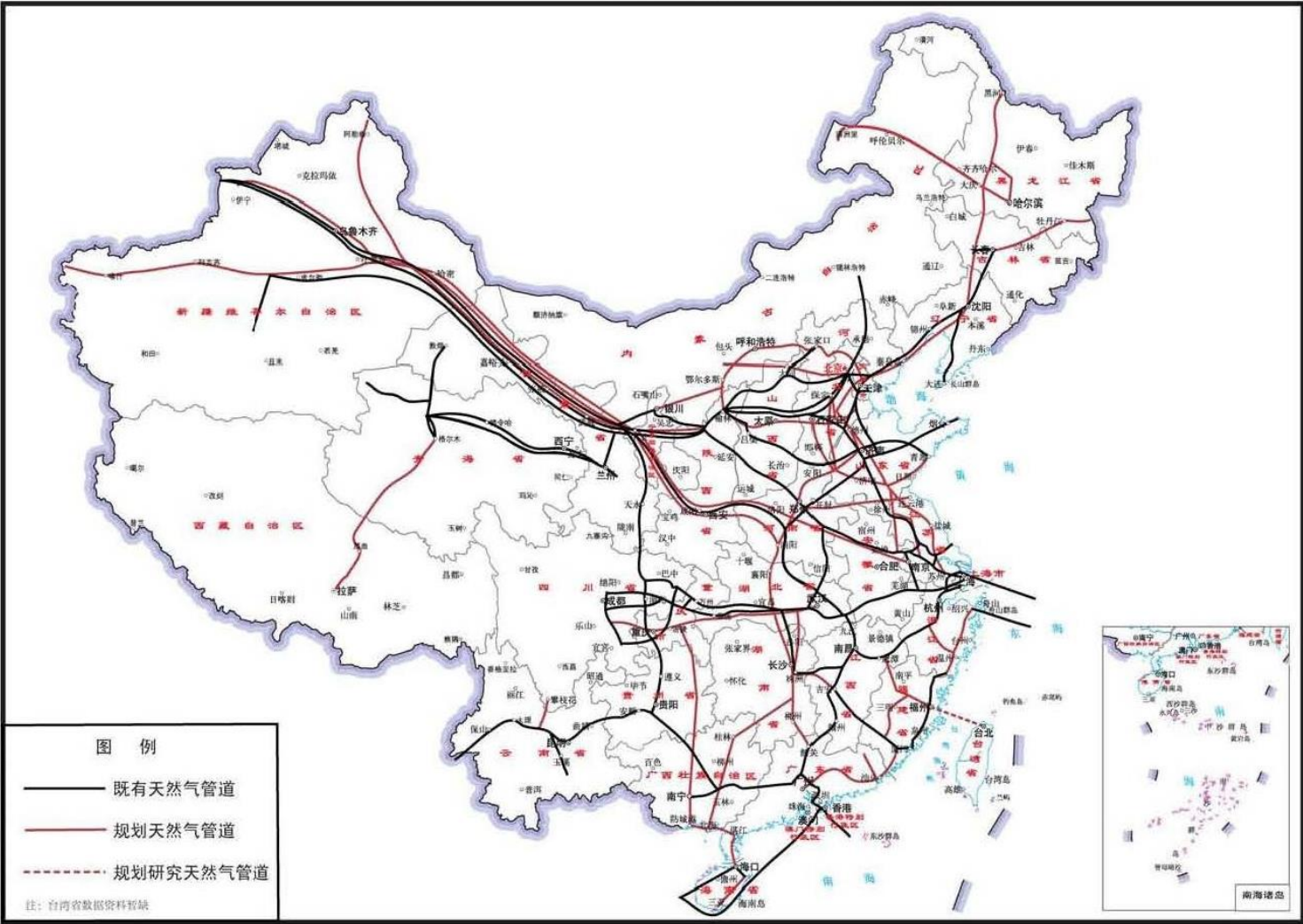
图 2.2-4 中长期天然气干线管道布局图
