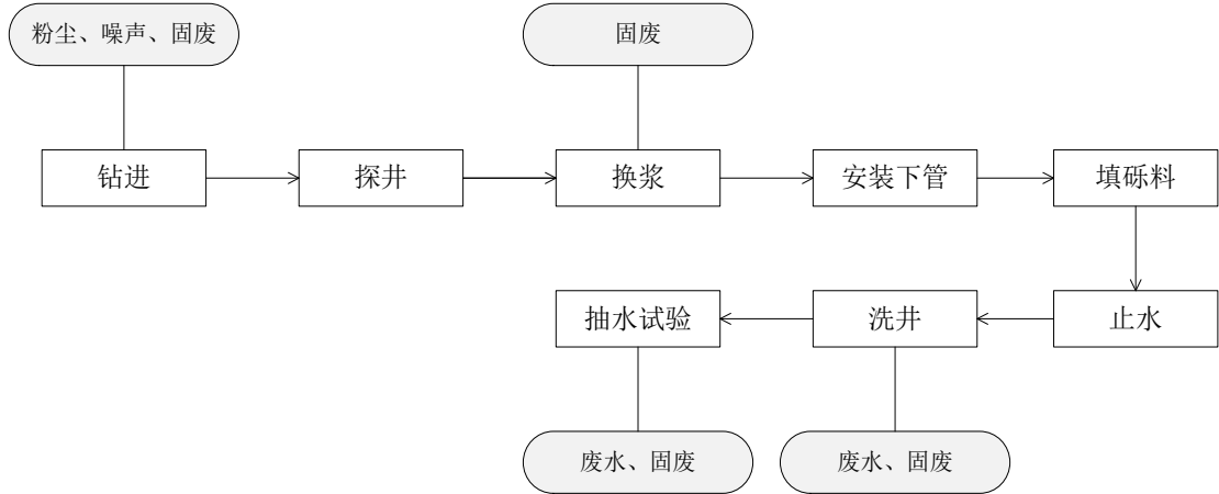
图 3.3-1 水源井成井工艺及排污节点图
