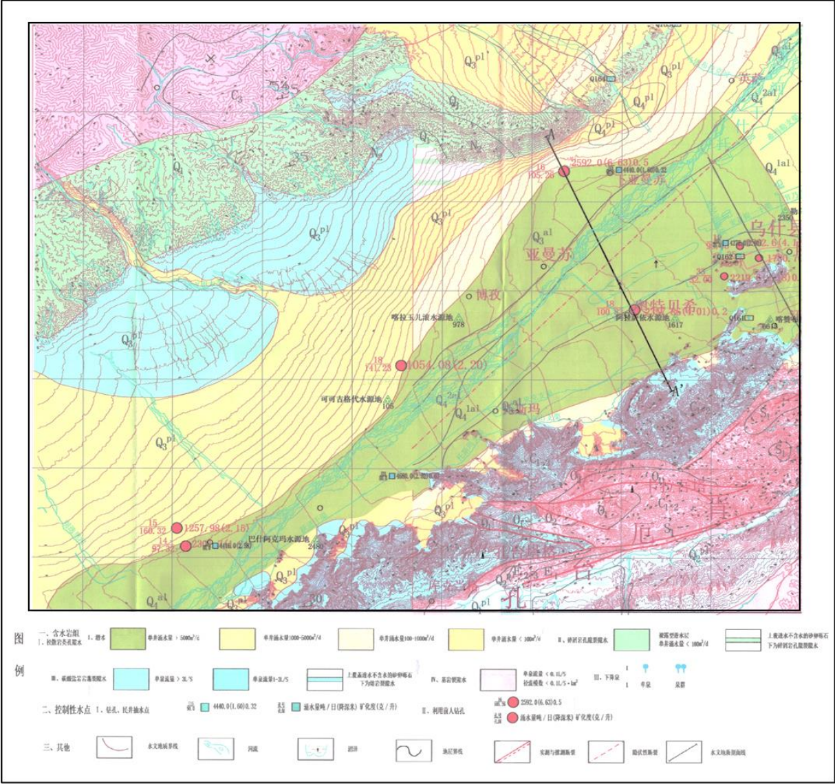
图5.2-1 区域水文地质图
