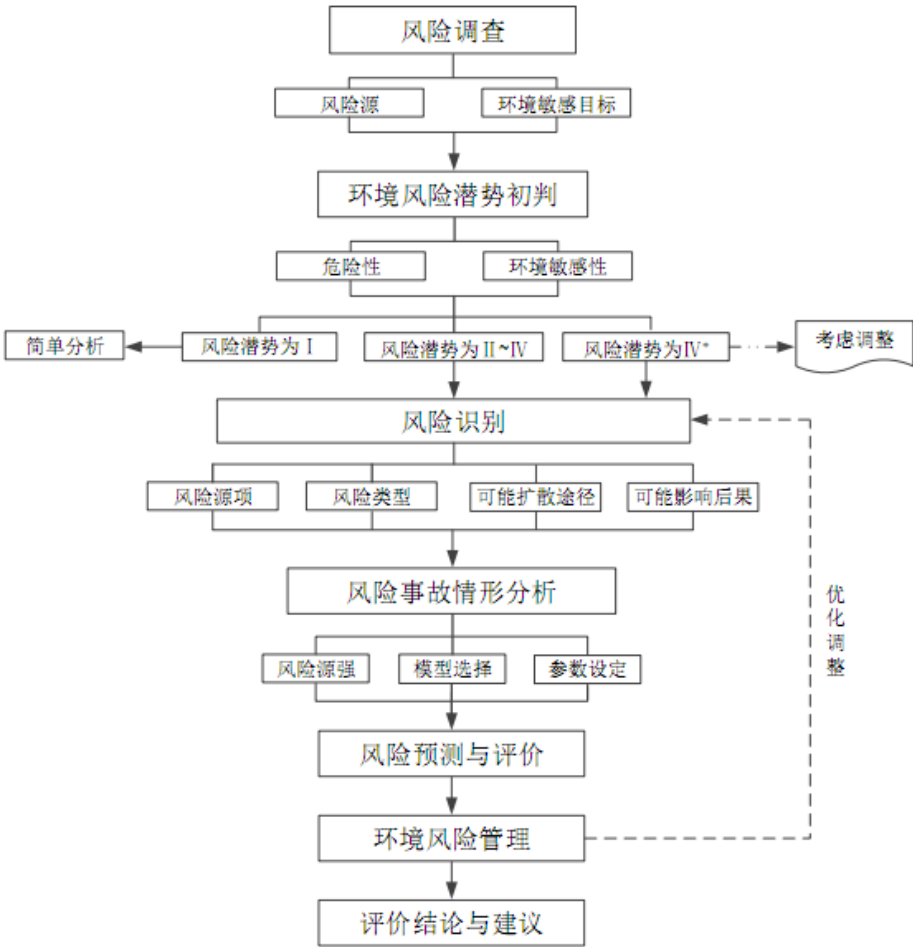
图 5.3-1 环境风险评价流程框图
