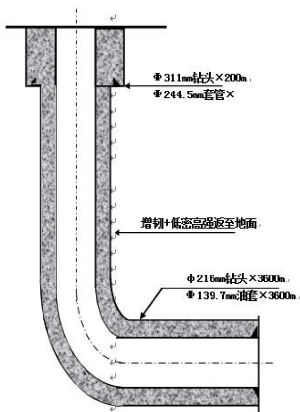
图 3.2-3 马 1 块芦草沟水平井井身结构示意图
