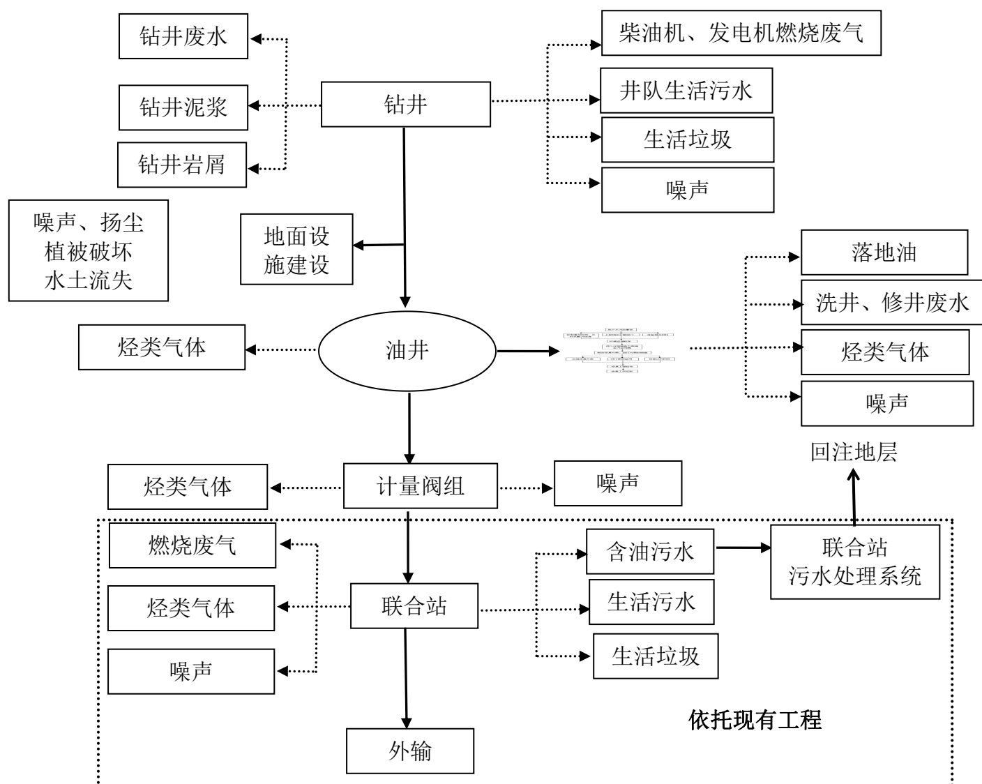
图 3.3-1 工艺流程及产污节点图
