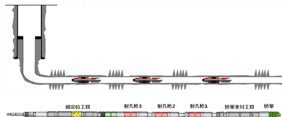
图 3.2-4 水平井桥塞压裂工艺图
