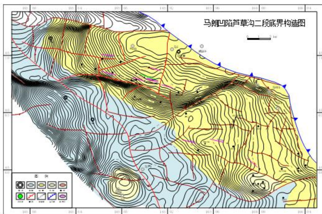
图 3.2-1 马朗凹陷芦草沟二段底界构造图
