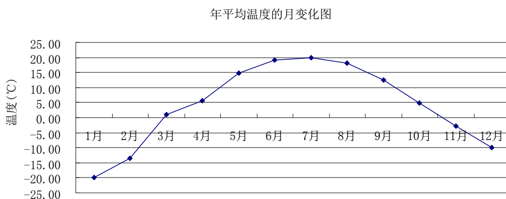
图 5.1-4 巴里坤哈萨克自治县 2018 年年平均温度的月变化曲线
