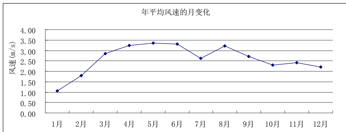
图 5.1-2 巴里坤哈萨克自治县 2018 年年平均风速的月变化曲线
