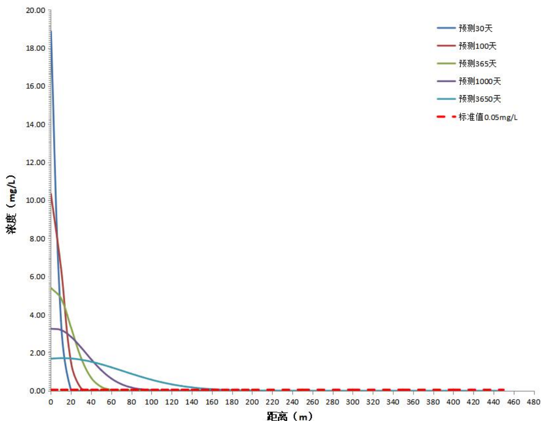
图 5.3-1 石油类随时间沿地下水流方向污染预测结果图
