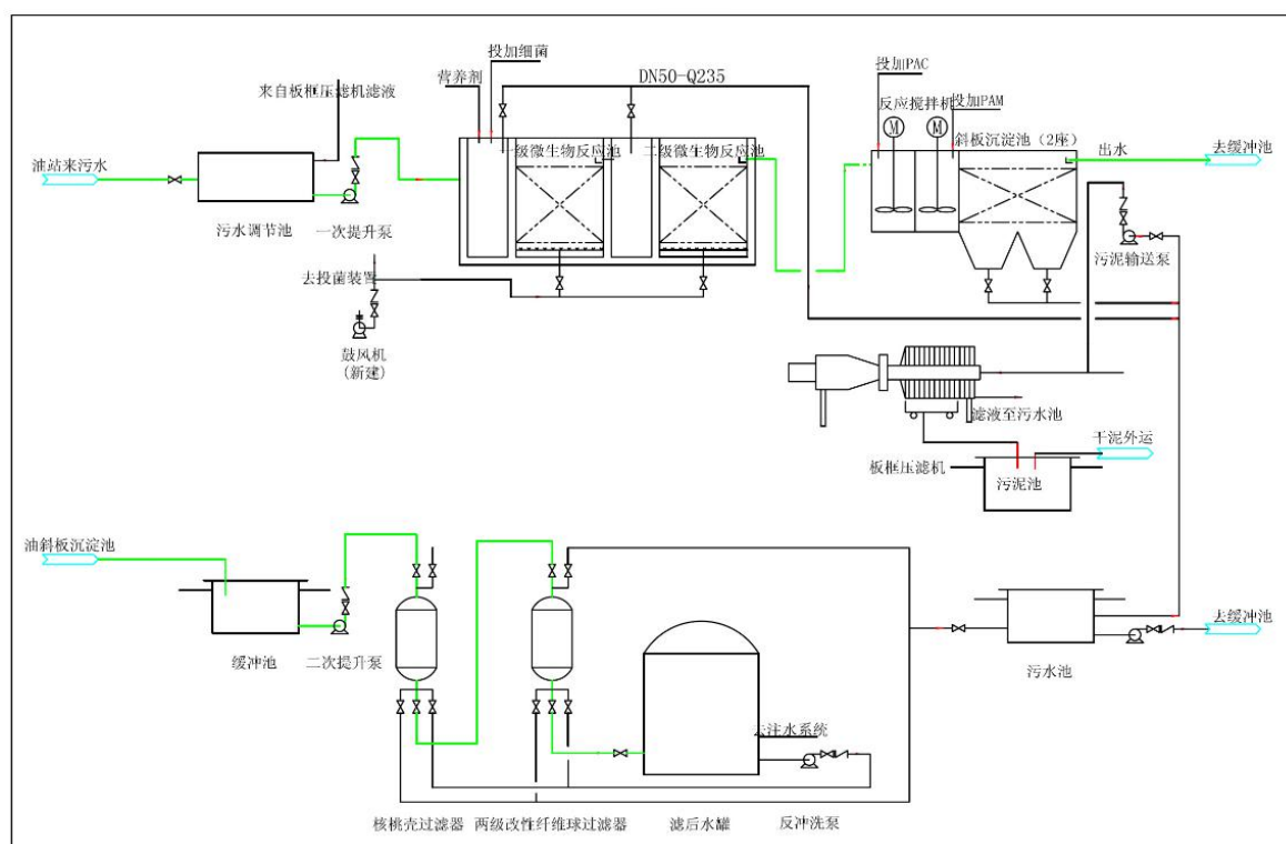
图 3.2-10 牛圈湖联合站污水处理工艺流程图
