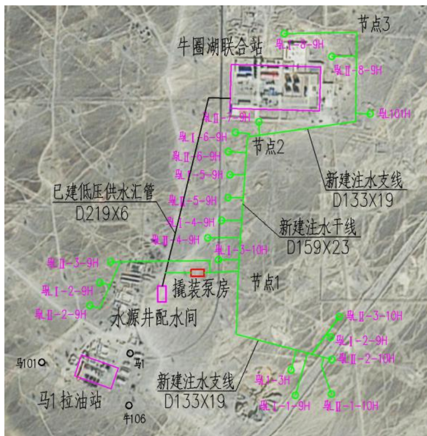
图 3.2-6 马1 芦草沟区块注水吞吐管线走向图
