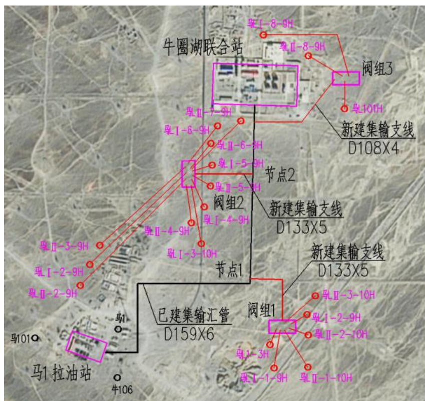
图 3.2-5 新建油气集输支线至马1井区集输汇管平面走向图
