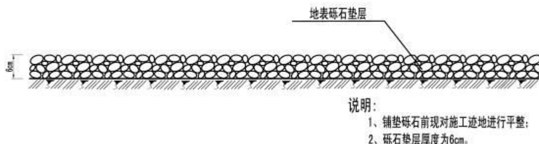
图 6.5-1 井场、阀组区砾石压盖措施典型设计图
