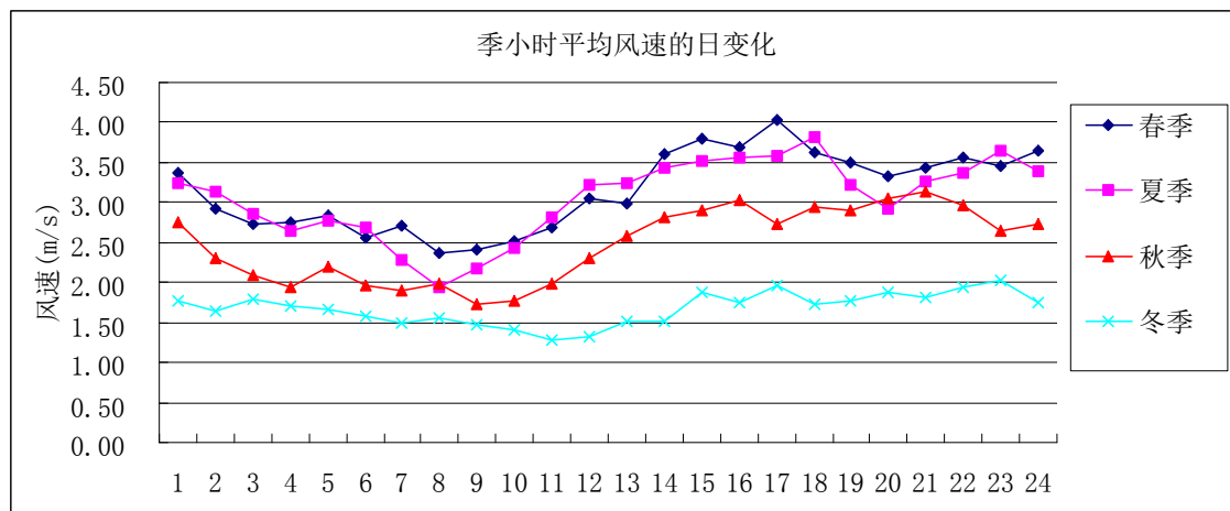
图 5.1-3 巴里坤哈萨克自治县 2018 年各季小时风速的日变化曲线
