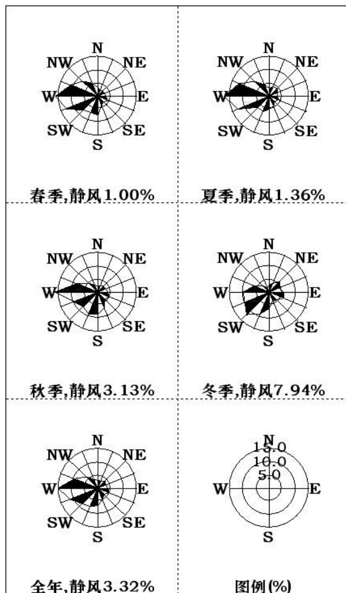
图 5.1-1 巴里坤哈萨克自治县 2018 年全年及各季风向玫瑰图
