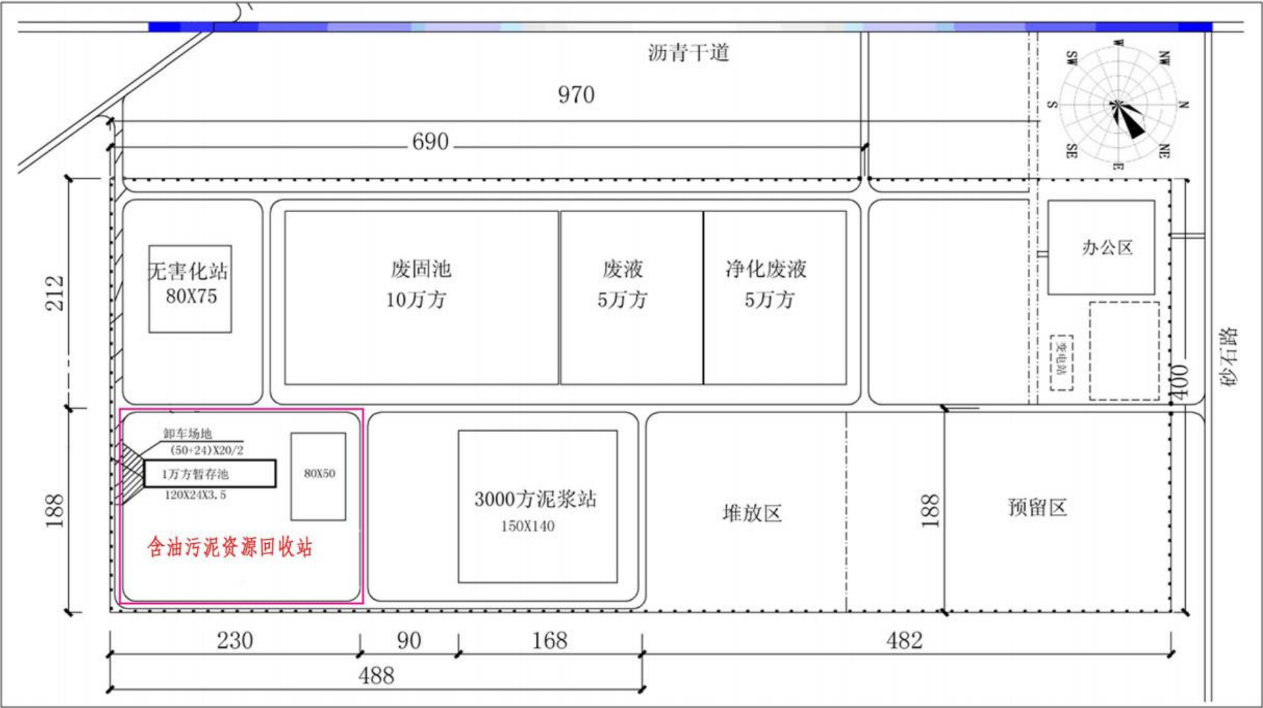
图 3.1-2 塔中环保站总平面布置图
