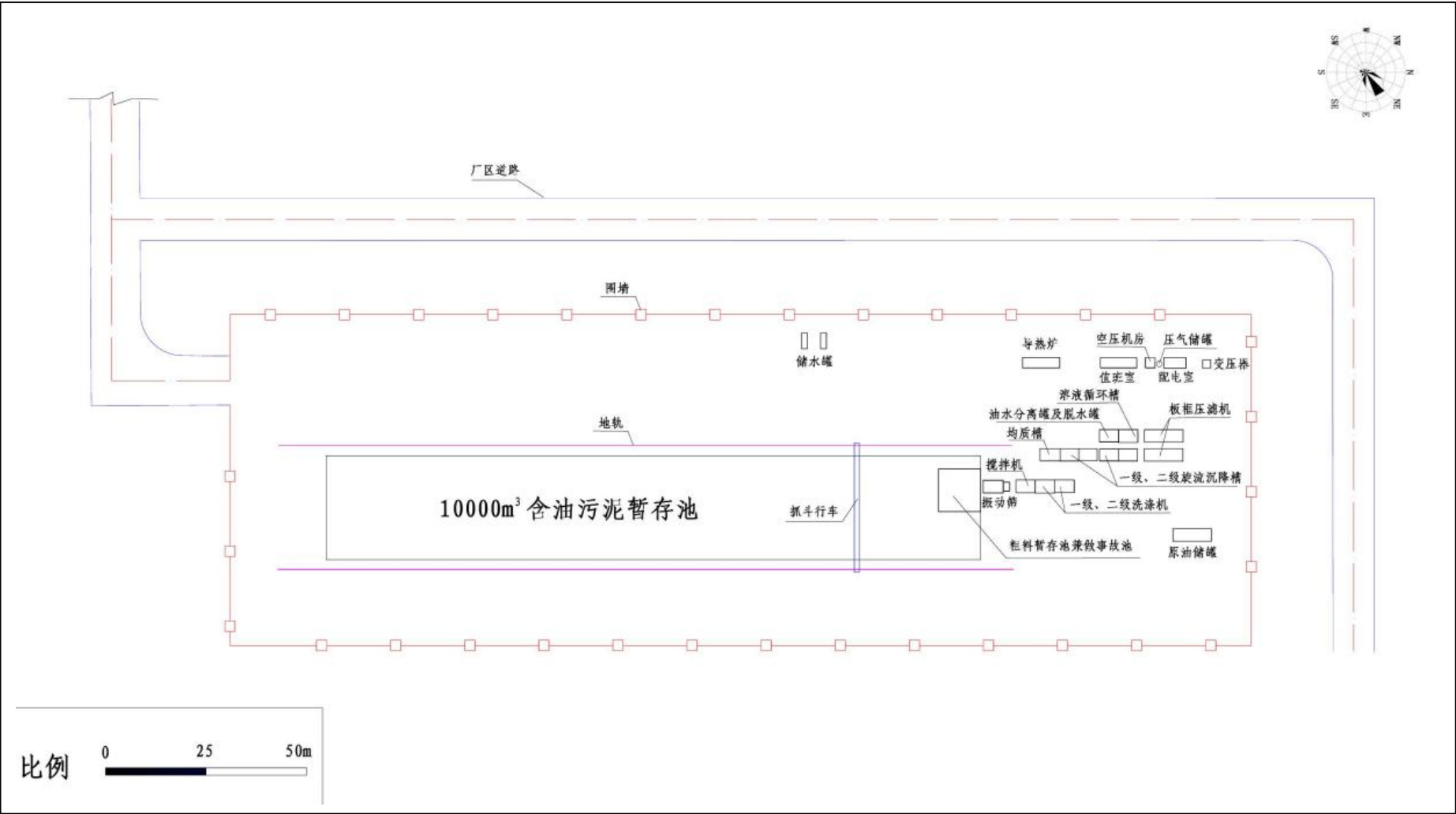
图 3.1-3 现有工程总平面布置图
