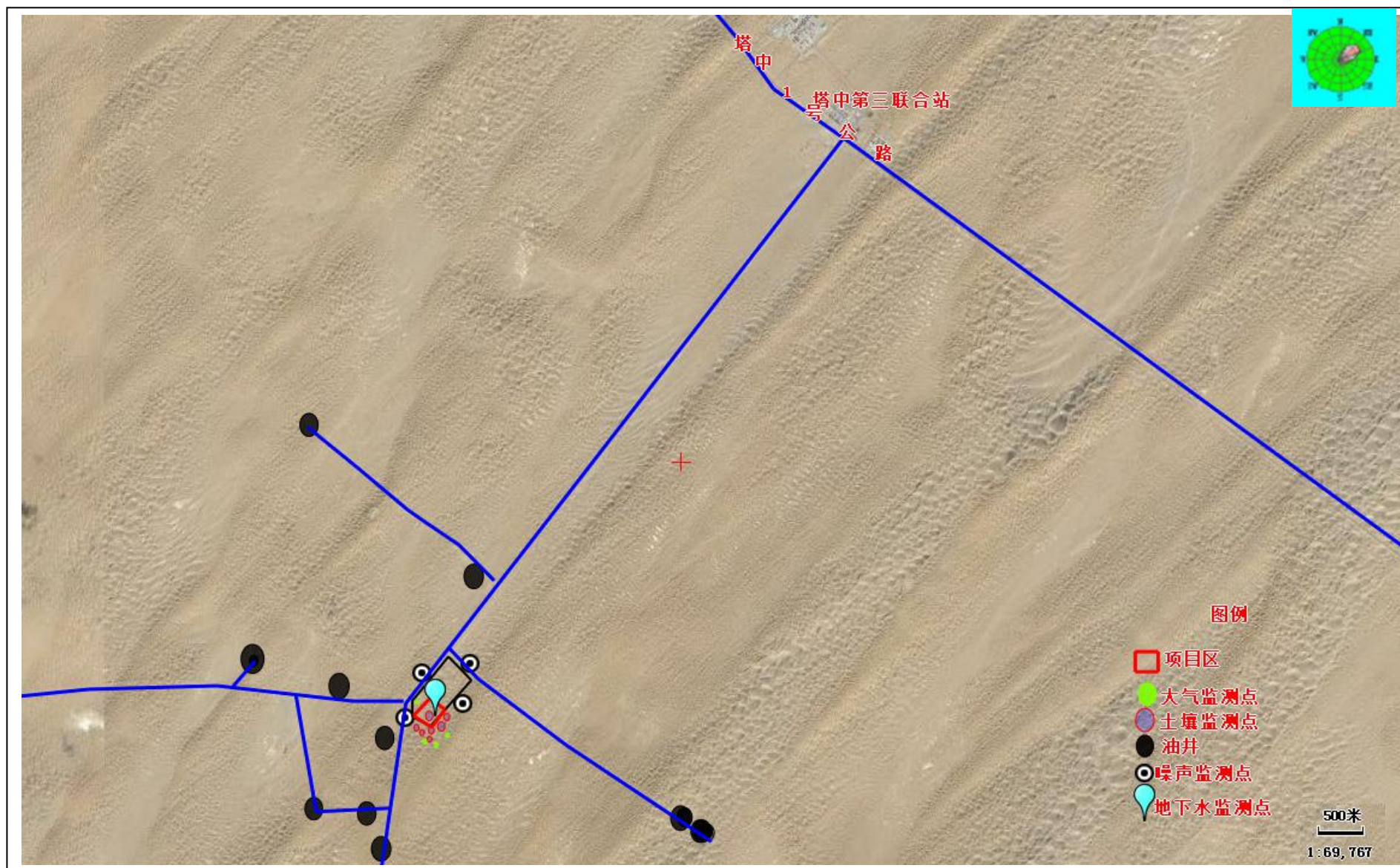
图 4.3-1 项目监测布点示意图
