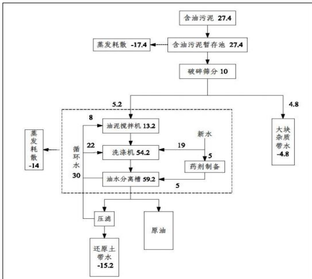
图 3.4-4 现有工程水量平衡图 单位： \text{m}^3/\text{d}
