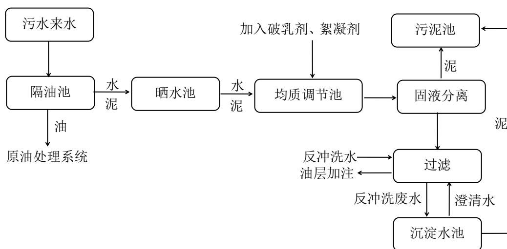
图 3.4-1 塔中环保站综合废水处理系统水处工艺流程图
