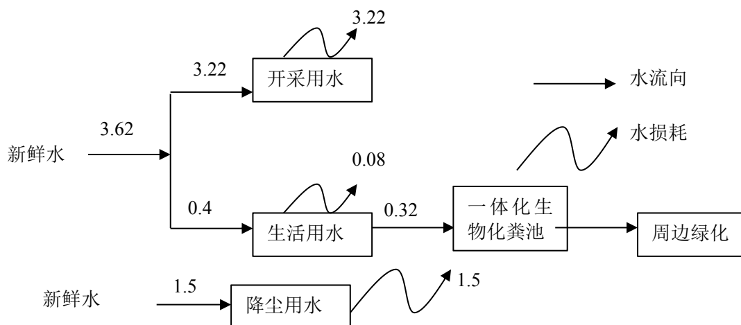
图 3.2-1 项目用排水平衡图 (m³/d)
