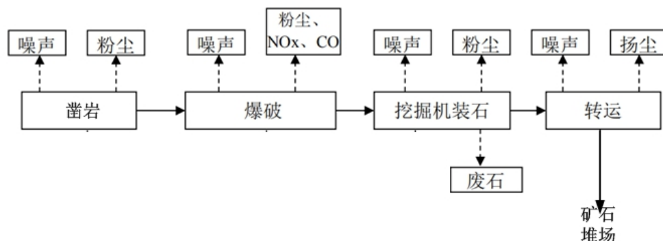
图 3.2-2 采矿工艺流程及产污节点图
