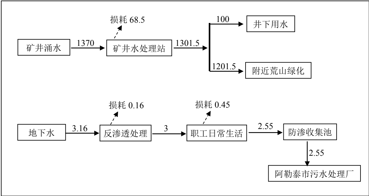
图 3.2-1 生产季节水平衡图 单位：m³/d
