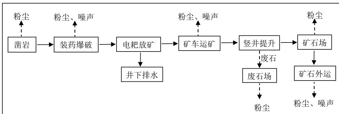
图 3.4-1 生产工艺流程及排污节点示意图
