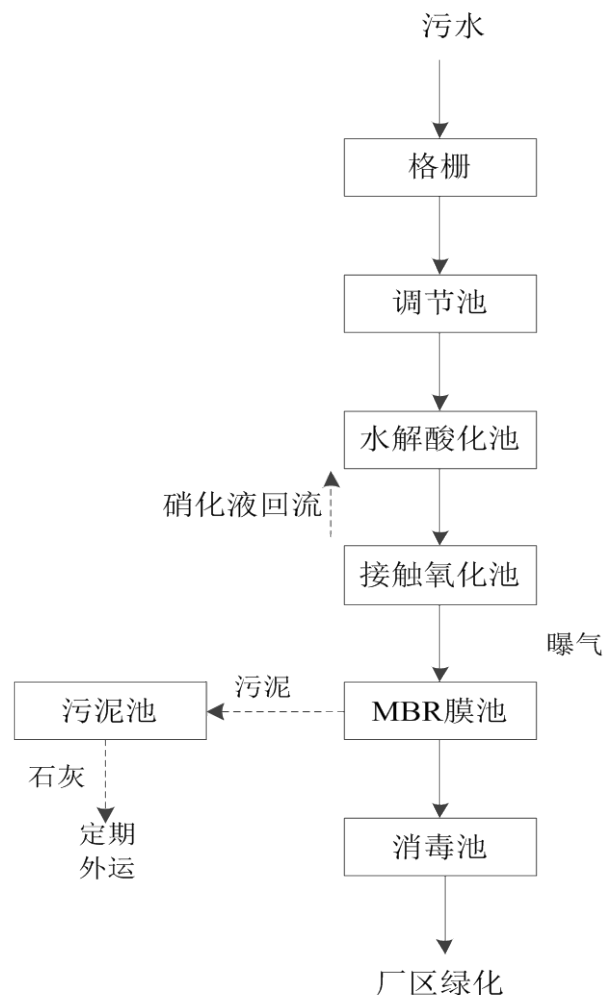
图 6.2-1 项目污水处理设施工艺流程图
