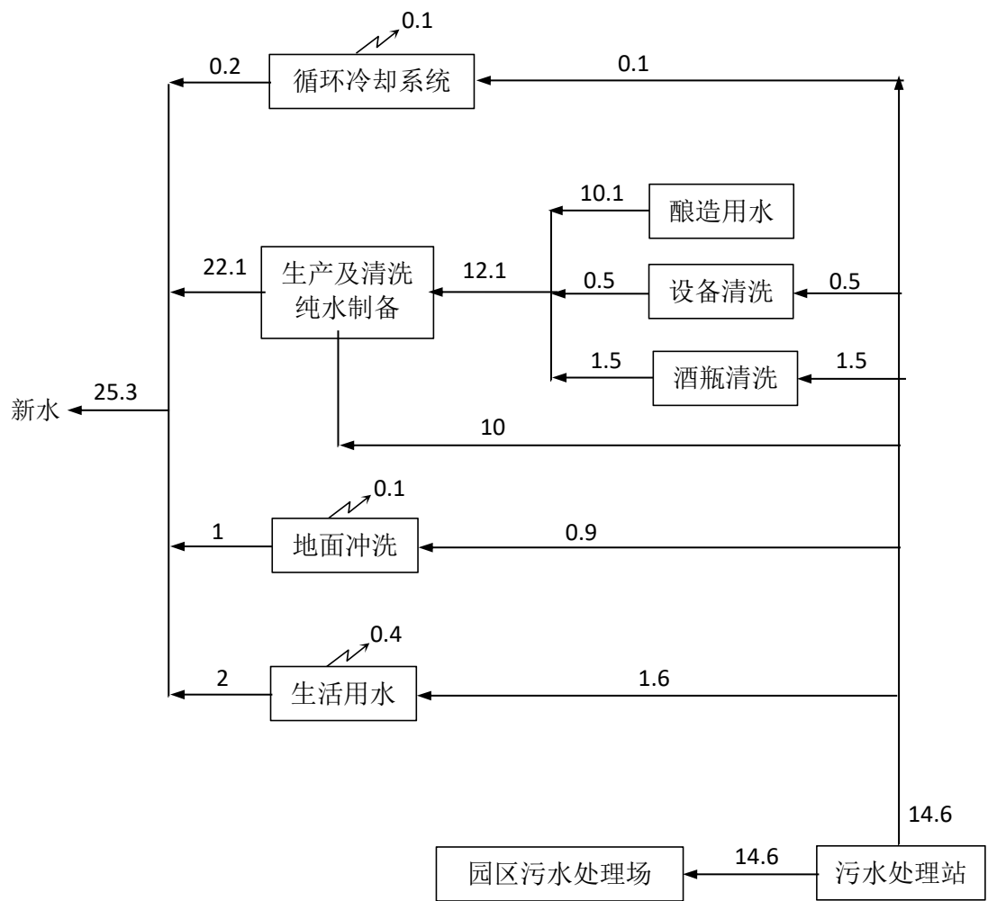
图 2-5 拟建项目水平衡图 m³/d
