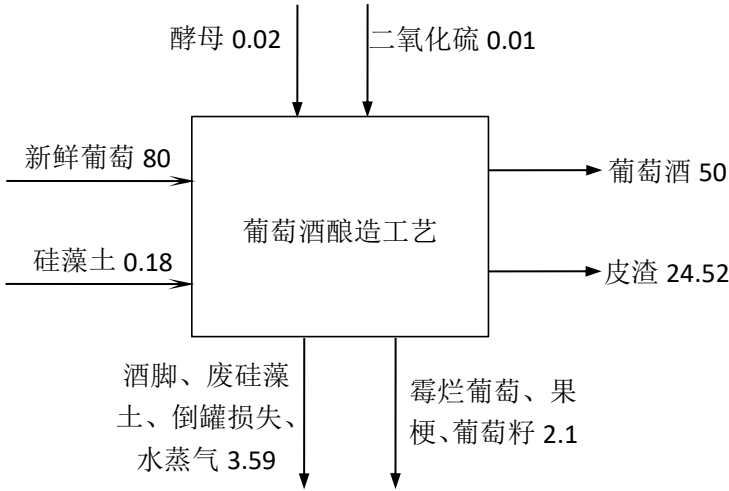
图 2-4 拟建项目葡萄酒物料平衡图
