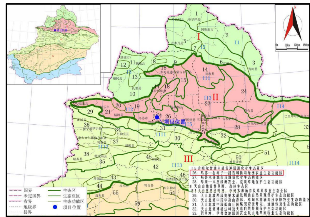
图 3-4 生态功能区划图
