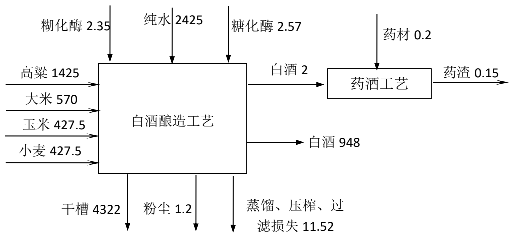
图 2-3 拟建项目白酒、药酒物料平衡图
