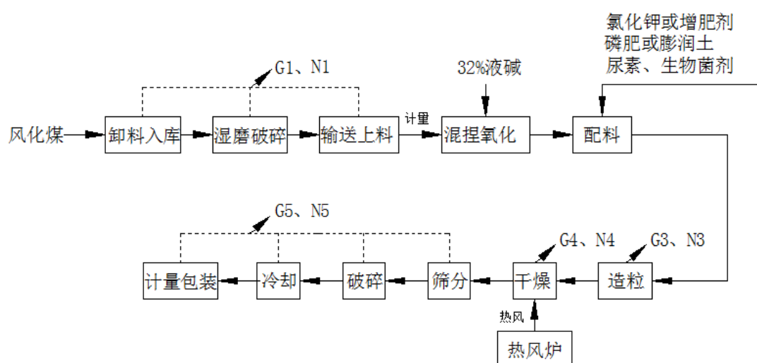
图 3.2-2 本项目腐植酸复混肥生产工艺及产污节点图
