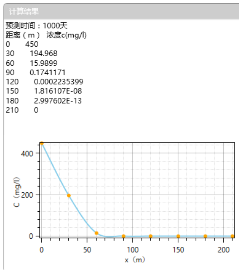
图 5.2-3 COD 持续泄露 1000d 随时间和位置变化的迁移结果
