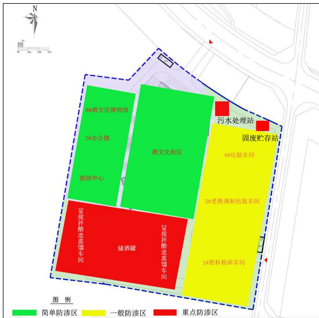
图 5.2-1 项目区分区防渗图
