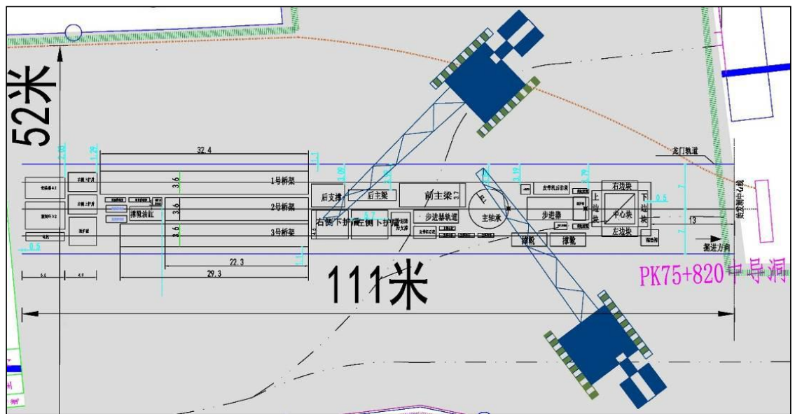
图 2.4-7 TBM 盾构拼装布置图
