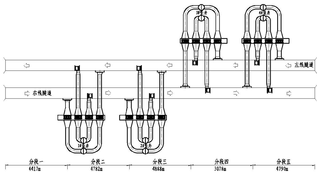
图 2.5.2-7 四竖井分五段纵向通风方案示意图
