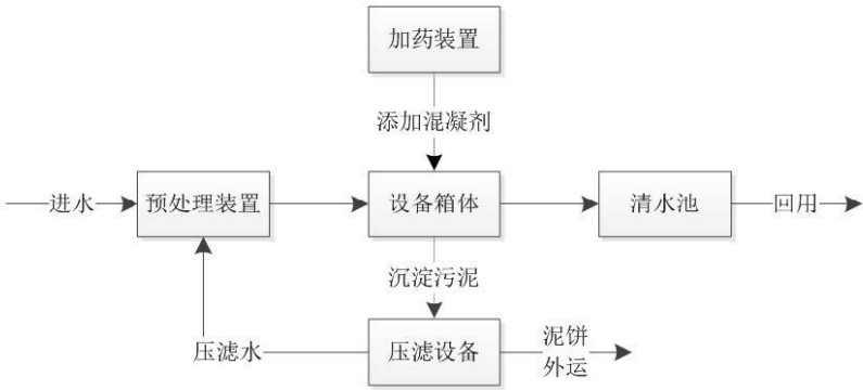
图2.5.5-3 一体化处理设备工艺流程图
