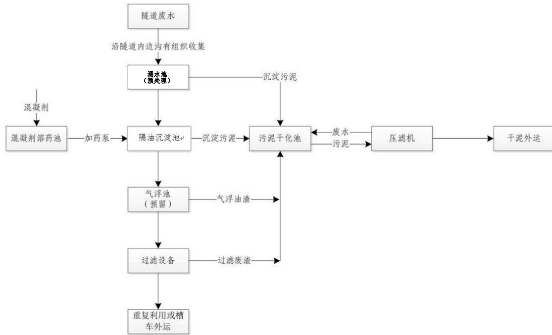
图6.2-6 隧道施工废水处理方案工艺流程图
