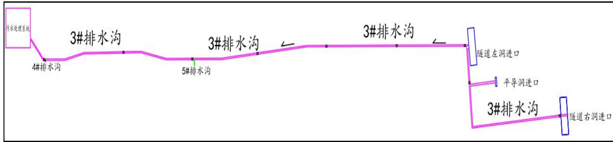
图6.2-4 隧道外施工废水导流典型设计图
