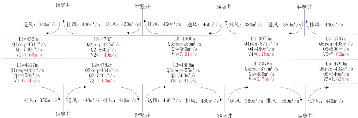
图 2.5.2-9 远期风量布置示意图
