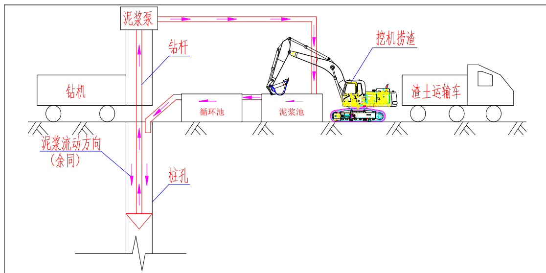
图 6.2-8 泥浆循环系统示意图
