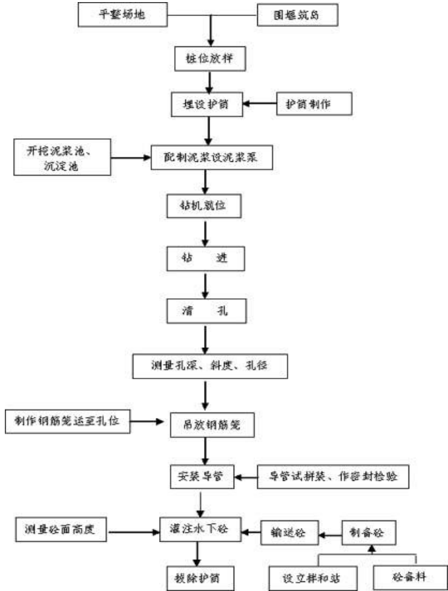
图 2.3.10-1 钻孔灌注桩基础施工工艺流程
