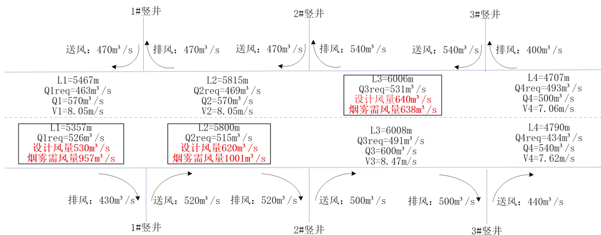
图 2.5.2-3 远期风量布置示意图
