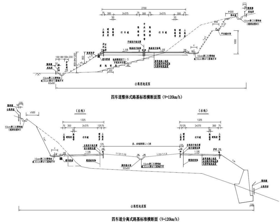
图 2.3-1a 拟建公路 26m 宽路基横断面图
