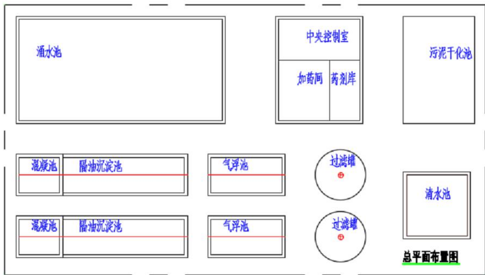
图 6.2-5 隧道施工废水处理设施布局示意图
