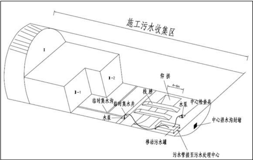
图 2.5.5-5 隧道施工废水收集、处理示意图
