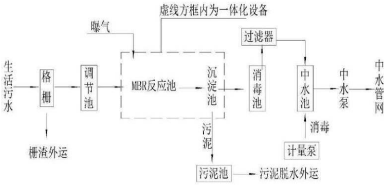
图2.5.5-4 膜生物反应器MBR 法处理工艺流程图
