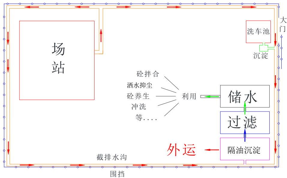
图 6.2-1 施工场地生产废水处理设施布局示意图
