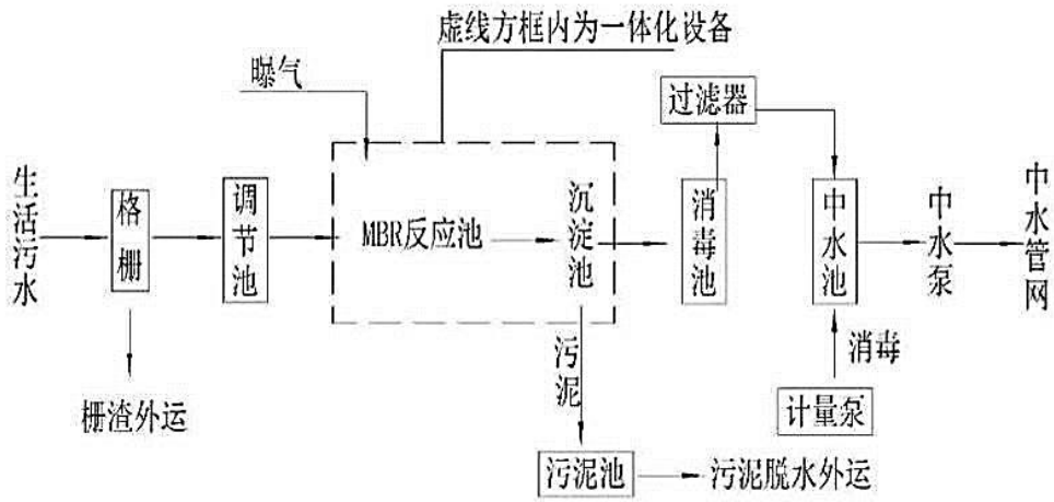
图 6.2-7 环境敏感区路段临时设施生活污水处理工艺流程
