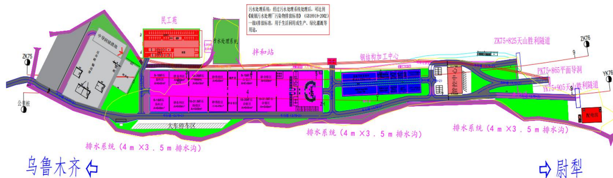
图 2.4-9 K75~K75+900 处的施工场地平面布置图
