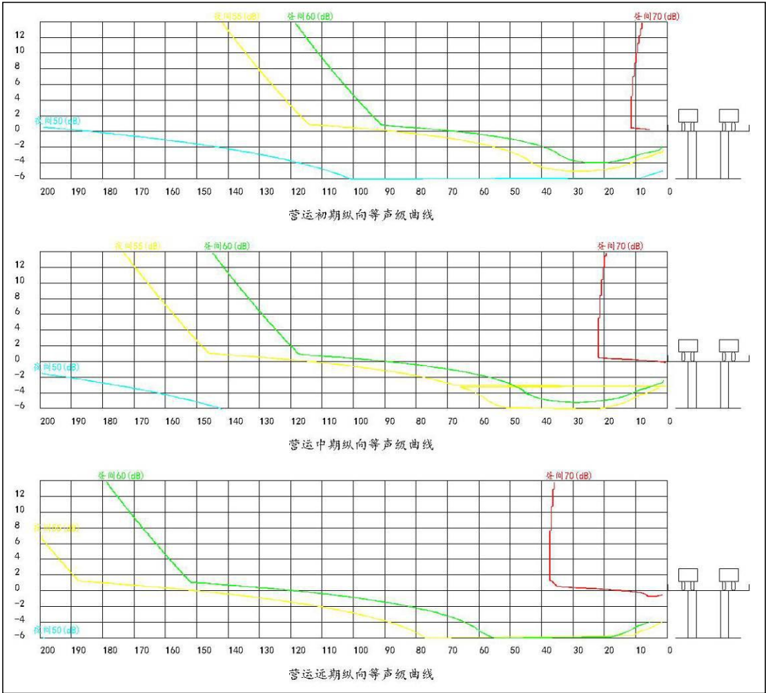
图 4.3-12 K148+200~K148+900 路段营运近、中、远期纵向等声级曲线图
