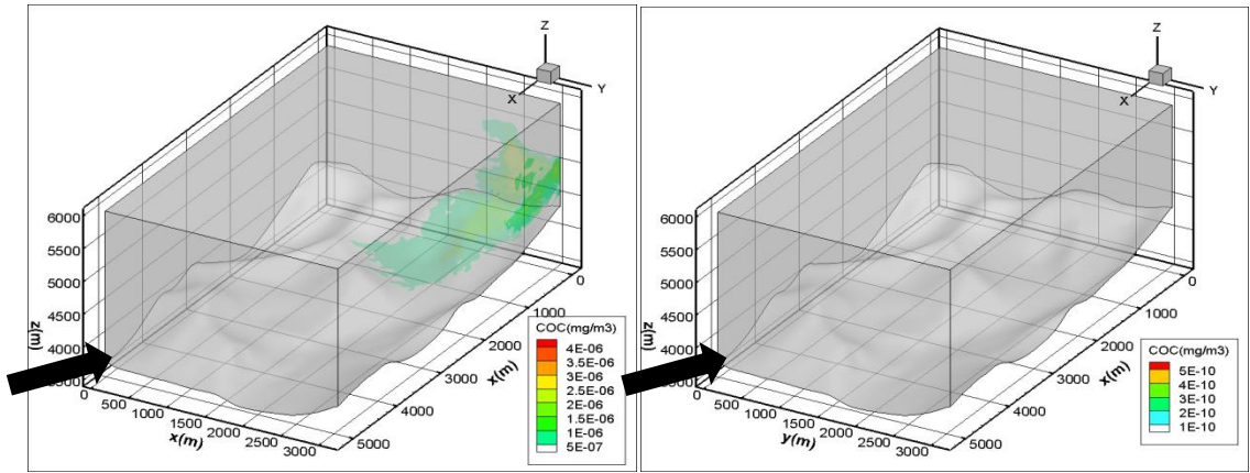
图 4.1.10-4 粉尘开始释放 0.5 小时、3 小时、10 小时、13 小时、18 小时和 24 小时后的粉尘浓度分布云图(13 小时后停止释放)
