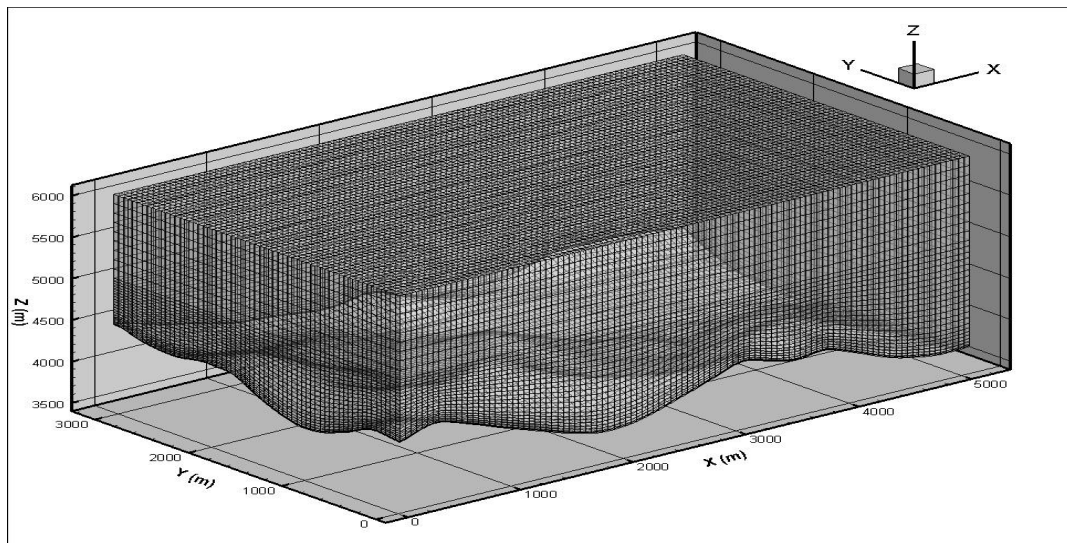
图4.1.10-2 计算模型示意图
