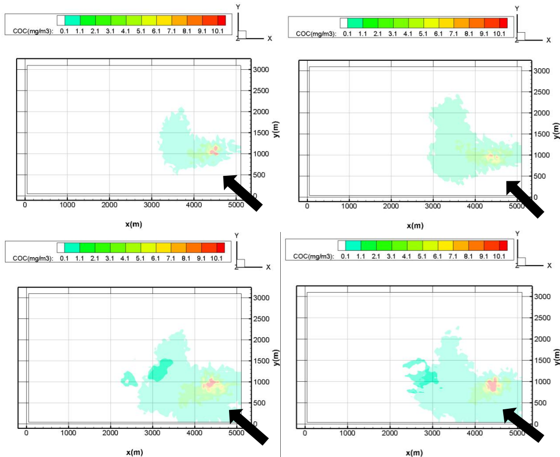
图 4.1.10-6 粉尘开始释放 0.5 小时、1 小时、3 小时和 5 小时后的粉尘浓度分布云图
