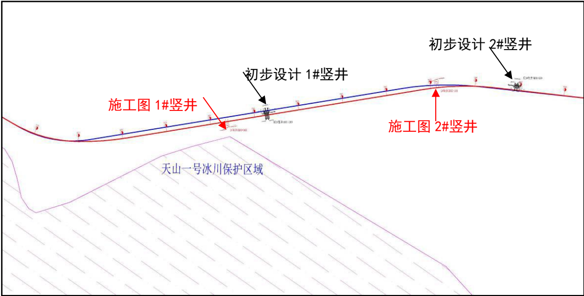
图 2.5.1-1 天山胜利隧道 1#、2#竖井位置变更示意图
