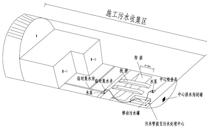
图6.2-3 隧道内施工废水收集典型设计图
