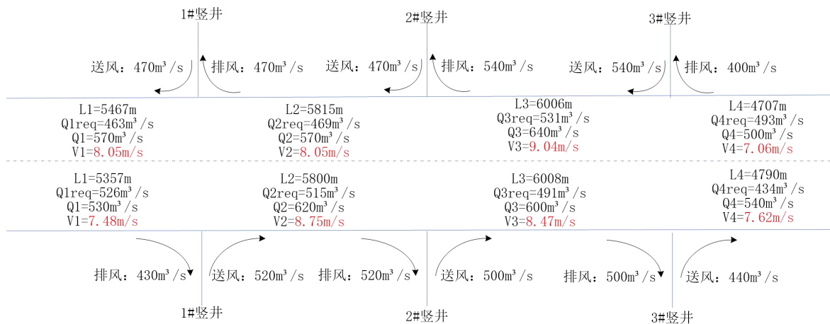
图 2.5.2-2 近期风量布置示意图
