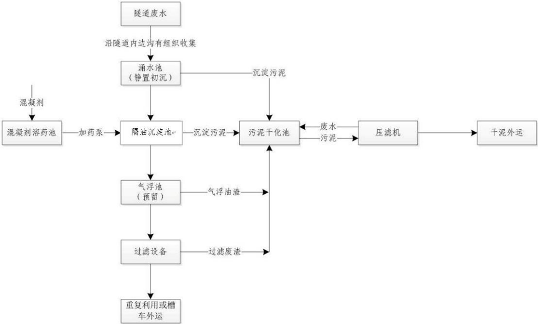
图2.5.5-6 隧道施工废水处理方案工艺流程图
