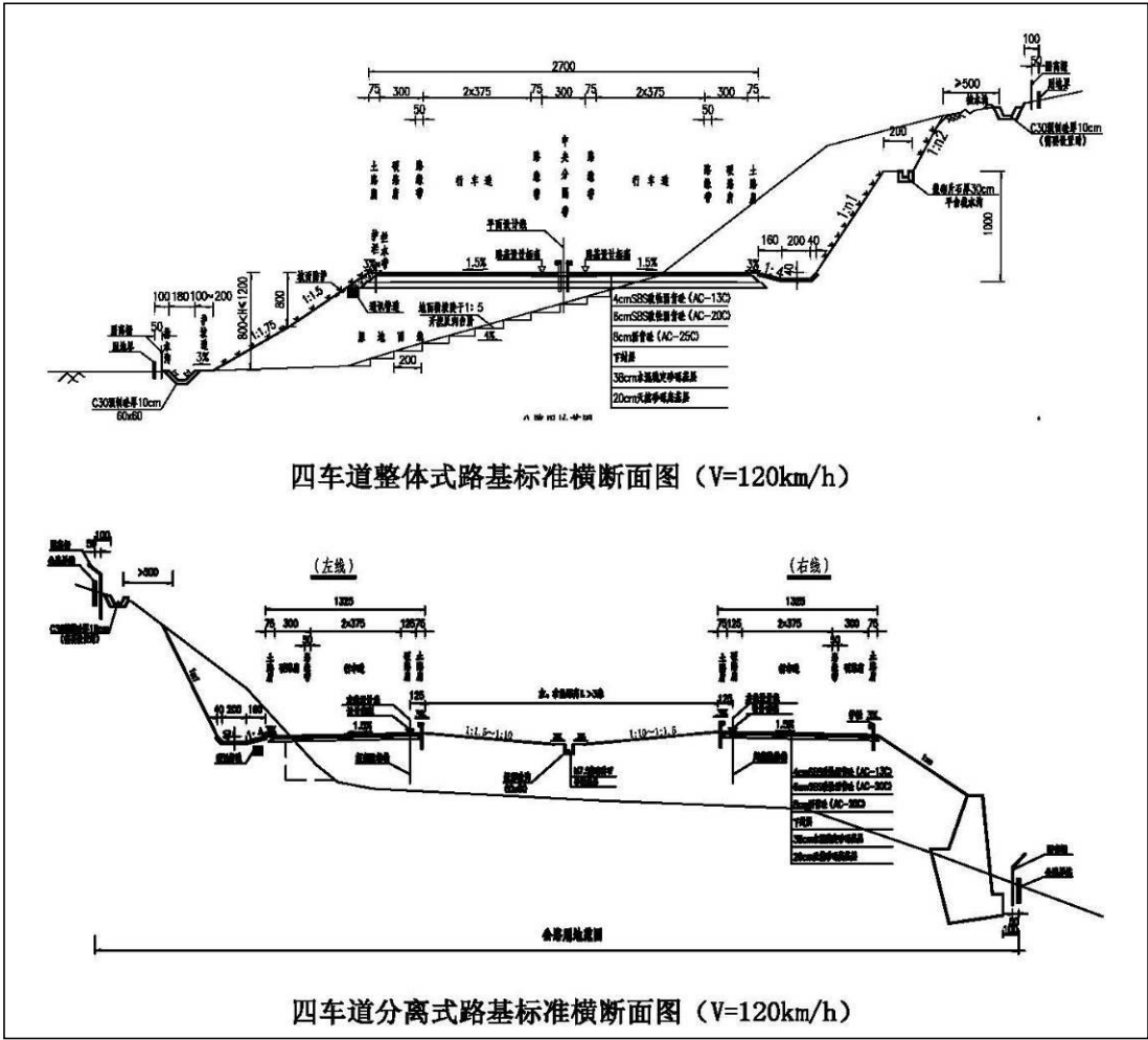
图 2.3-1b 拟建公路 27m 宽路基横断面图
