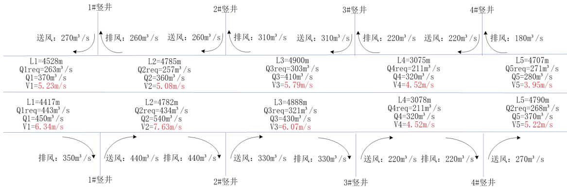
图 2.5.2-8 近期风量布置示意图
