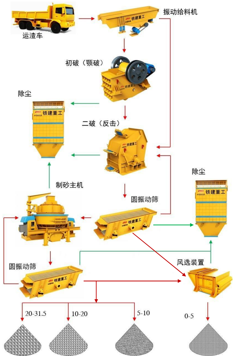
图 2.5.4-2 软岩干法洞渣处理工艺
