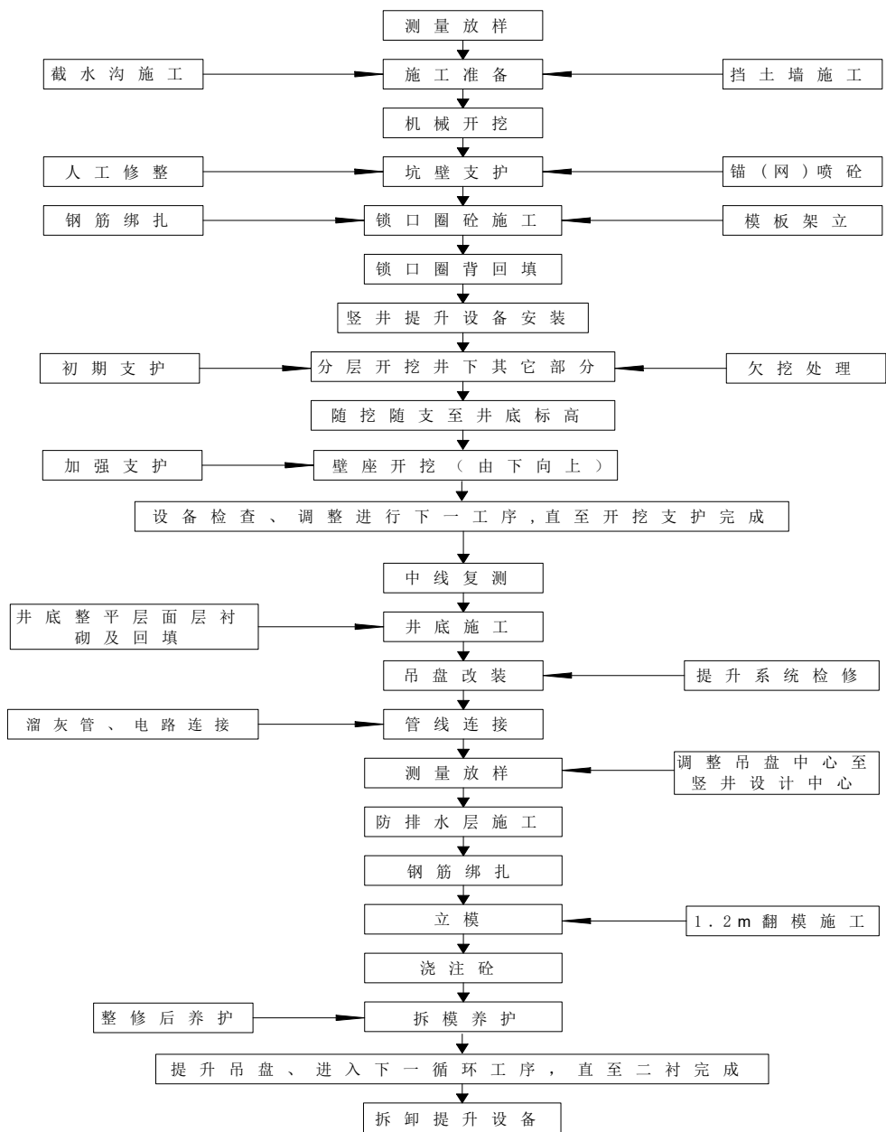
图 2.3.10-3 竖井施工工艺流程图
