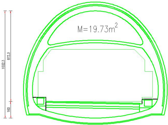
图 2.5.2-5 主洞顶部排烟道
