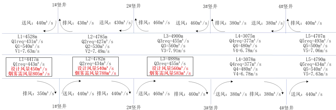
图 2.5.2-10 远期需采用静电除尘的区段
