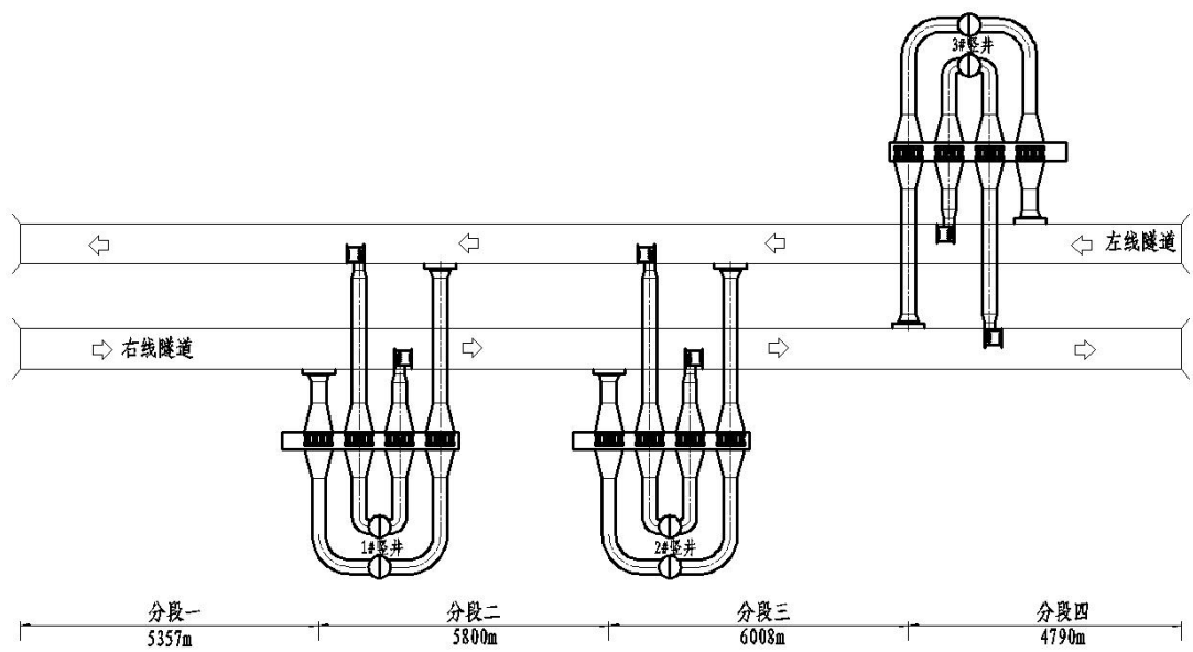
图 2.5.2-1 分四段纵向通风方案示意图
