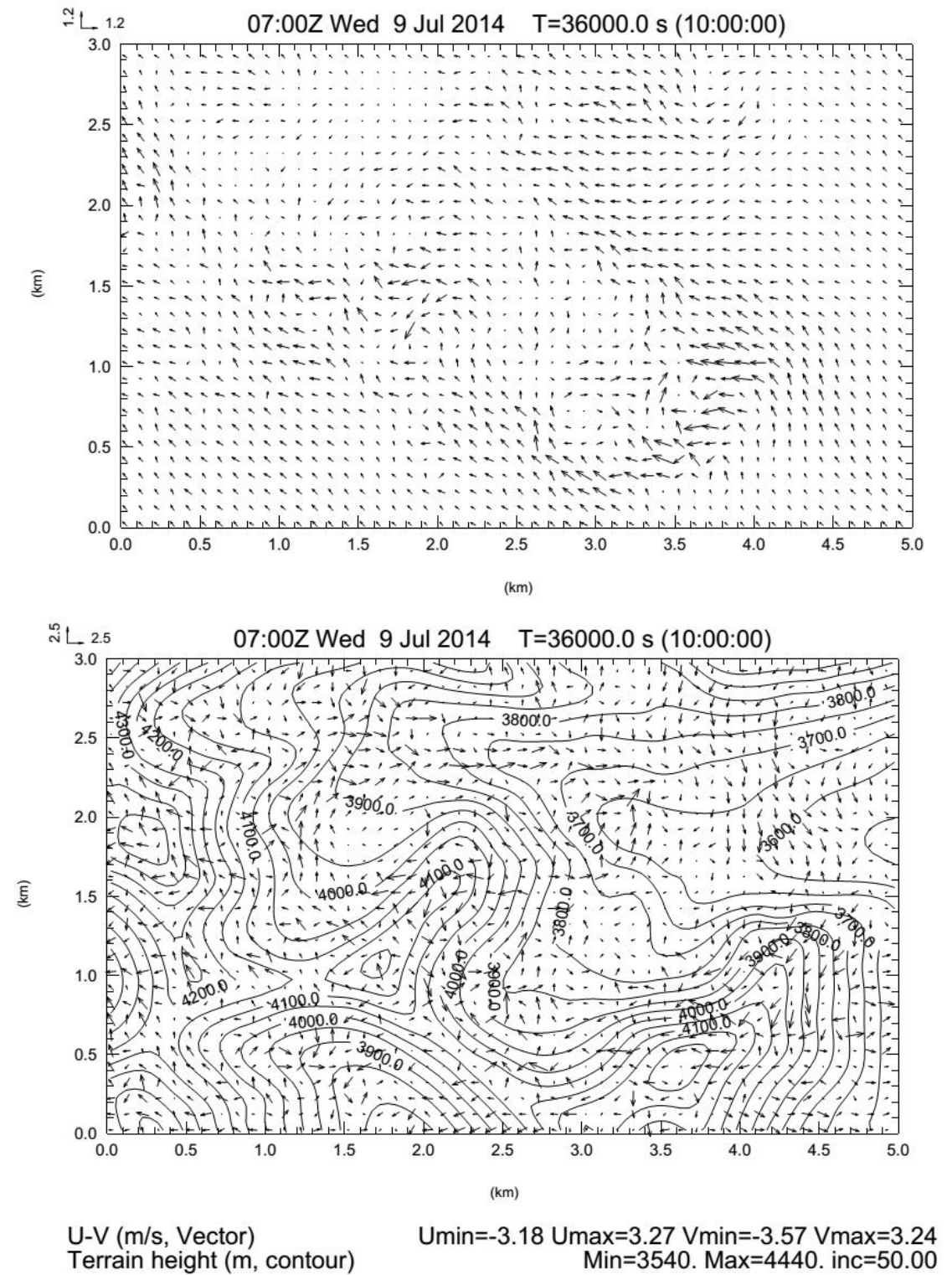
图 4.1.10-3 风场矢量图
