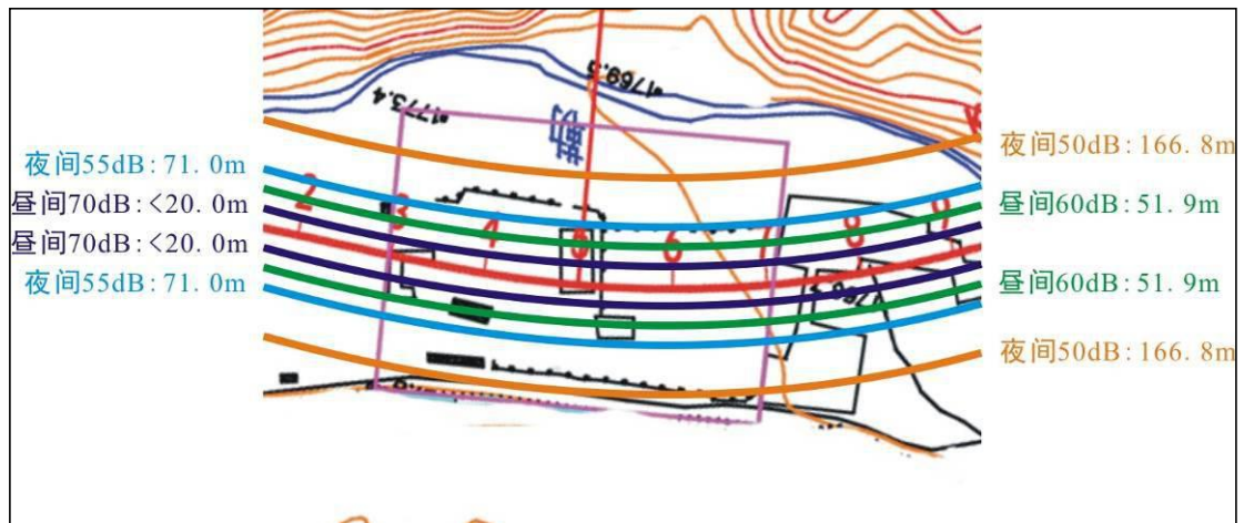
图 4.3-11 K148+200~K148+900 路段营运中期平面等声级曲线图
