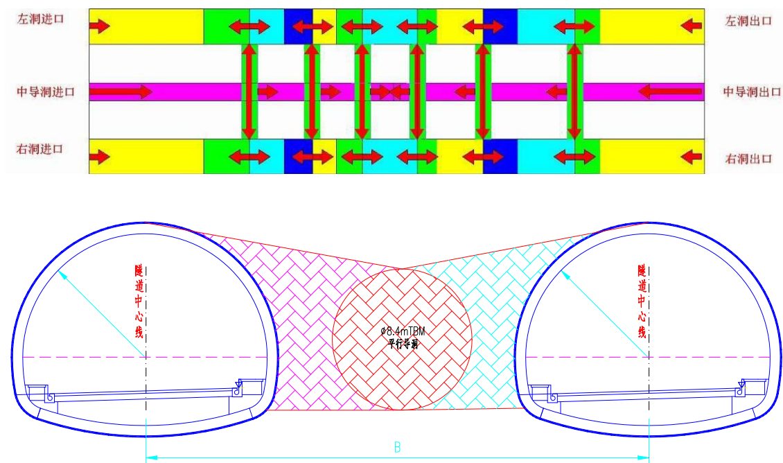
图 2.3.10-2 正洞钻爆+中导洞 1TBM+1 竖井钻爆法施工平面、横断面示意图
