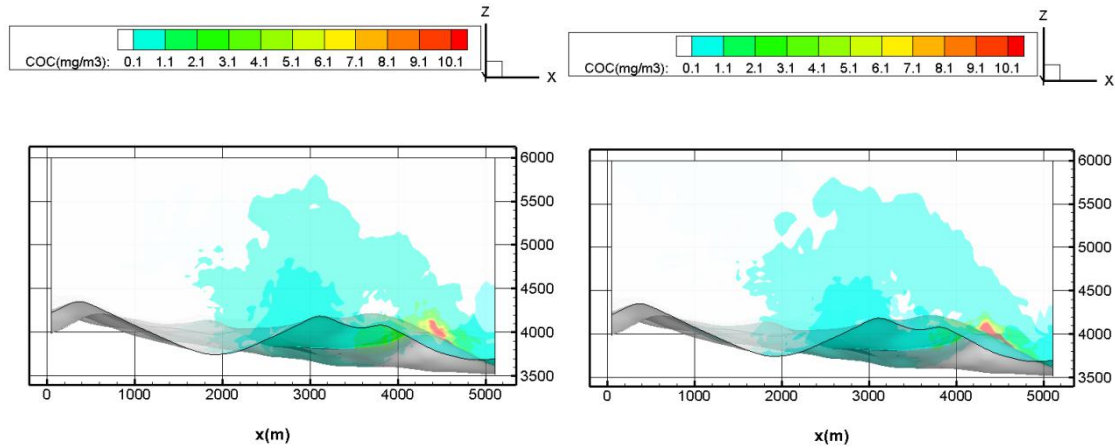
图 4.1.10-5 粉尘开始释放 3 小时和 5 小时后的粉尘浓度高度分布云图
