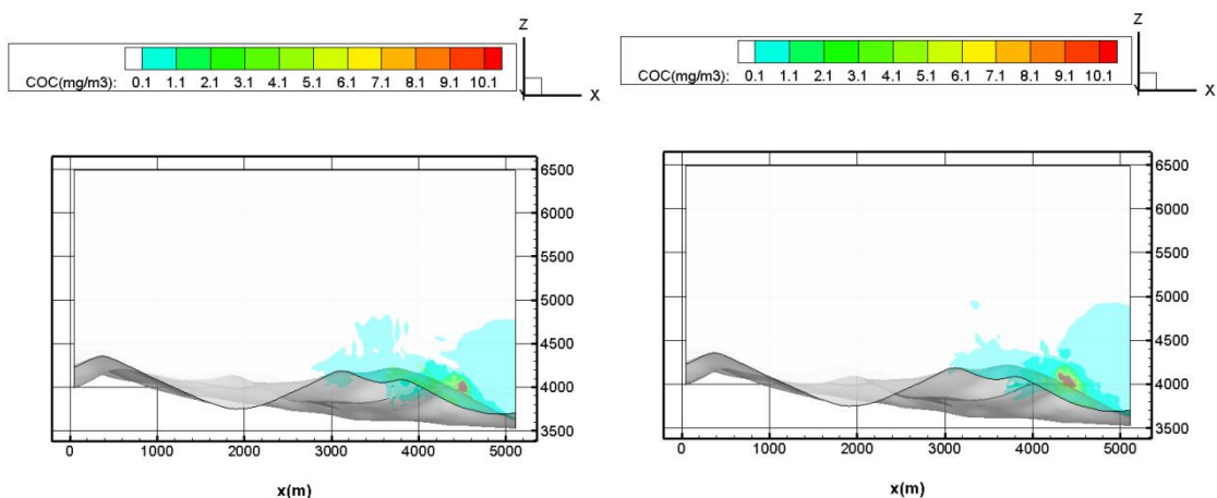
图 4.1.10-9 粉尘开始释放 1 小时和 5 小时后的粉尘浓度高度分布云图
