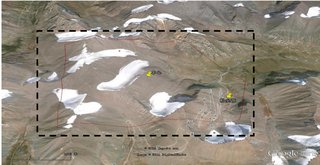
图4.1.10-1 冰川区域示意图
