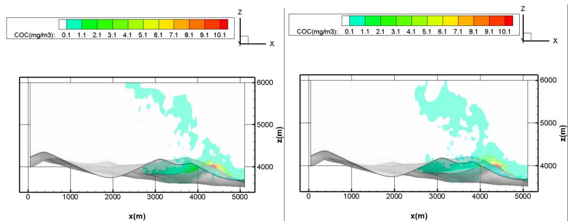
图 4.1.10-7 粉尘开始释放 1 小时和 5 小时后的粉尘浓度高度分布云图
