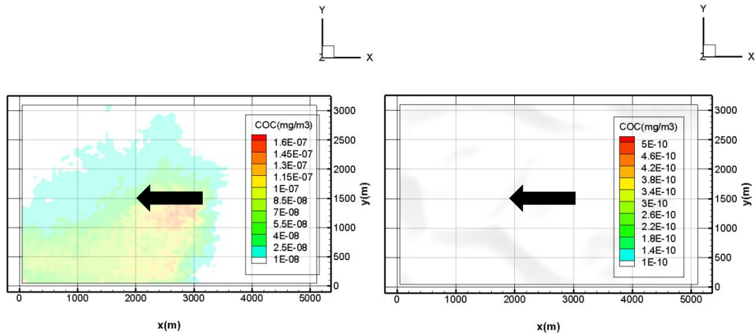
图 4.1.10-8 粉尘开始释放 1 小时、3 小时、10 小时、13 小时、18 小时和 24 小时后的粉尘浓度分布云图(13 小时后停止释放)
