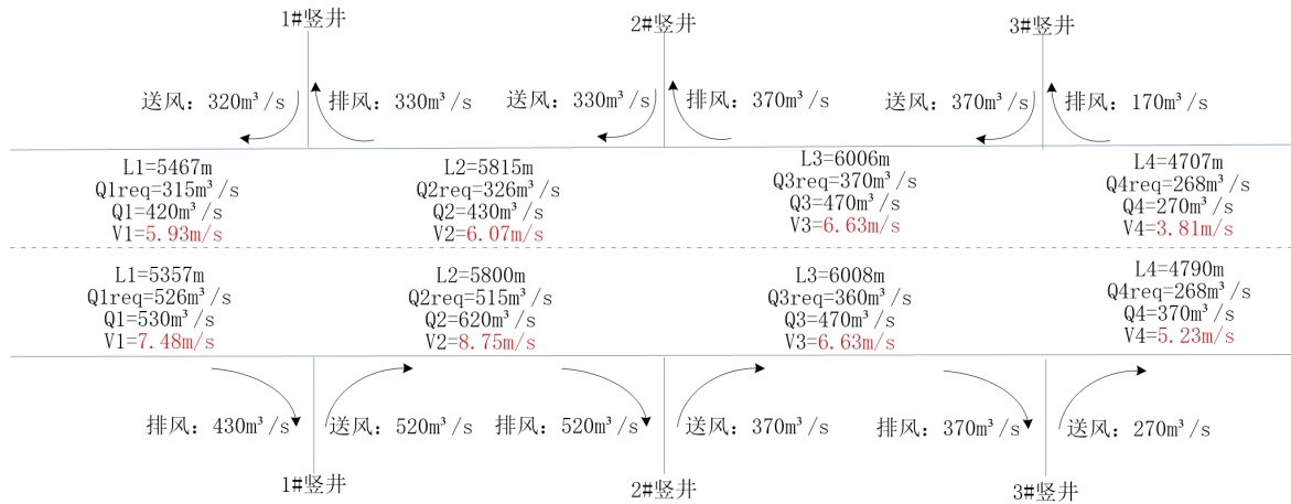
图 2.5.2-2 近期风量布置示意图
