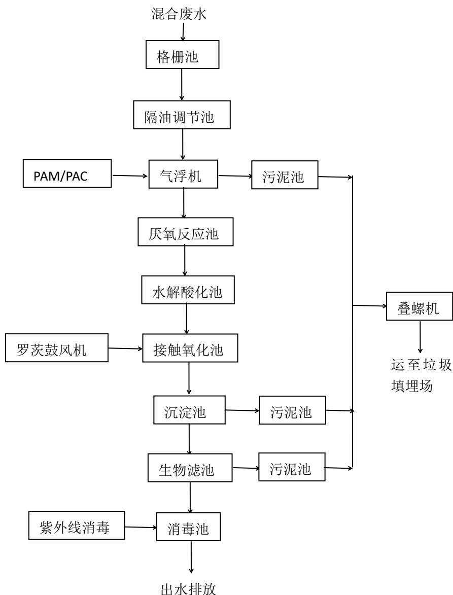
图 6.2-1 污水处理站工艺流程图
