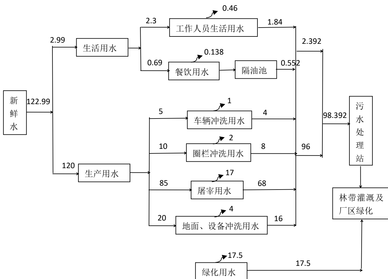
图 3.2-5 项目水平衡图 (单位: m 3 /d)
