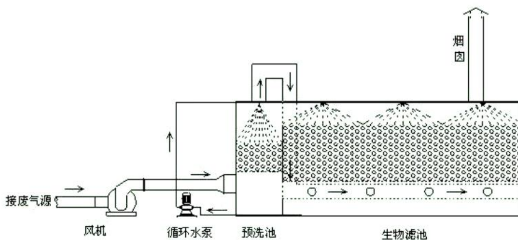
图 6.2-2 一体式生物滤池除臭装置工艺设备示意图
