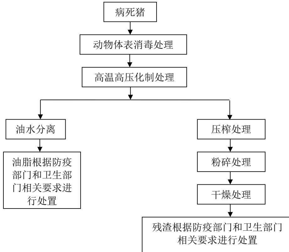
图3.1-7 项目病、死猪尸体无害化处理工艺图
