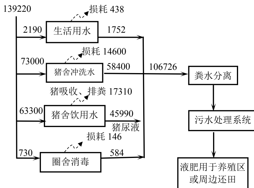
图3.1-1 项目水量平衡图(单位：m 3 /a)
