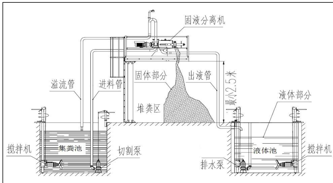
图 3.1-5 固液分离系统断面示意图
