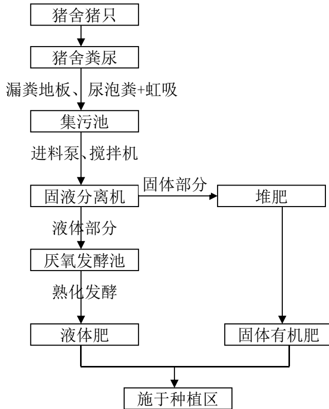
图 3.1-4 粪肥处理利用工艺流程图
