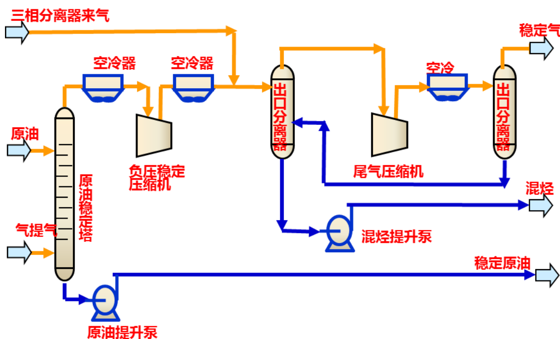
图 3.1-6 原油负压稳定脱硫工艺图
