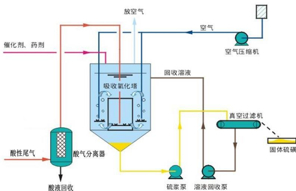
图 3.1-9 自循环硫磺回收部分工艺流程
