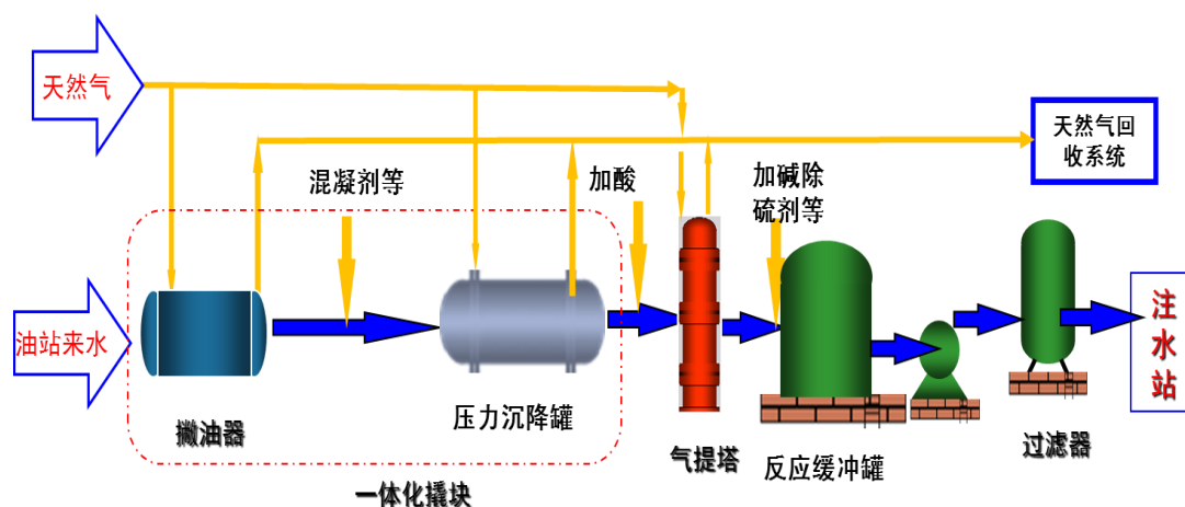
图 3.1-10 污水处理工艺流程
