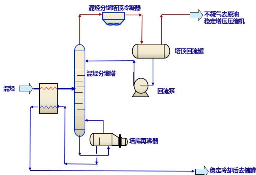
图 3.1-7 混烃分馏工艺流程图
