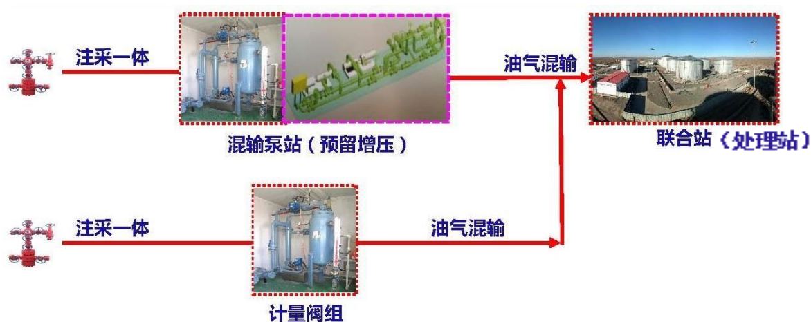
图 3.2-1 本项目布站工艺流程图
