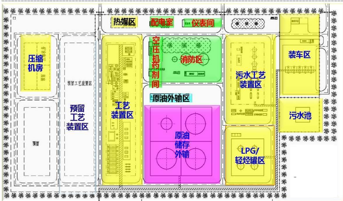
图 3.1-4 五号联合站平面布置示意图
