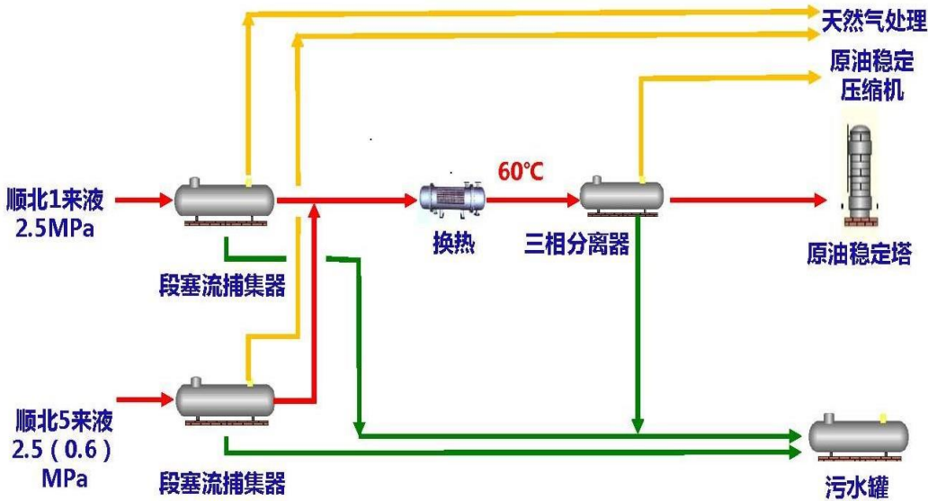
图 3.1-5 五号联合站原油处理工艺
