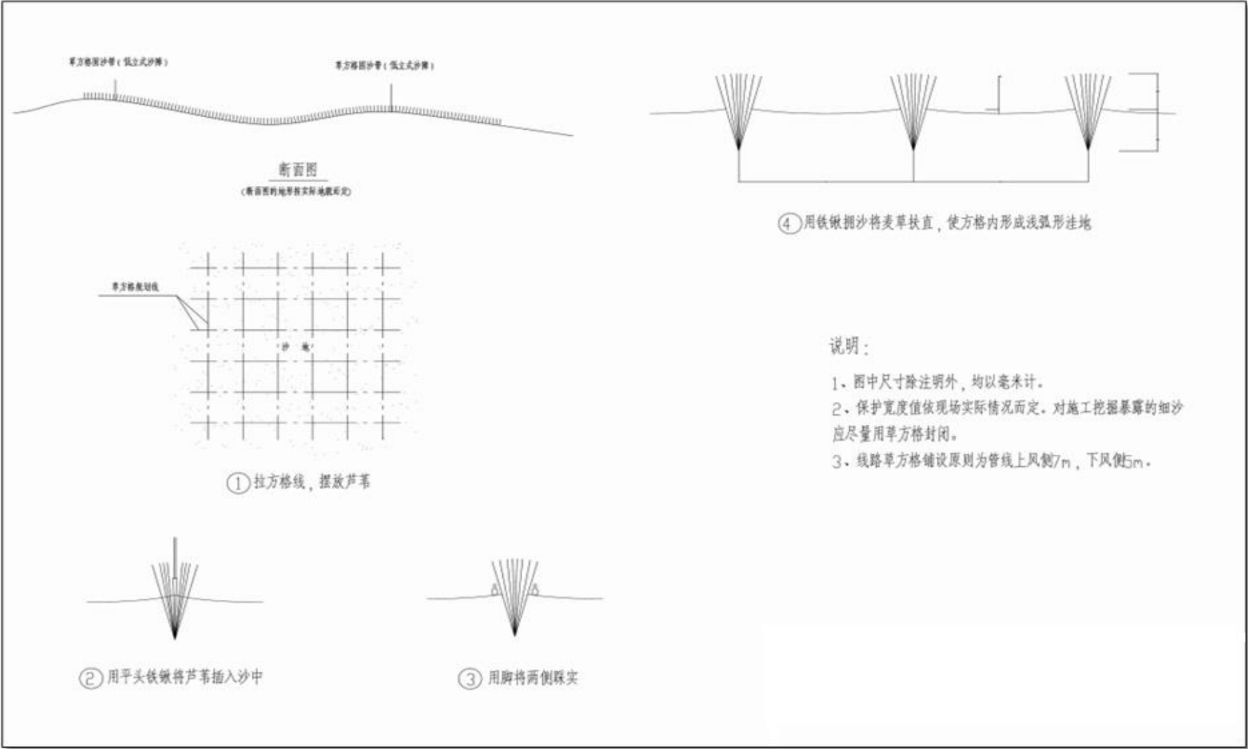
图 6.1-1 固沙草方格设置通用图
