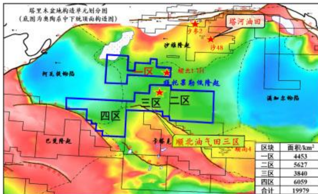
图 5.4-1 塔里木盆地顺北构造单元划分图
