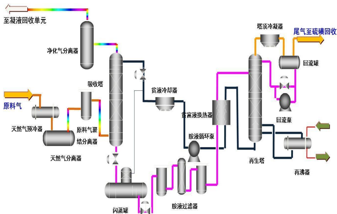
图 3.1-8 砒胺法脱硫部分工艺流程图
