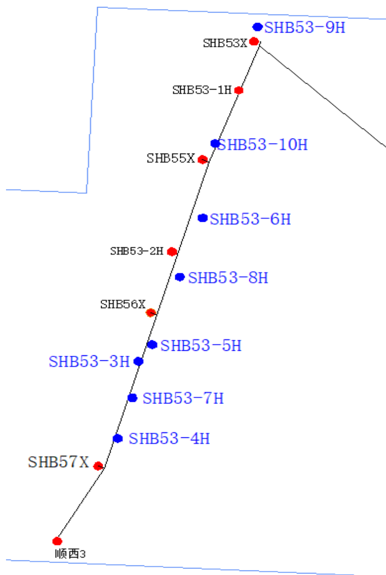
图 3.1-3 顺北三区 5 条带井位部署图
