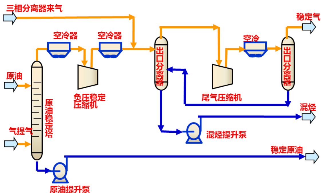
图 3.1-8 原油负压稳定脱硫工艺图
