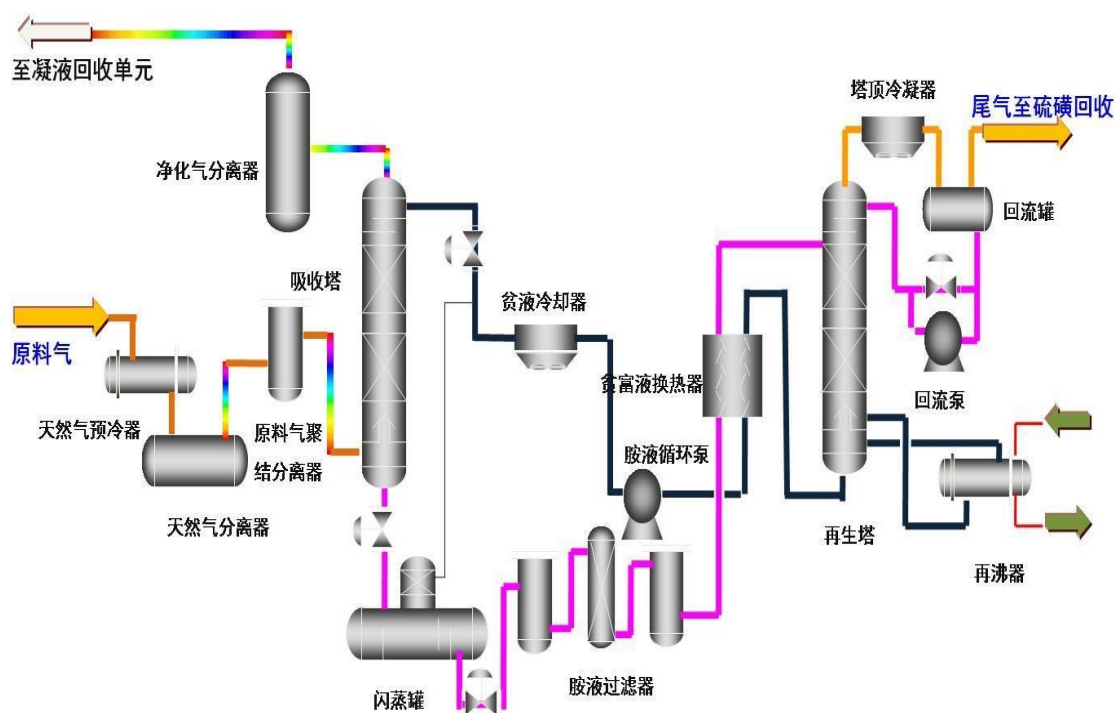
图 3.1-10 胺法脱硫部分工艺流程图
