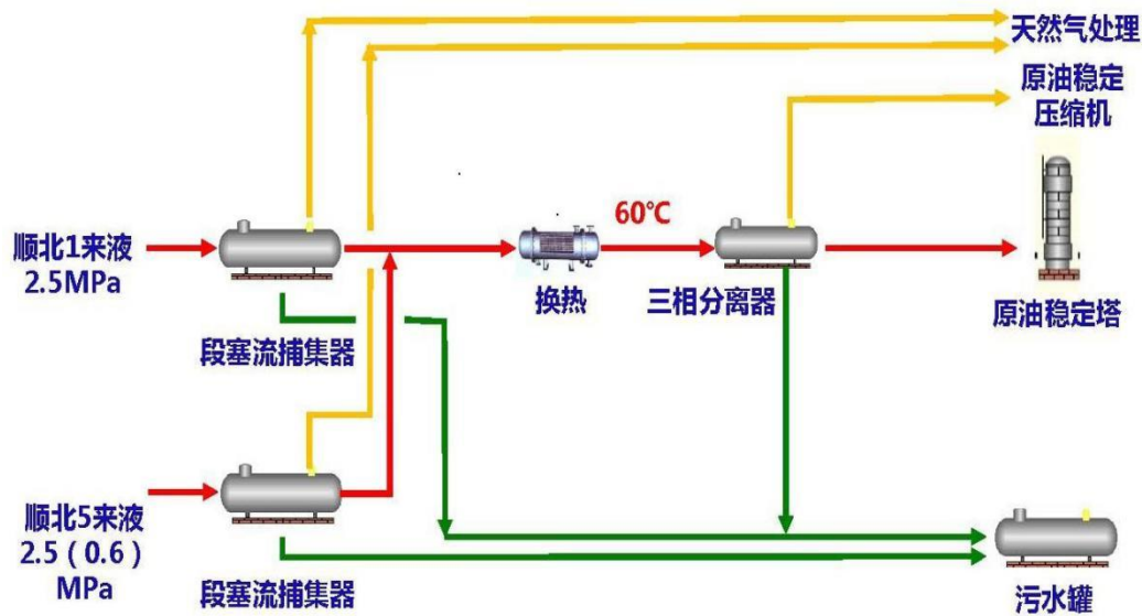
图 3.1-7 五号联合站原油处理工艺
