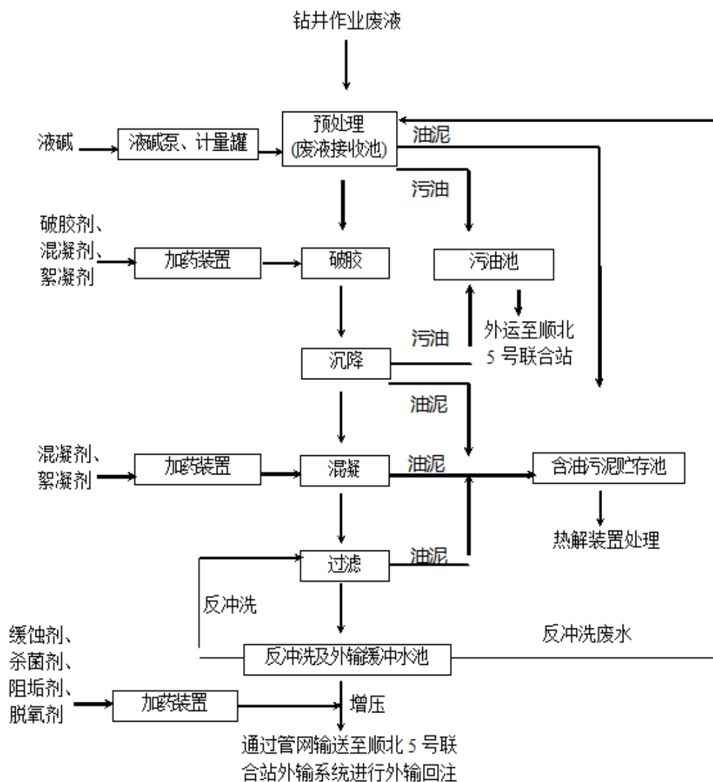
图 3.1-14 废液处理工艺流程
