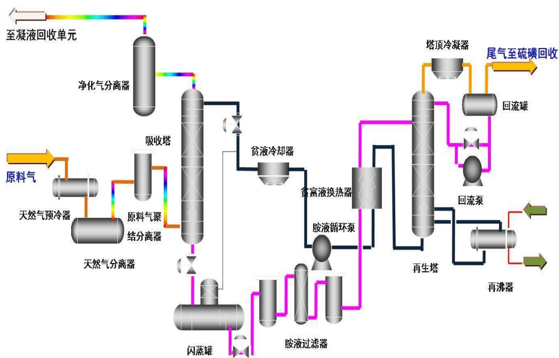
图 3.1-11 砵胺法脱硫部分工艺流程图
