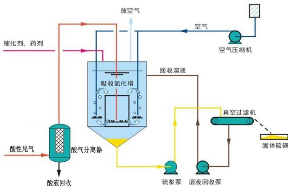
图 3.1-12 自循环硫磺回收部分工艺流程
