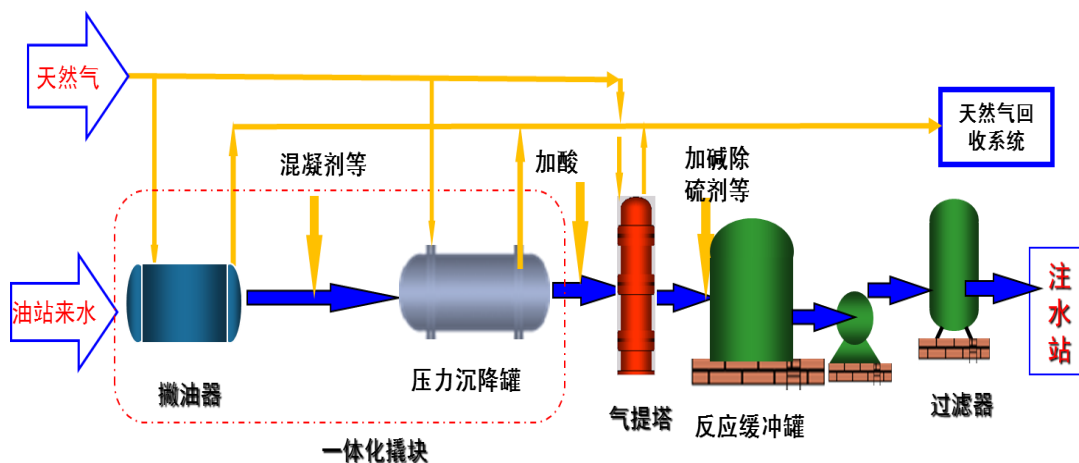
图 3.1-13 污水处理工艺流程
