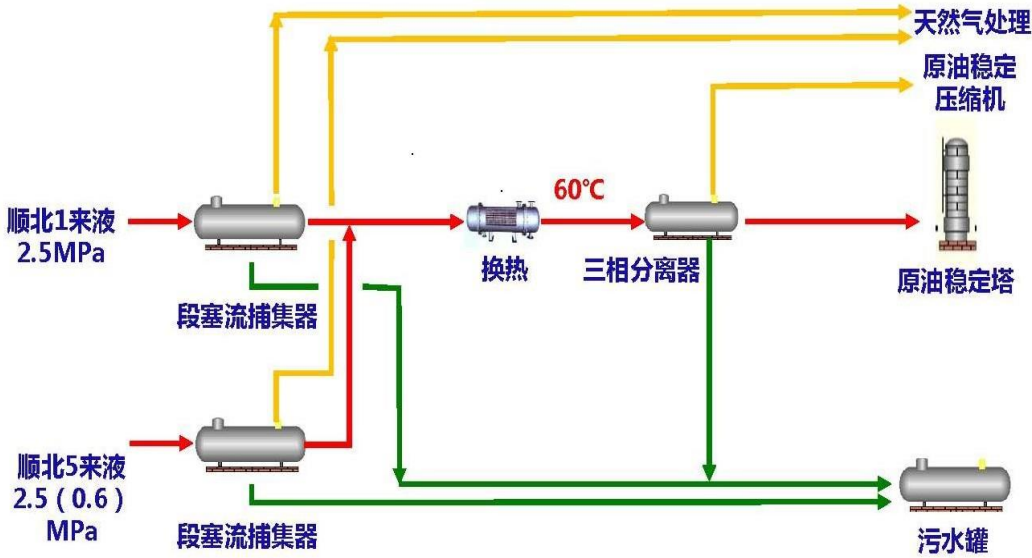
图 3.1-8 五号联合站原油处理工艺
