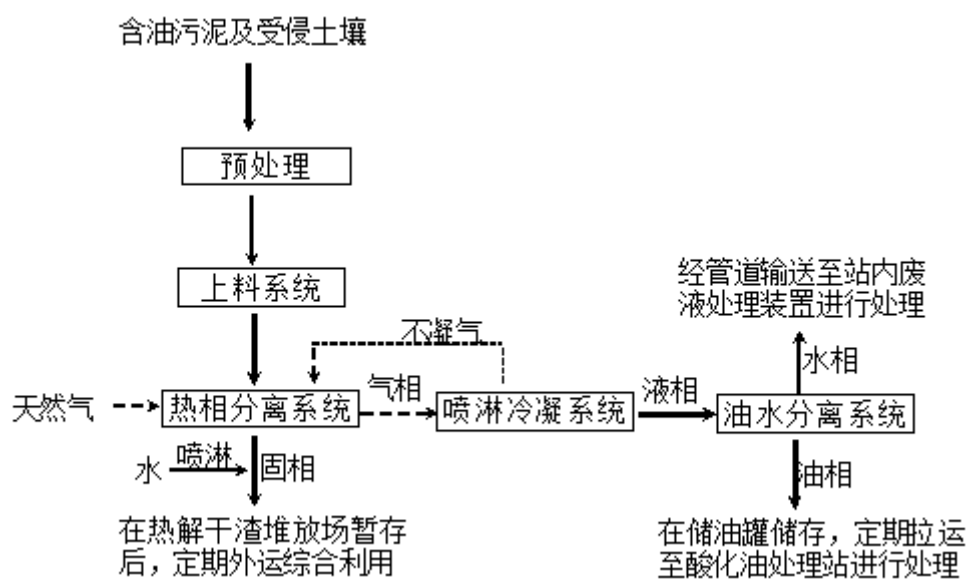
图 3.1-15 含油污泥处理工艺流程
