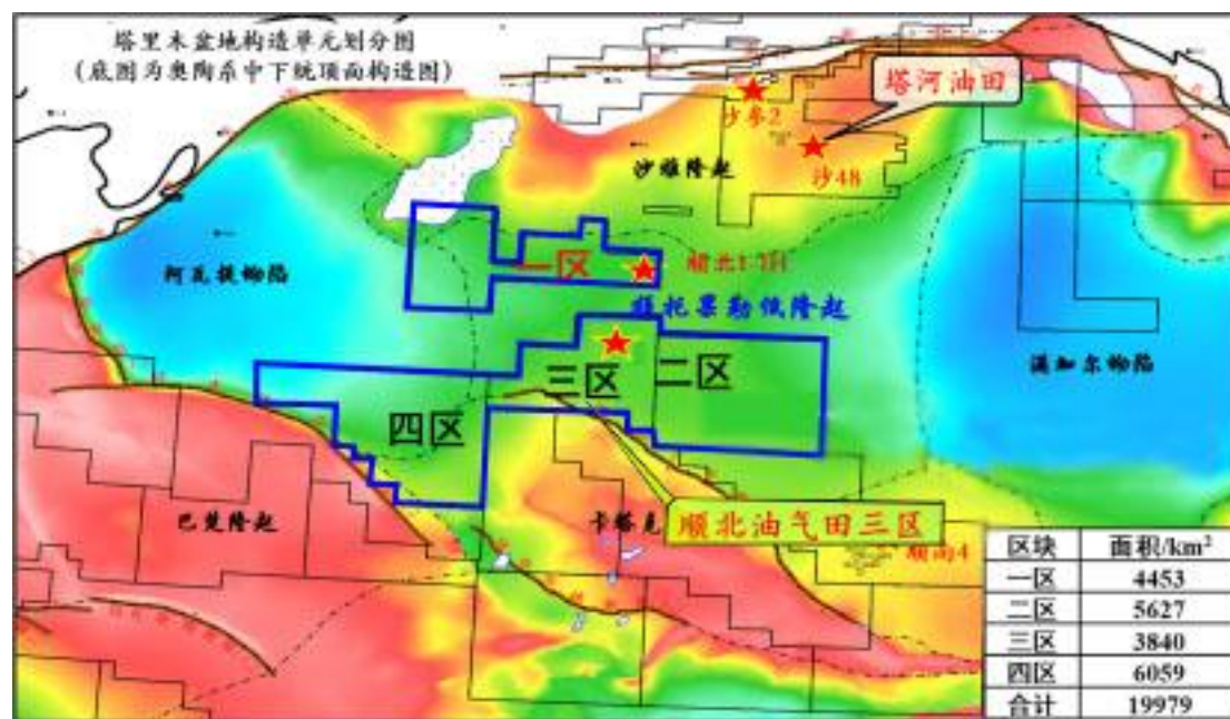
图 5.4-1 塔里木盆地顺北构造单元划分图
