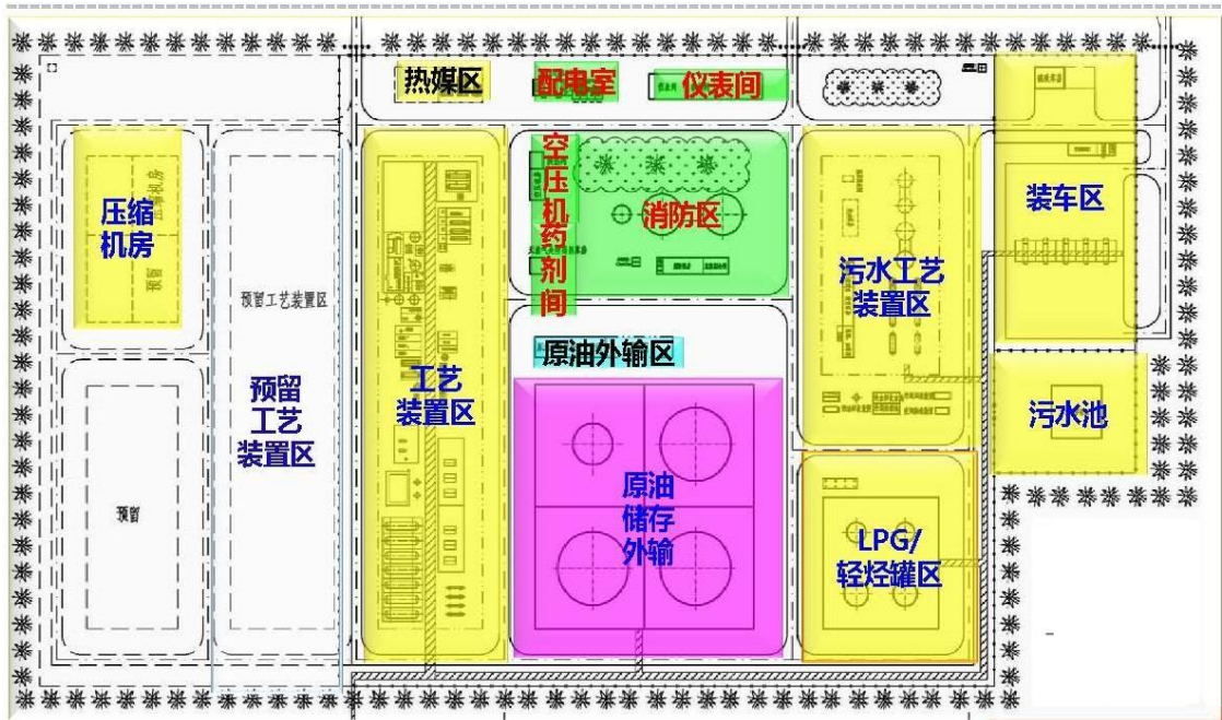
图 3.1-7 五号联合站平面布置示意图
