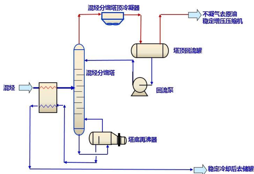
图 3.1-10 混烃分馏工艺流程图
