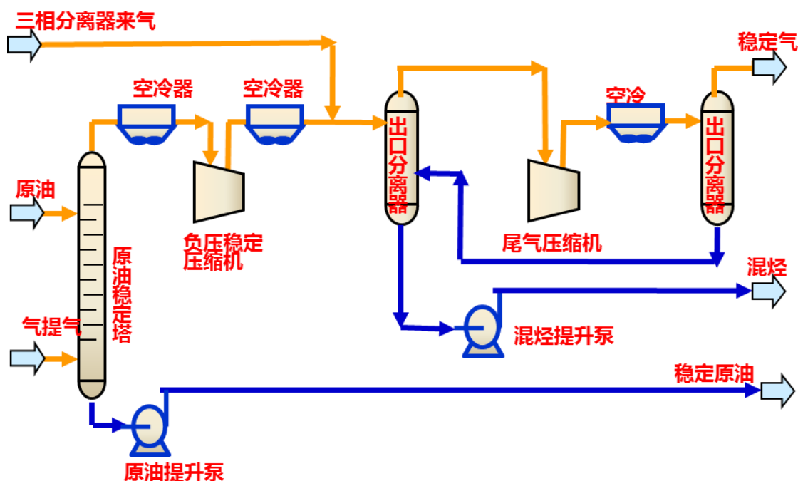
图 3.1-9 原油负压稳定脱硫工艺图
