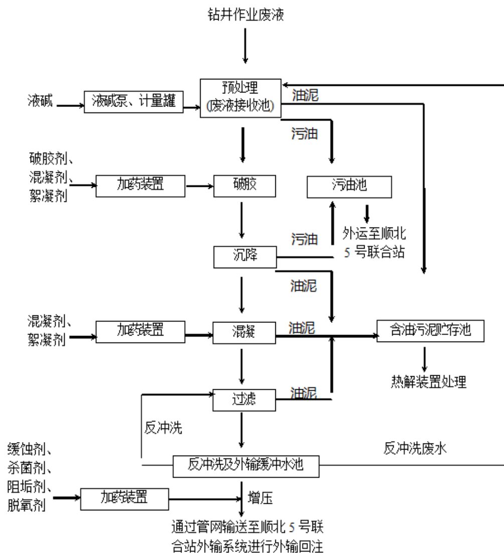
图 3.1-13 废液处理工艺流程
