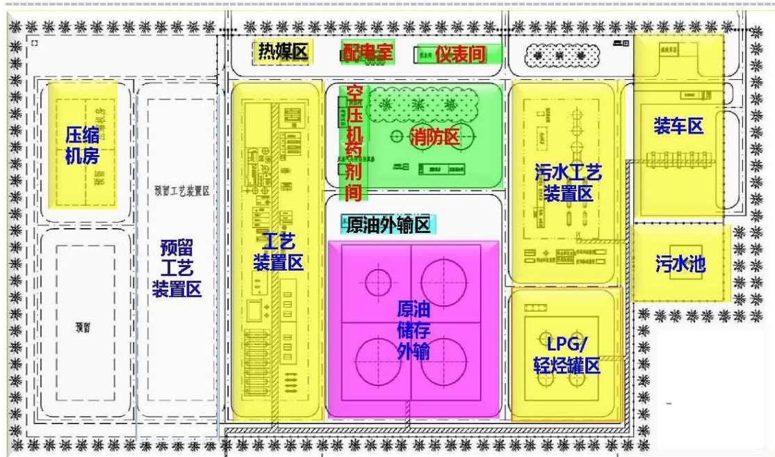
图 3.1-6 五号联合站平面布置示意图
