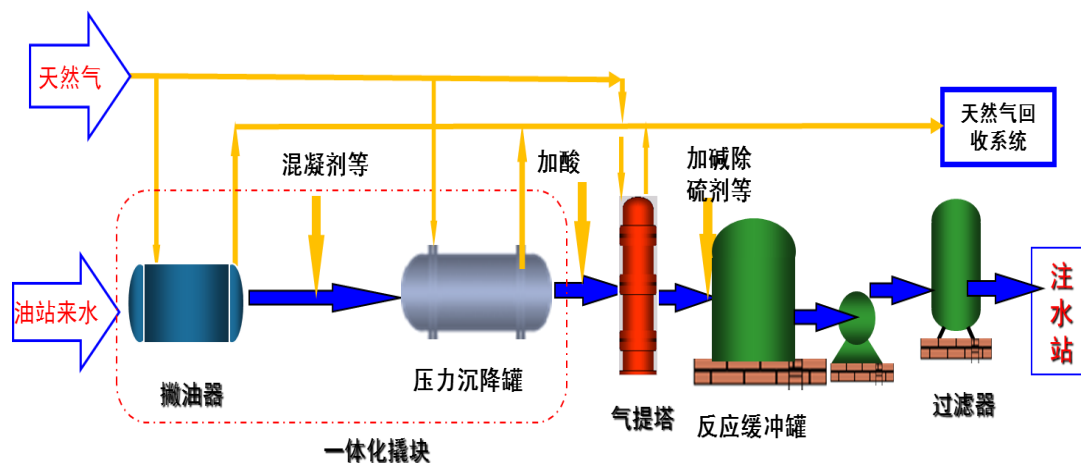
图 3.1-12 污水处理工艺流程
