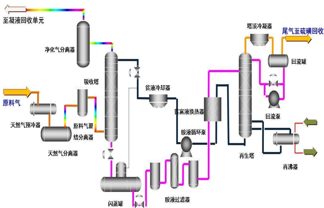
图 3.1-10 砒胺法脱硫部分工艺流程图
