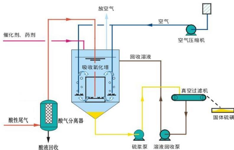
图 3.1-11 自循环硫磺回收部分工艺流程
