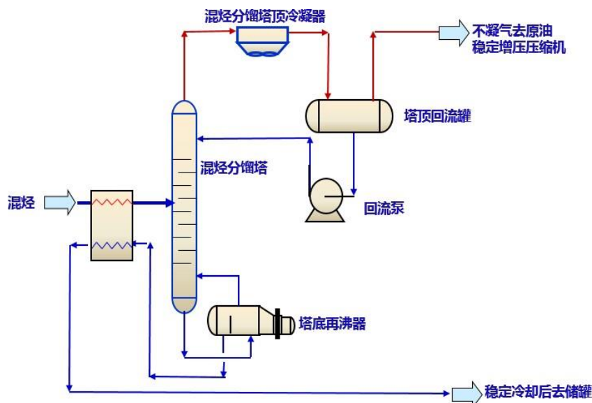
图 3.1-9 混烃分馏工艺流程图
