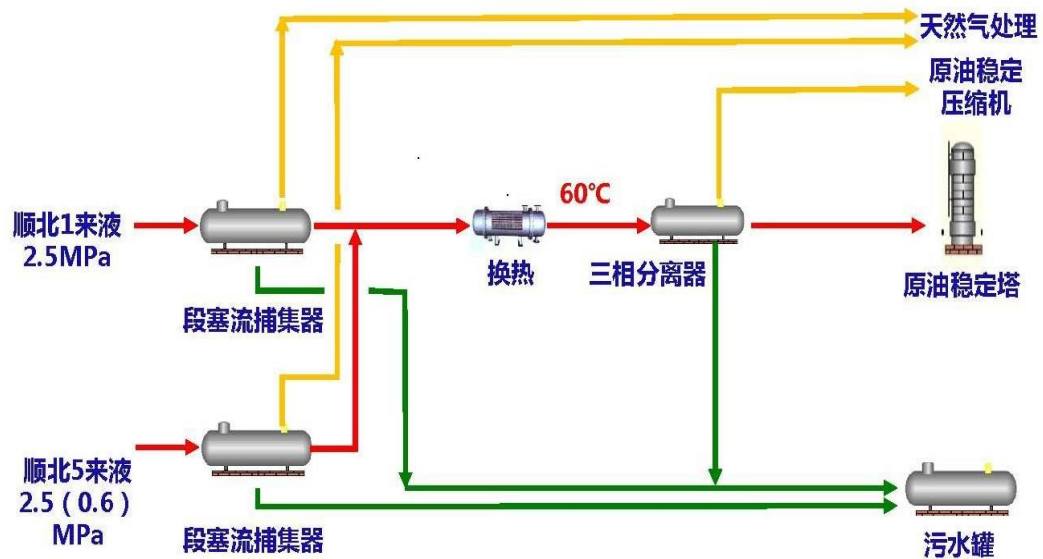
图 3.1-7 五号联合站原油处理工艺
