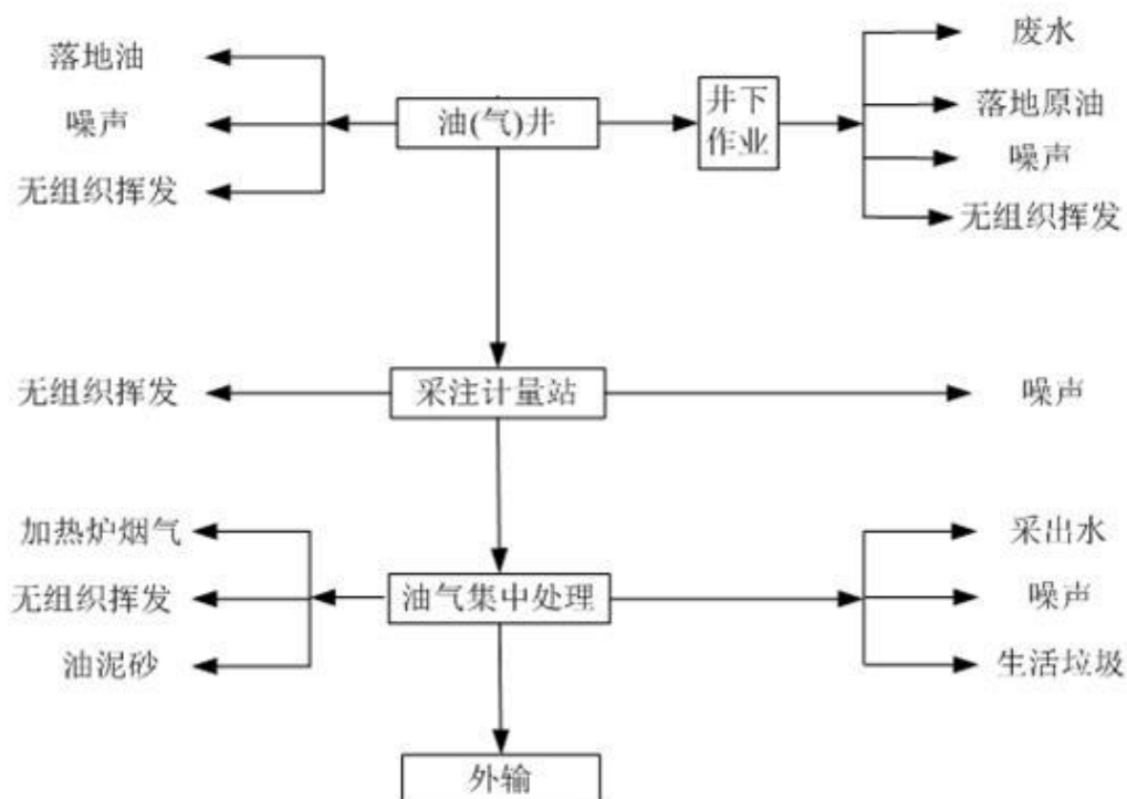
图 3.3-2 油田开发过程污染物排放流程
