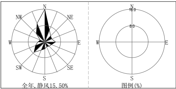
图 5.2-2 区域近 20 年风频玫瑰图
