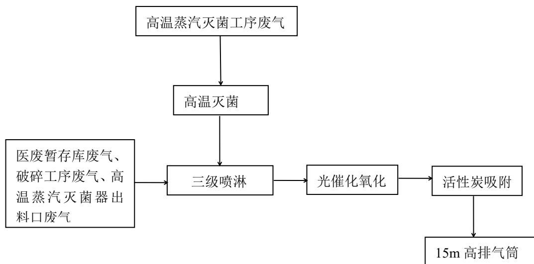
图 6.2-1 废气处理工艺流程图
