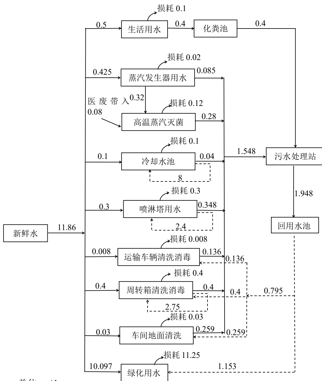
图 3.3-1 本项目水平衡图
