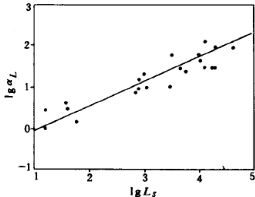
图 5.2-11 孔隙介质数值模型的 \lg \alpha L — \lg L_s 图
