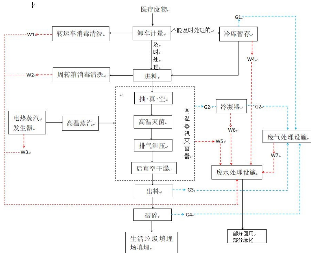
图 3.3-1 本项目工艺流程及产污节点示意简图
