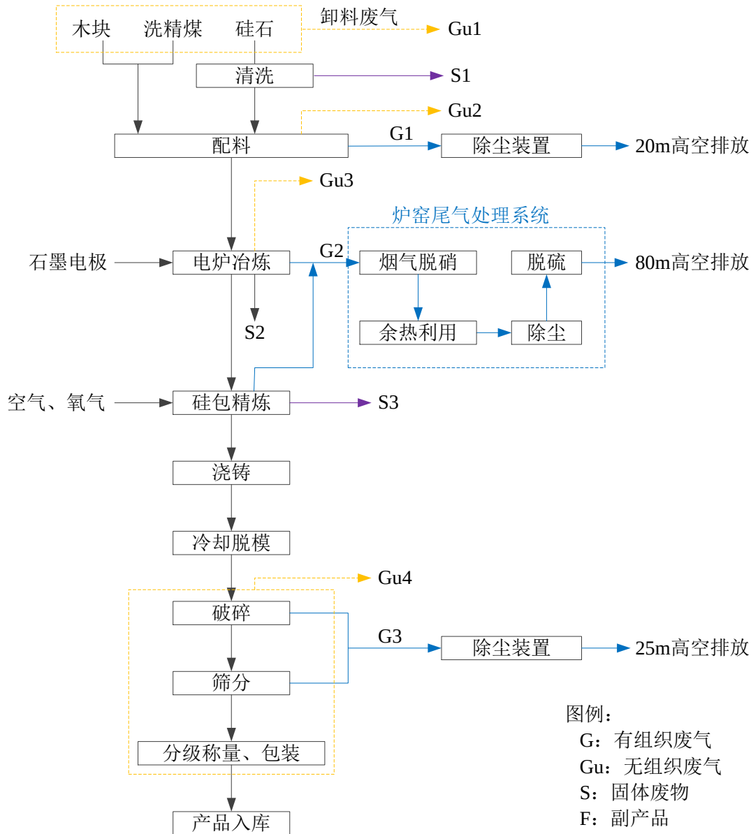
图 4.2-1 工业硅生产工艺流程及产污环节图
