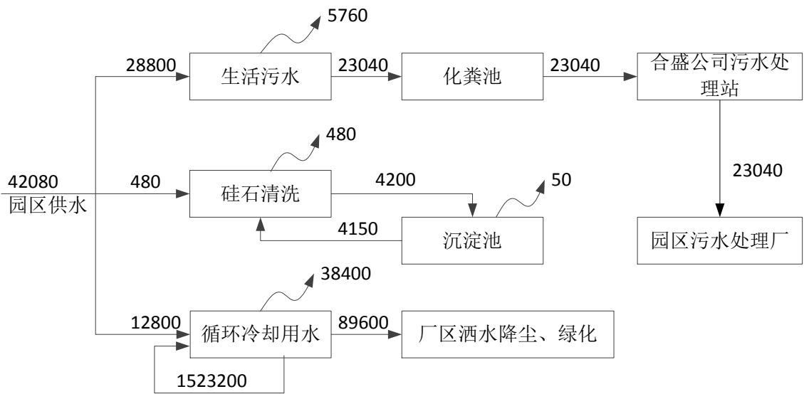
图 3.2-1 现有项目全厂水平衡图
