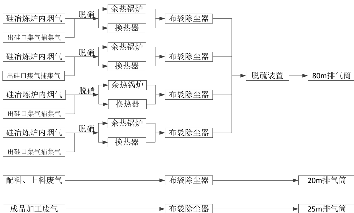
图 7.1-1 本项目有组织废气收集处理工艺路线图
