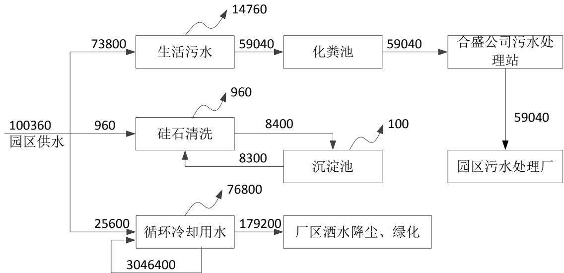
图 4.2-4 项目建成后全厂水平衡图 (t/a)
