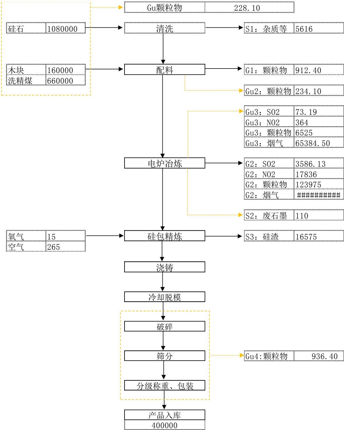
图 4.2-1 工业硅生产物料平衡图 (单位: t/a)
