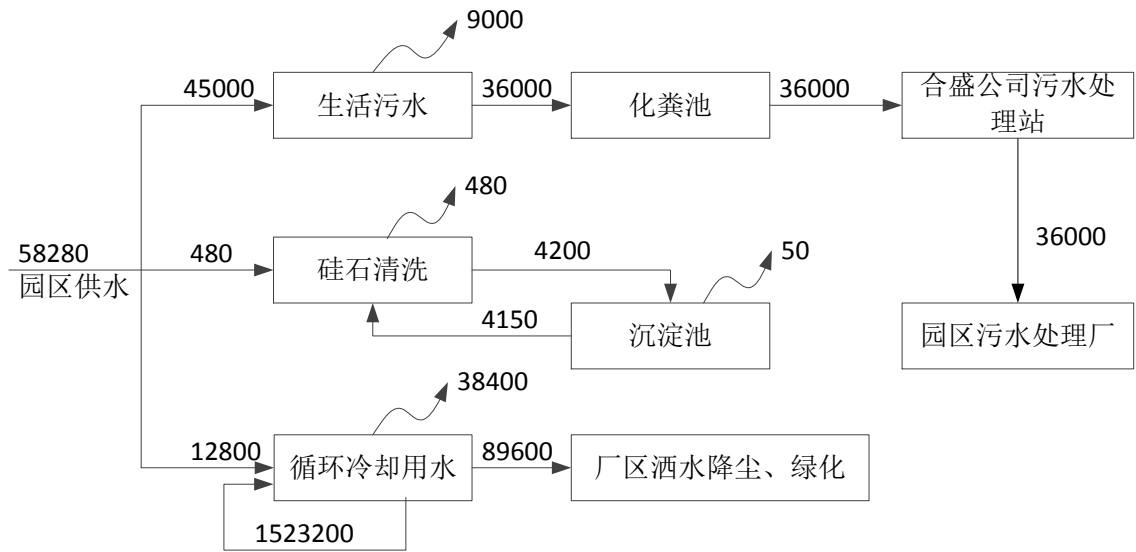
图 4.2-3 本项目水平衡图 (t/a)
