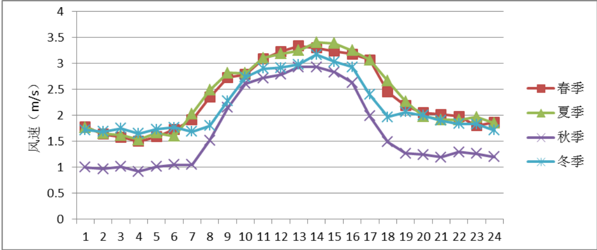
图 6.1-3 季小时平均风速的日变化曲线
