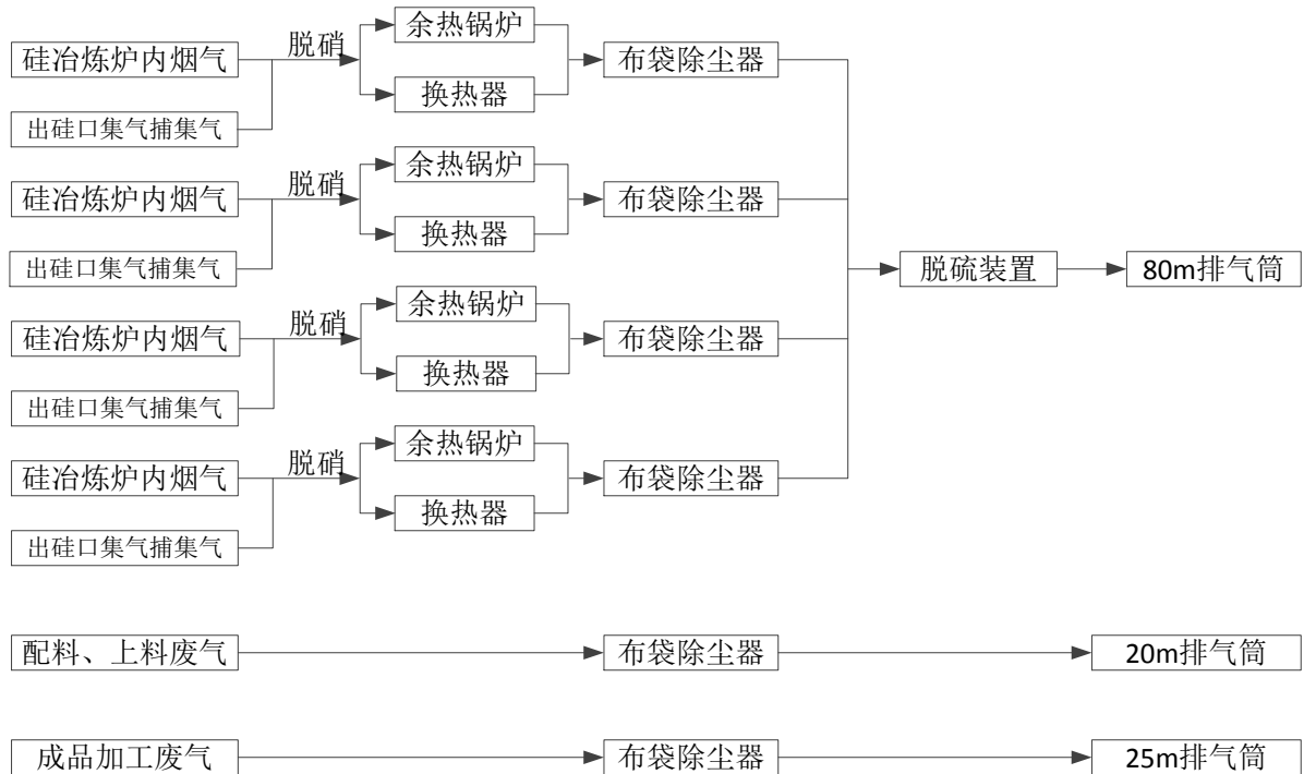
图 3.3-1 现有项目有组织废气收集处理工艺路线图
