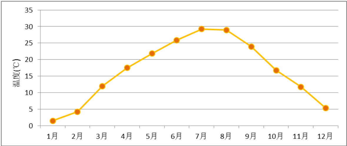
图 6.1-1 年平均温度的月变化曲线
