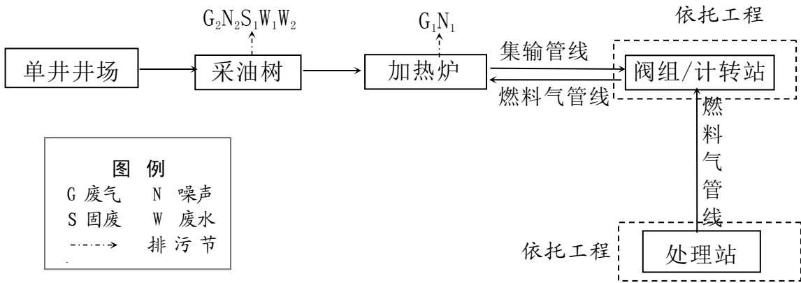
图 3.2-8 油气开采及集输工艺流程图
