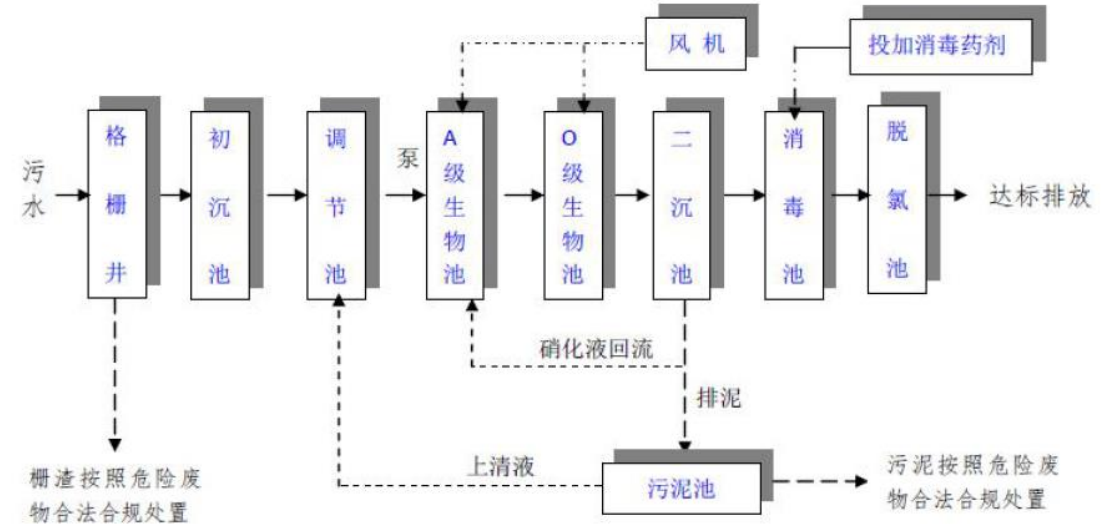
图 6.2-1 医疗废水处理工艺流程图
