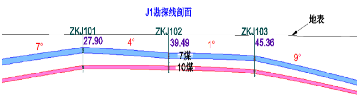
图 3.2-6 J1 勘探线剖面图
