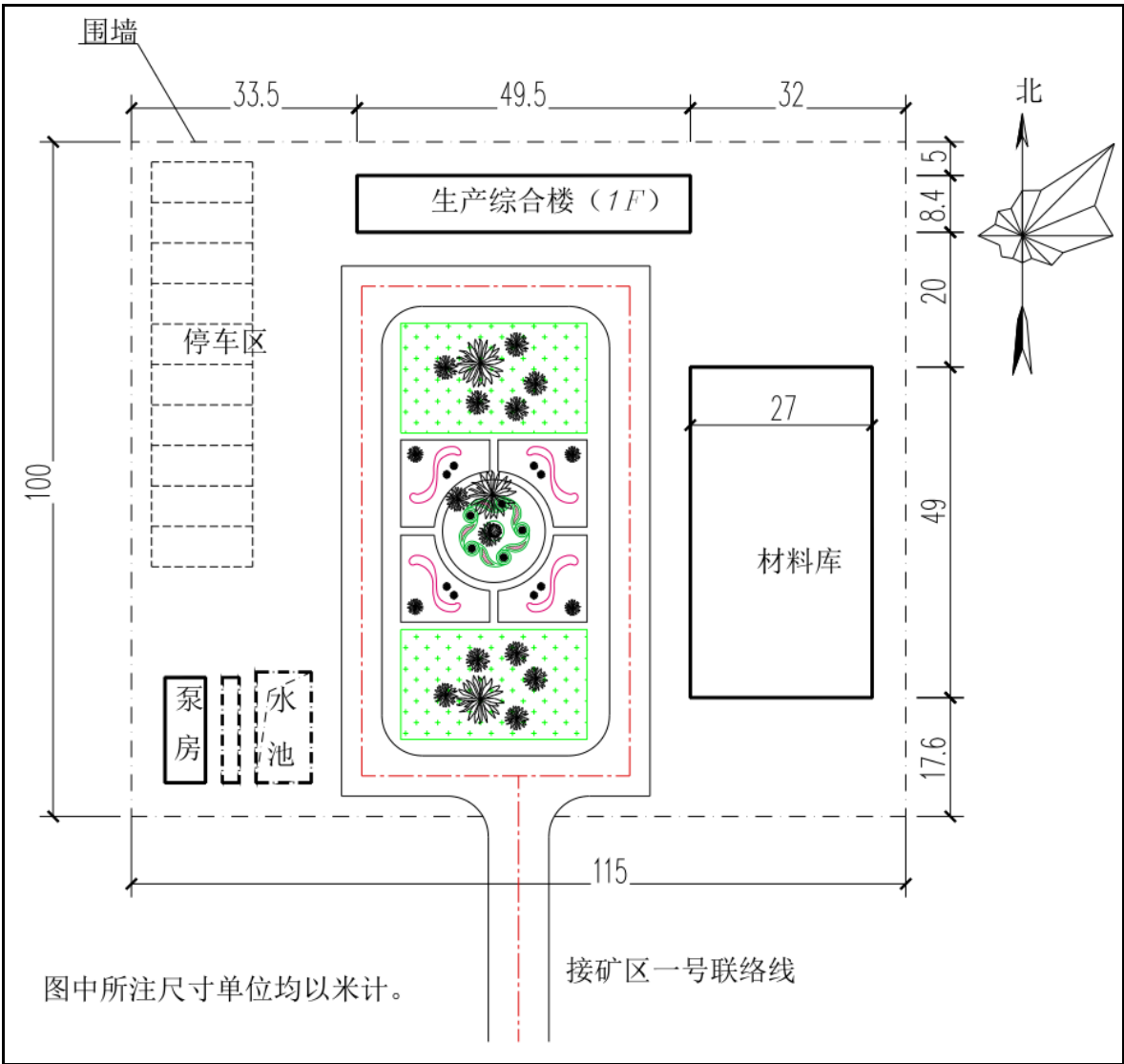
图 3.5-2 配套工程总平面布置图
