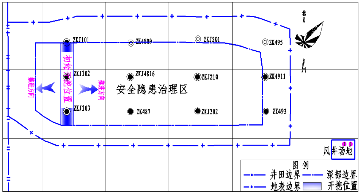
图 3.2-10 初始开挖位置及治理范围示意图
