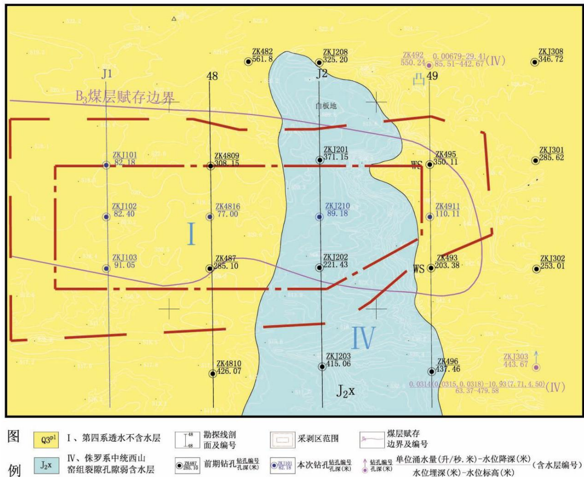
图 4.1-7 治理区含（隔）水层（段）分布图
