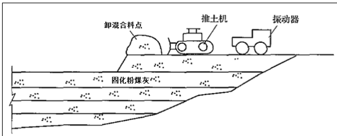
图 3.11-2 回填方法示意图
