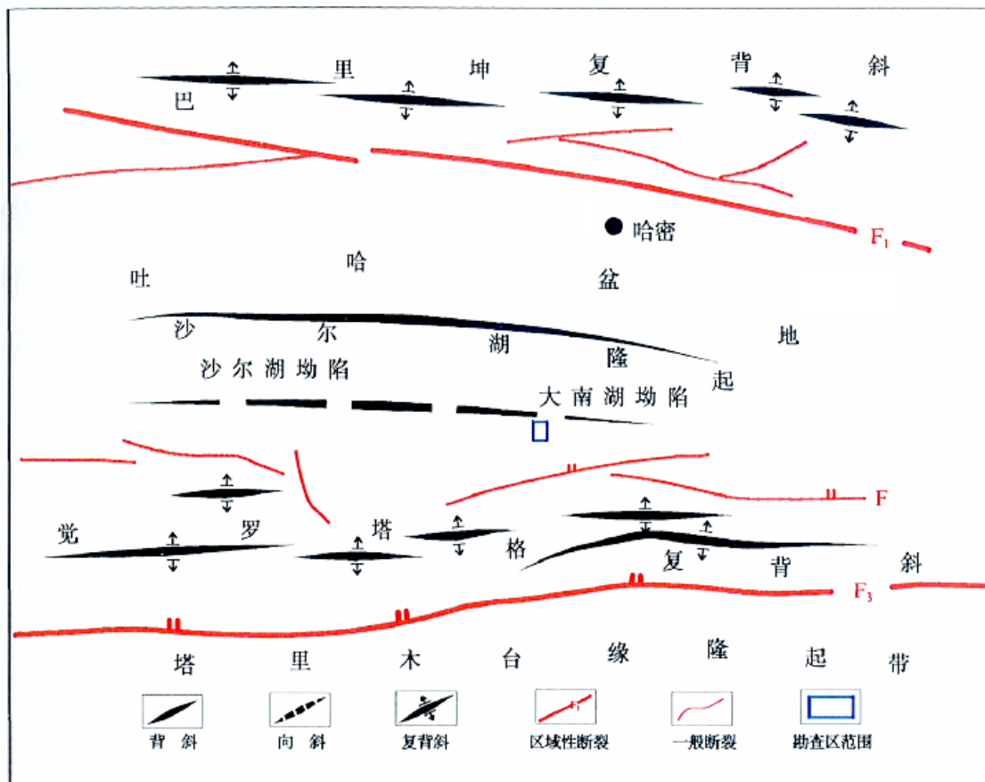
图 4.1-5 矿区区域地质构造略图
