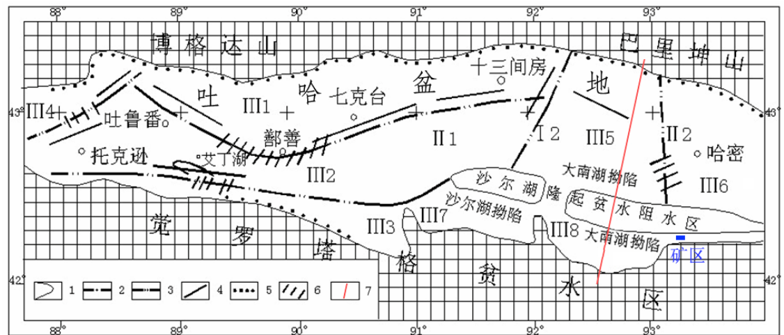
1.I级水文地质界线;2.II级水文地质界线;3.III级水文地质界线;4.断裂构造; 5.补给区;6.排泄区;7.哈密盆地次级水文地质单元剖面线(见下图 3-6);I 1 —水文地质地块;I 2 —潜水及承压水盆地;II 1 —吐鲁番拗陷潜水及深层承压水盆地;II 2 —哈密拗陷浅层潜水及深层承压水盆地。
