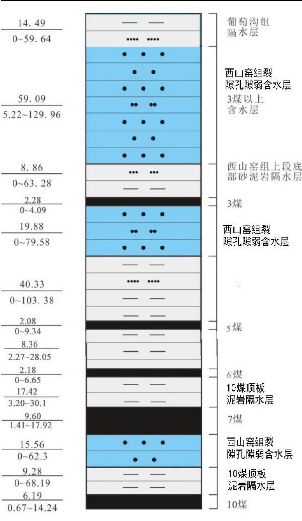
图 5.2-1 含（隔）水层垂向分布示意图
