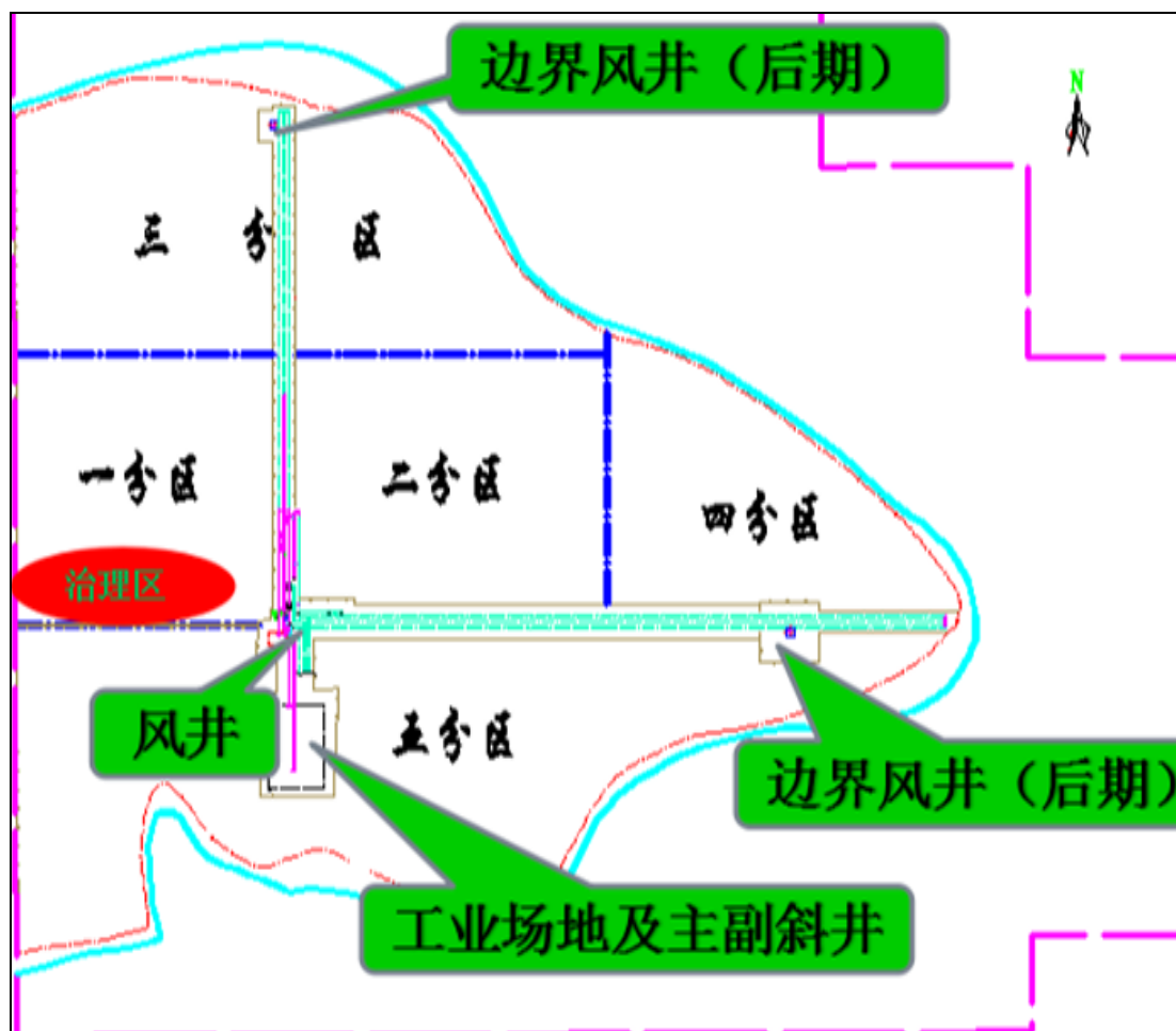
图 3.1-1 矿井分区划分图
