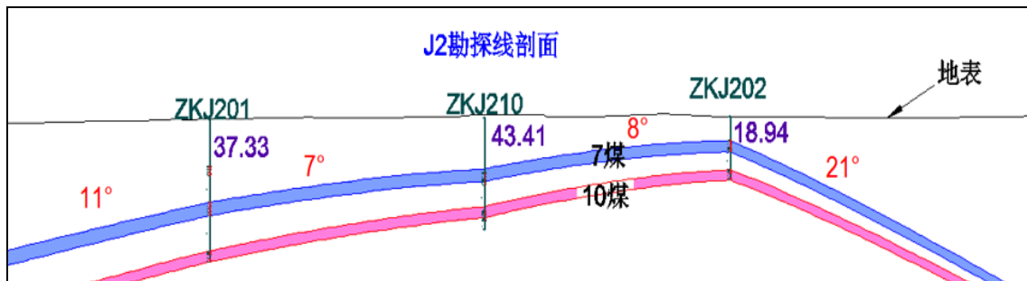
图 3.2-8 J2 勘探线剖面图
