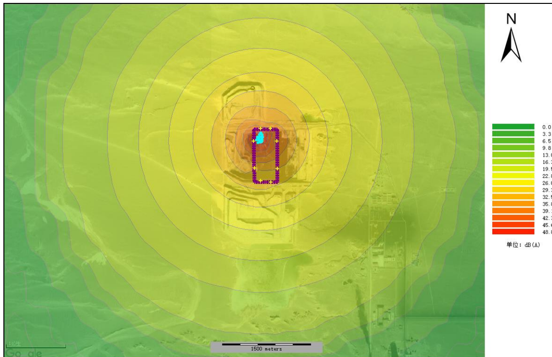
图 5.3-1 噪声预测结果图
