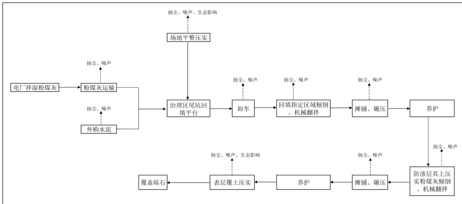
图 3.11-2 回填治理工艺流程及产污节点图
