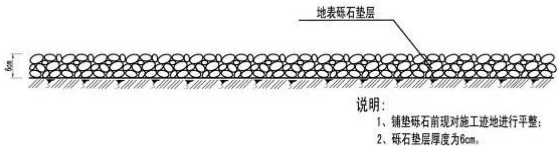
图 6.6-1 砾石压盖措施典型设计图
