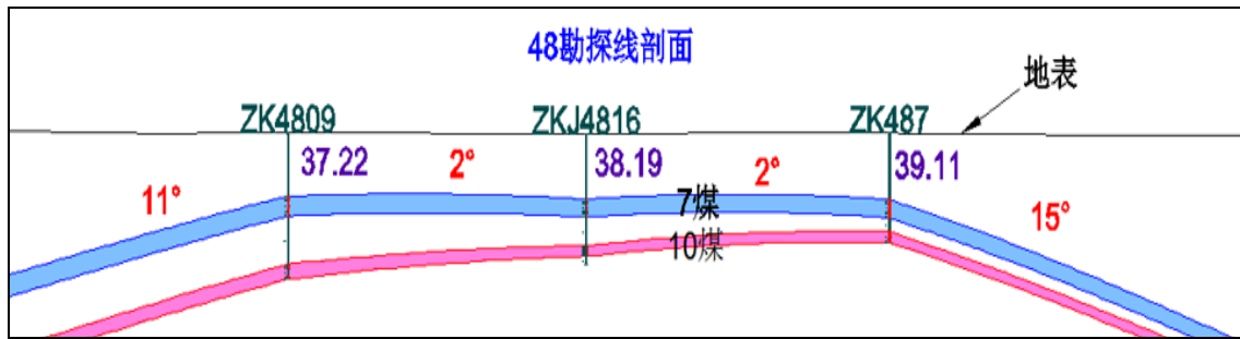
图 3.2-7 48 勘探线剖面图
