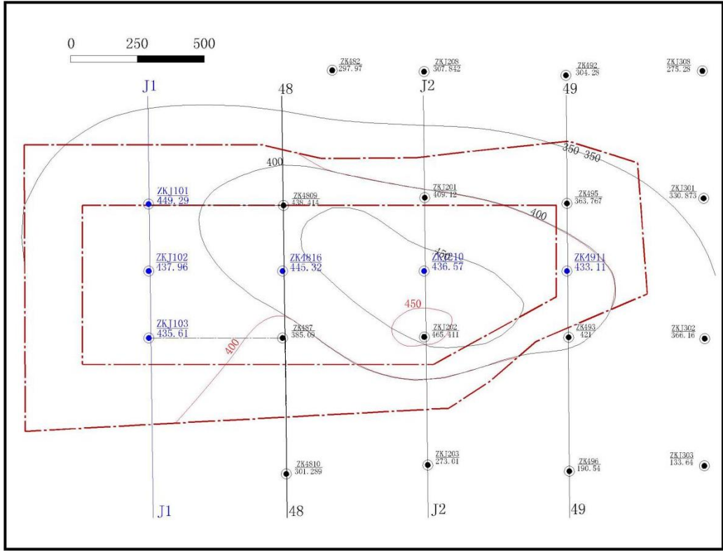
图 4.1-5 治理区 10#煤层底板等高线（图例同上）
