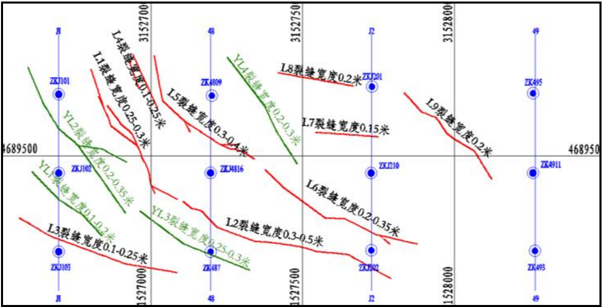
图 3.2-1 地表及施工过程中发现的裂隙分布图
