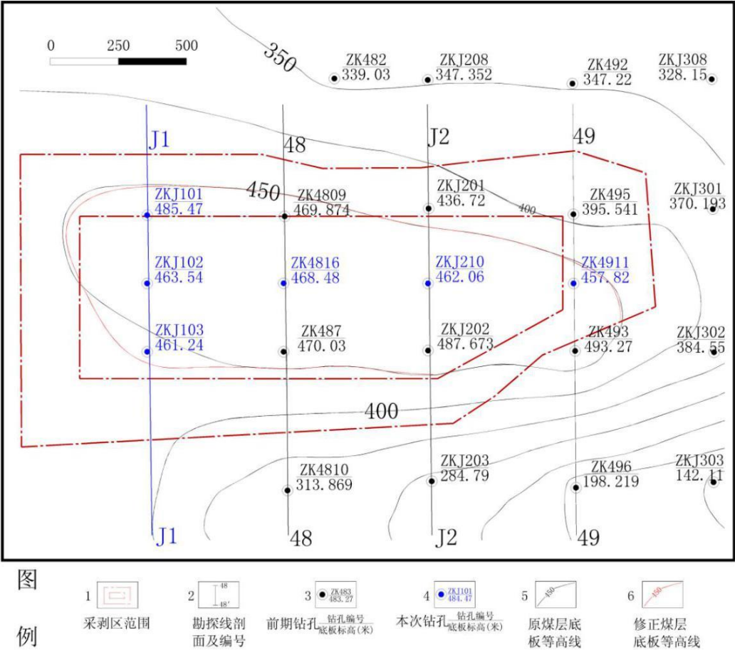
图 4.1-4 治理区 7#煤层底板等高线
