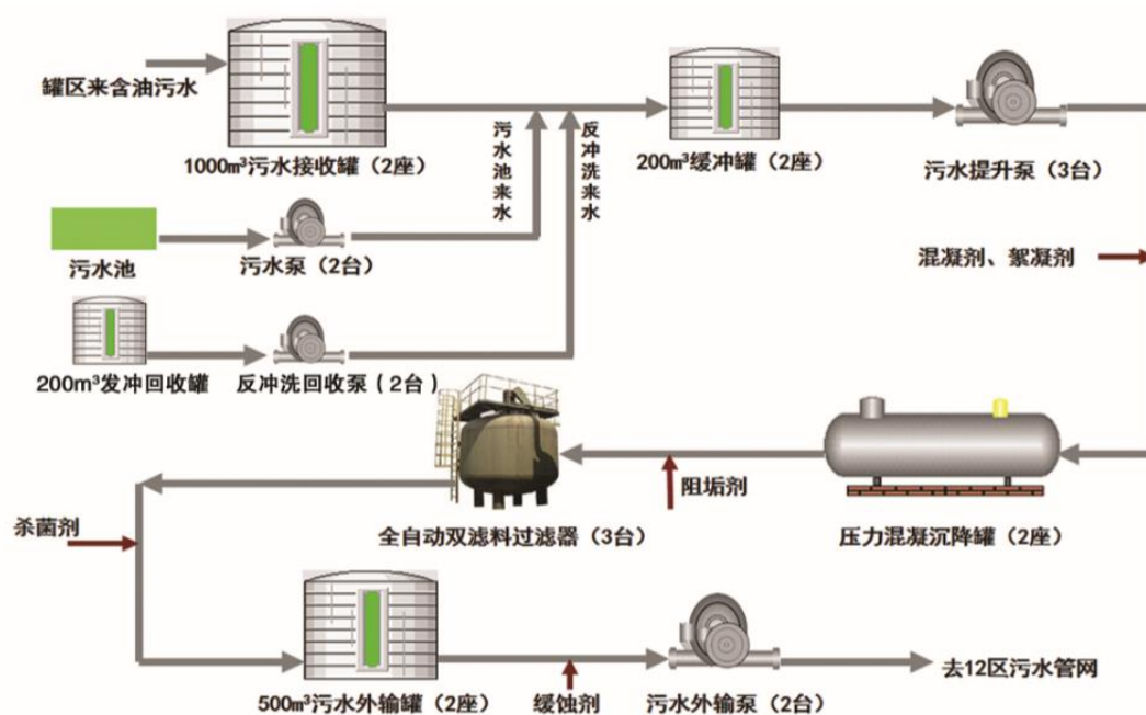
图 3.1-7 四号联合站污水处理系统工艺流程示意图
