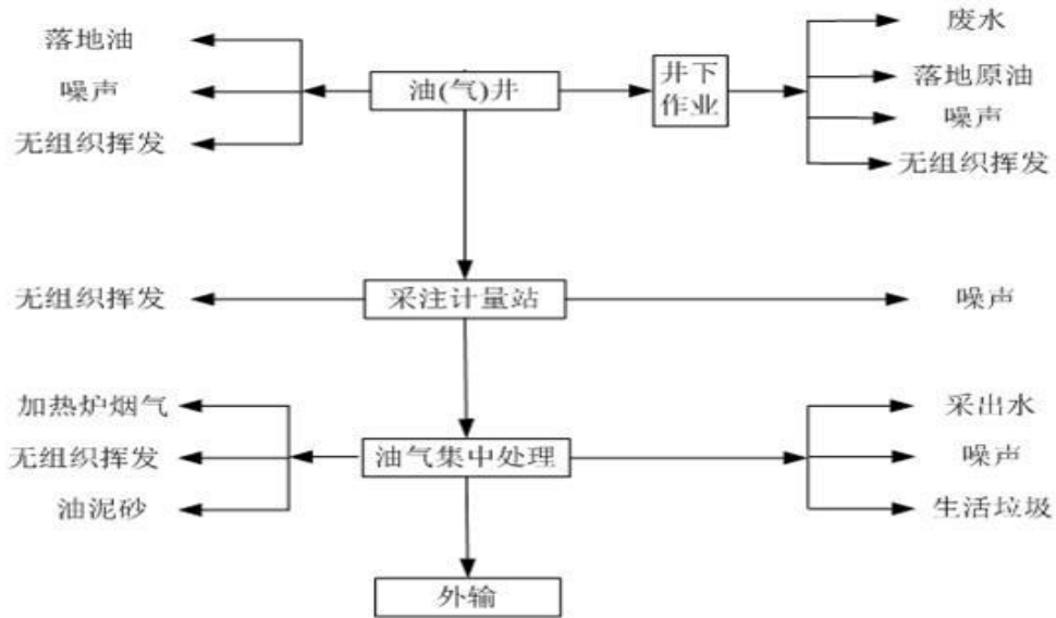
图 3.3-2 油田开发过程污染物排放流程
