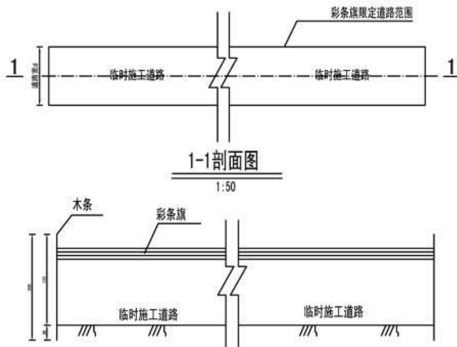
图 6.1-3 彩条旗拦挡典型设计图
