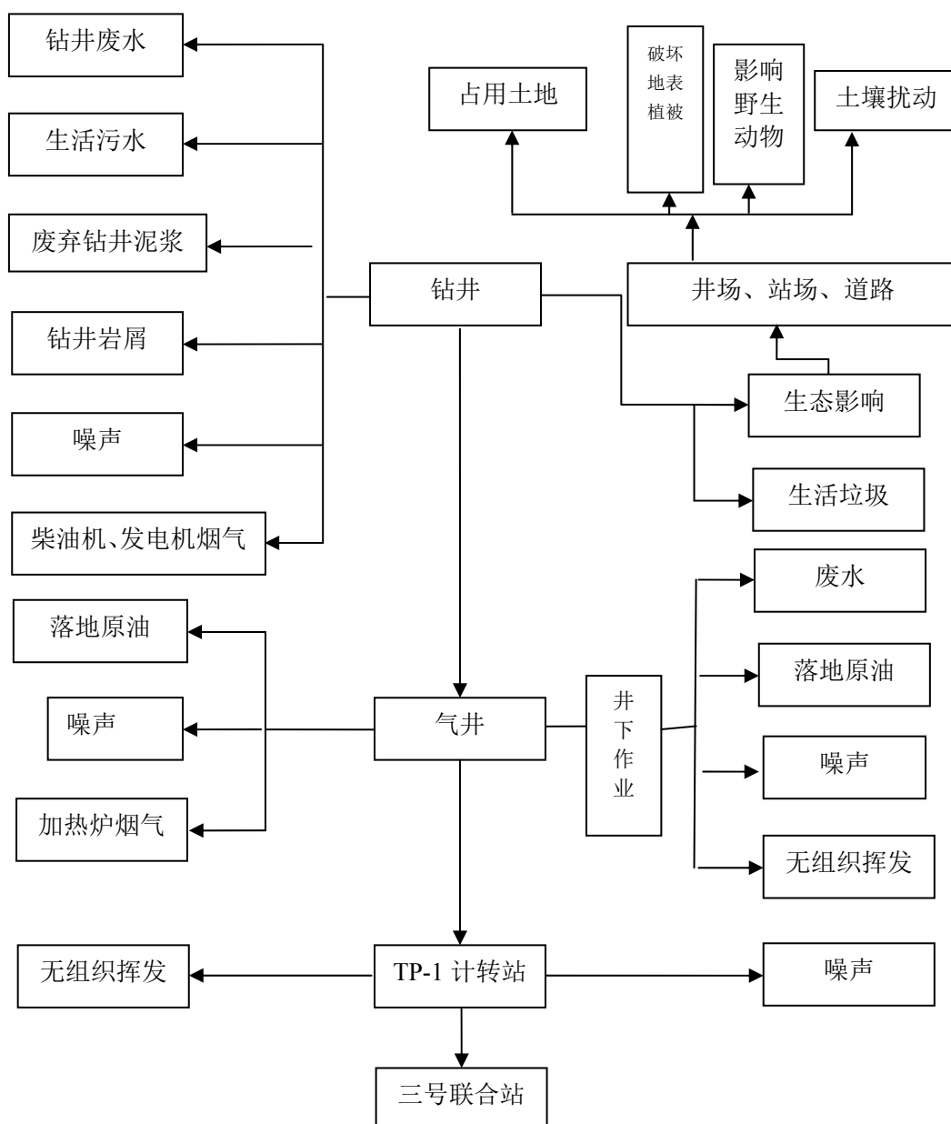
图 3.2-2 油气田开发过程污染物排放流程
