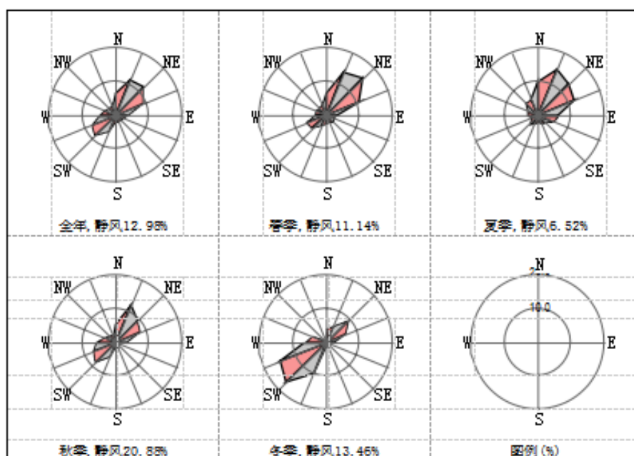
图 5.2-2 沙雅县 2019 年各季、全年风向玫瑰图
