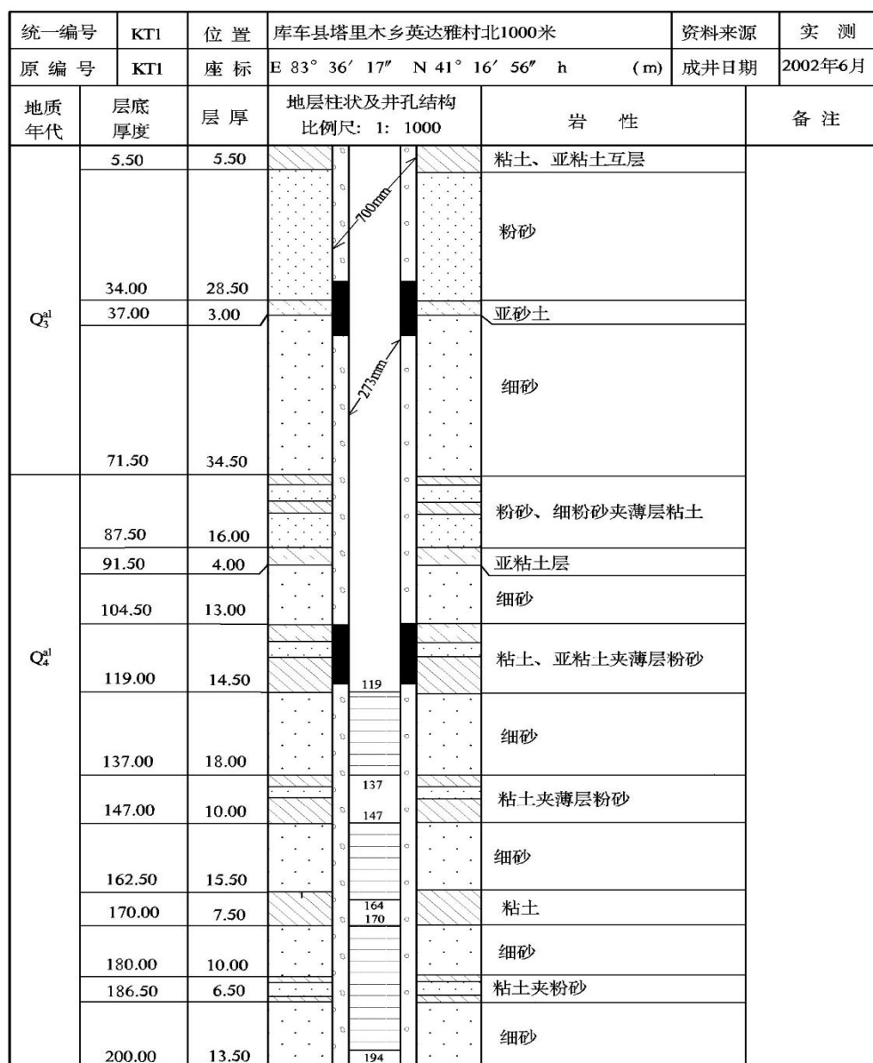
图 4.6-1 钻孔柱状图
