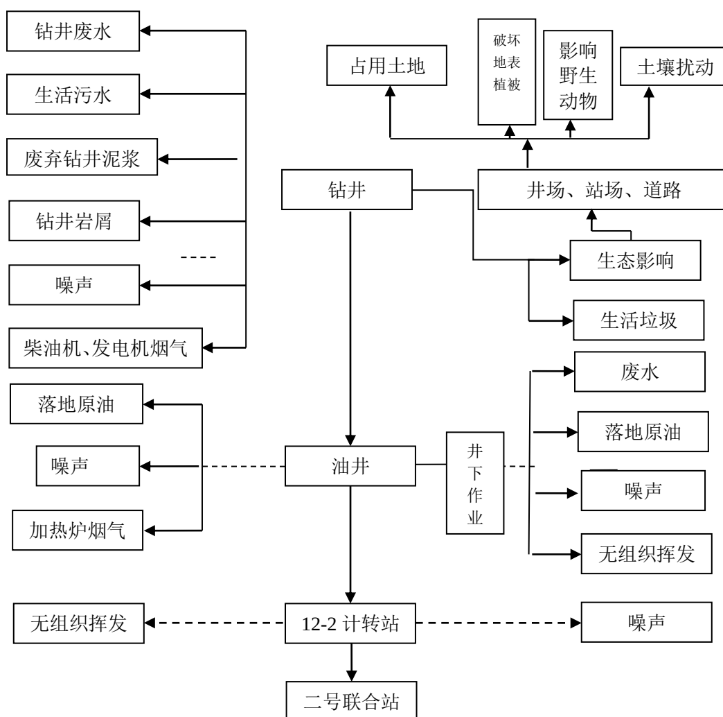
图 3.2-2 油田开发过程污染物排放流程
