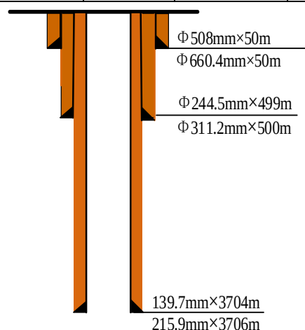
图 3.1-3 TKE1-1 井井身结构示意图
