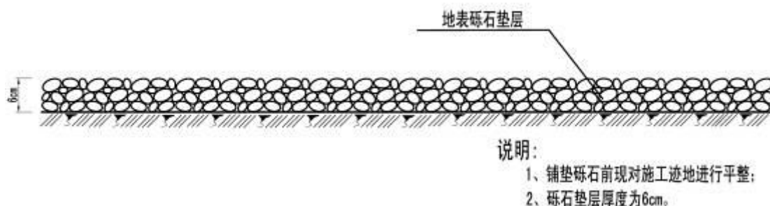
图 6.1-2 井场、站场砾石压盖措施典型设计图
