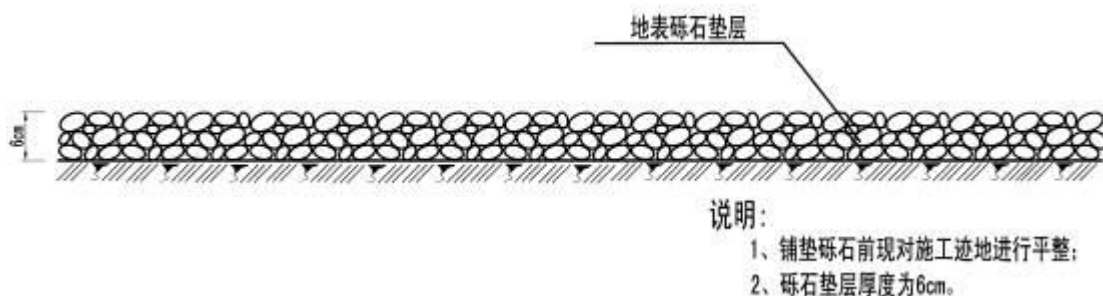
图 6.1-1 井场、站场砾石压盖措施典型设计图
