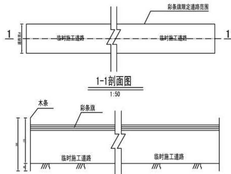
图 6.1-3 彩条旗拦挡典型设计图
