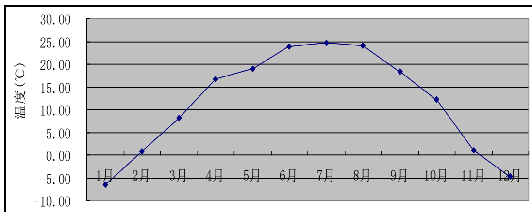
图 5.2-2 2020 年平均温度月变化统计图
