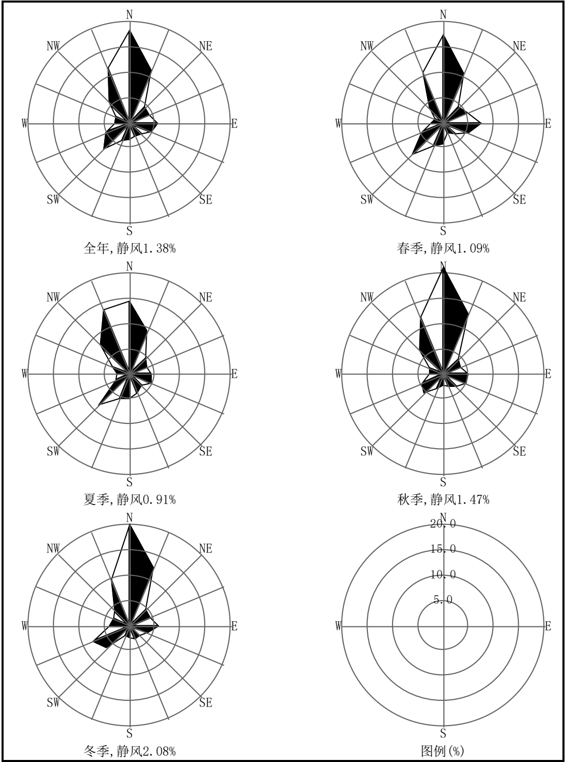
图 5.2-1 库车市 2019 年全年及各季度风向玫瑰图
