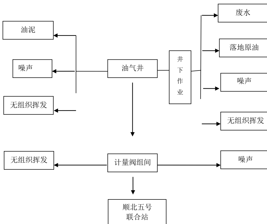
图 3.2-2 本项目开发过程污染物排放流程简图
