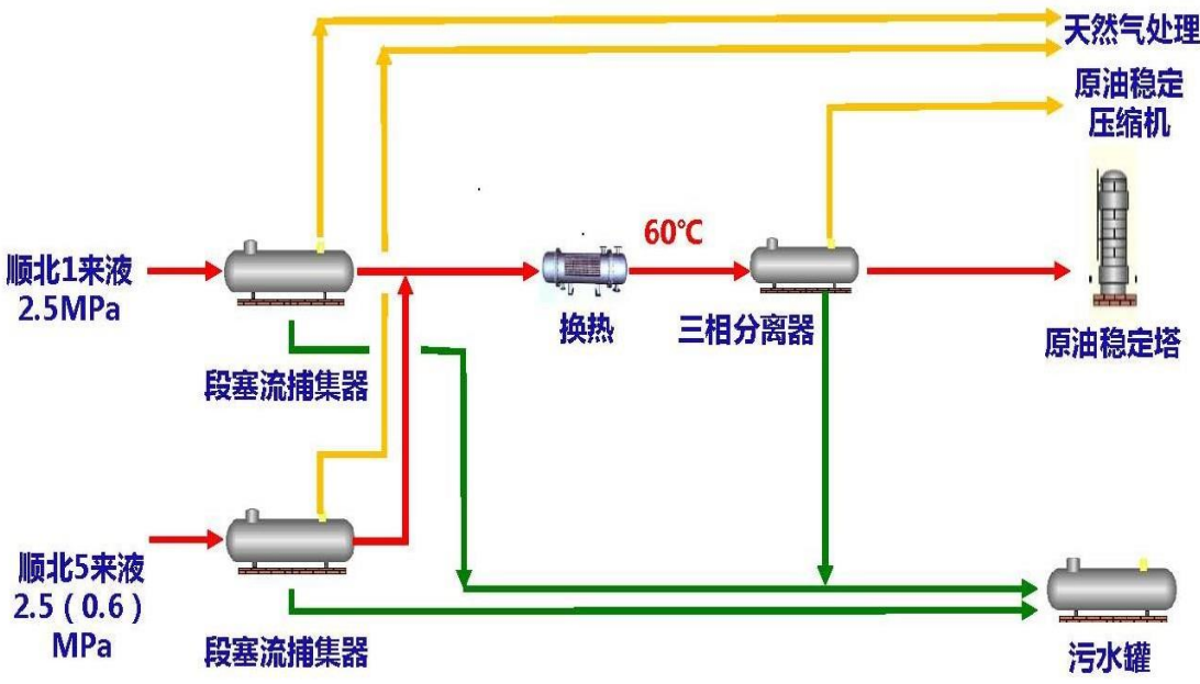
图 3.1-5 五号联合站原油处理工艺
