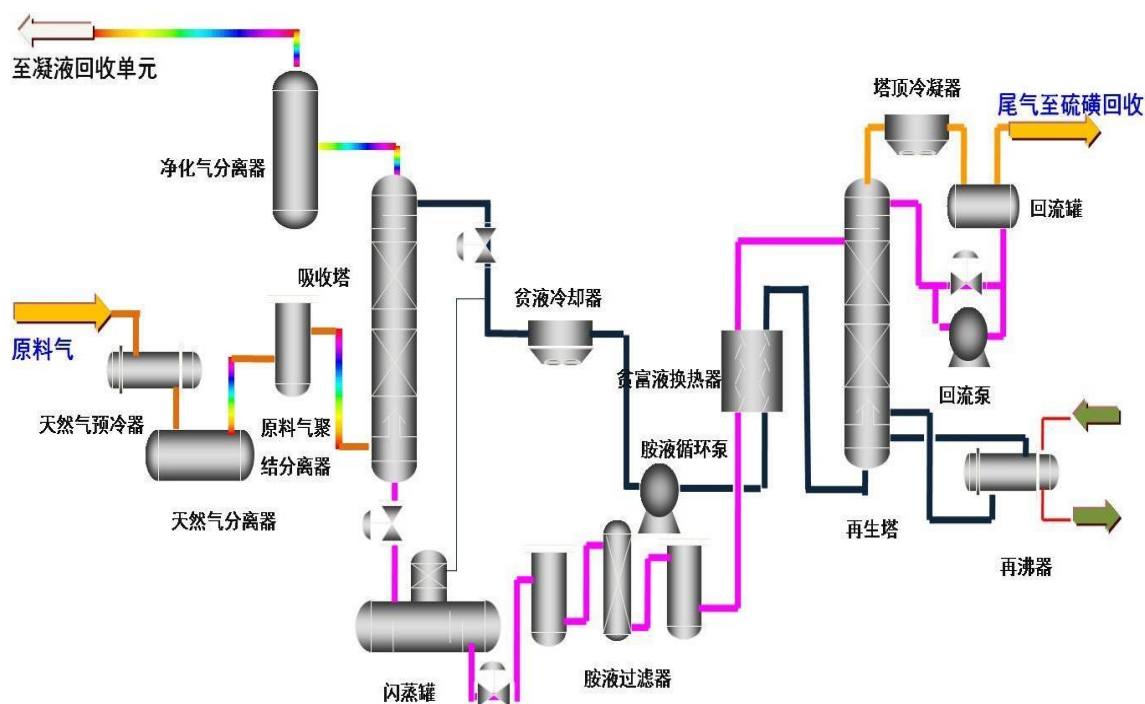
图 3.1-8 砵胺法脱硫部分工艺流程图
