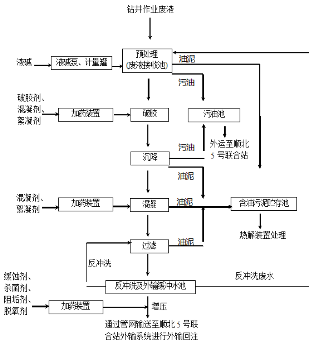
图 3.1-11 废液处理工艺流
