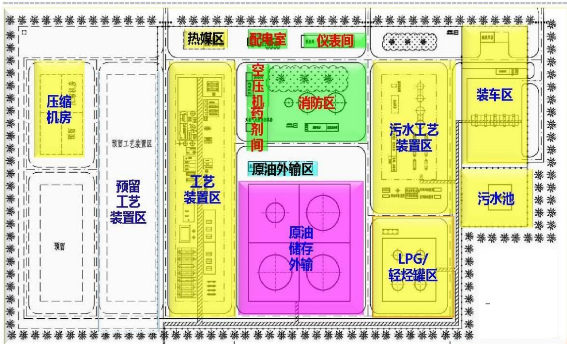
图 3.1-4 五号联合站平面布置示意图
