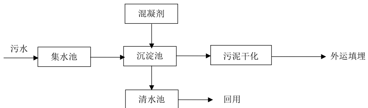
图 7.2-1 絮凝沉淀流程图
