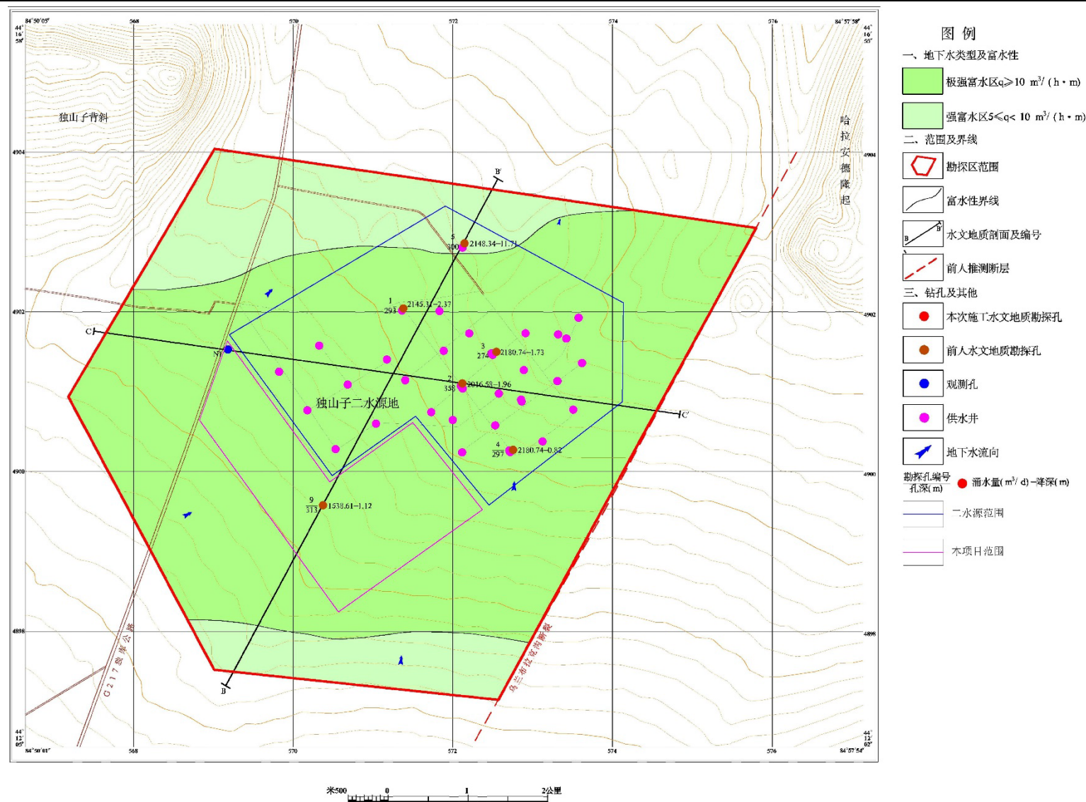
图 5.2-5 勘探区水文地质图
