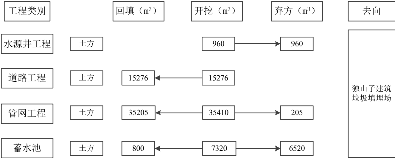
图 3.5-1 土石方平衡图
