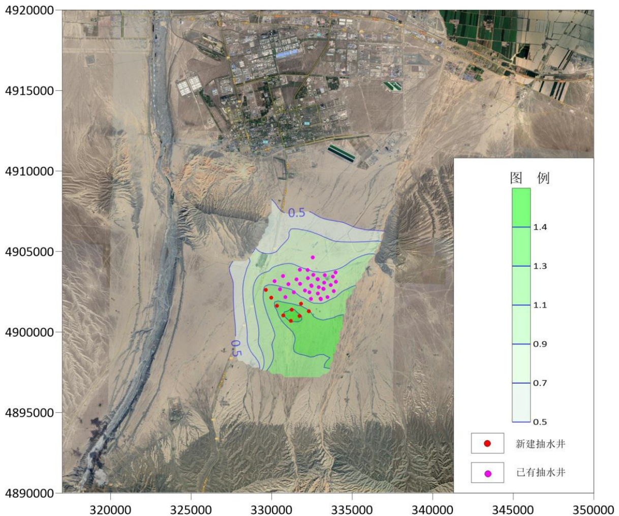
图 5.2-22 预测 30 年降深等值线图
