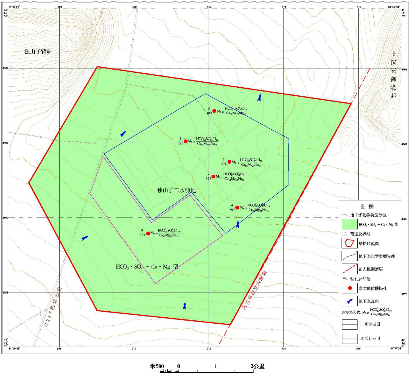
图 5.2-8 勘探区地下水化学类型图 表 5.2-6 勘探区地下水化学类型一览表
