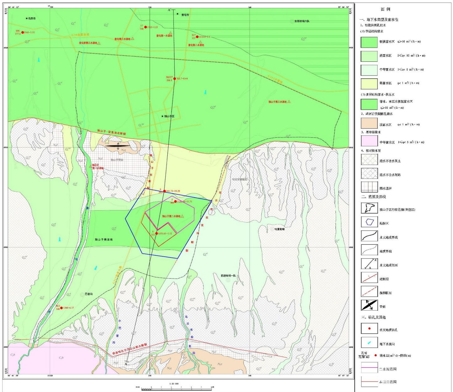
图 5.2-2 区域水文地质图
