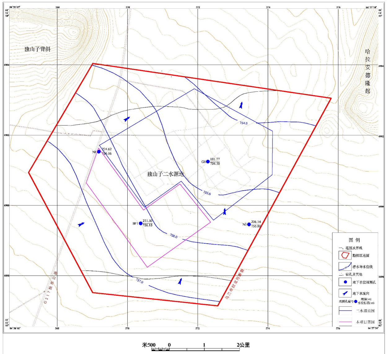
图 5.2-7 勘探区等水位线图
