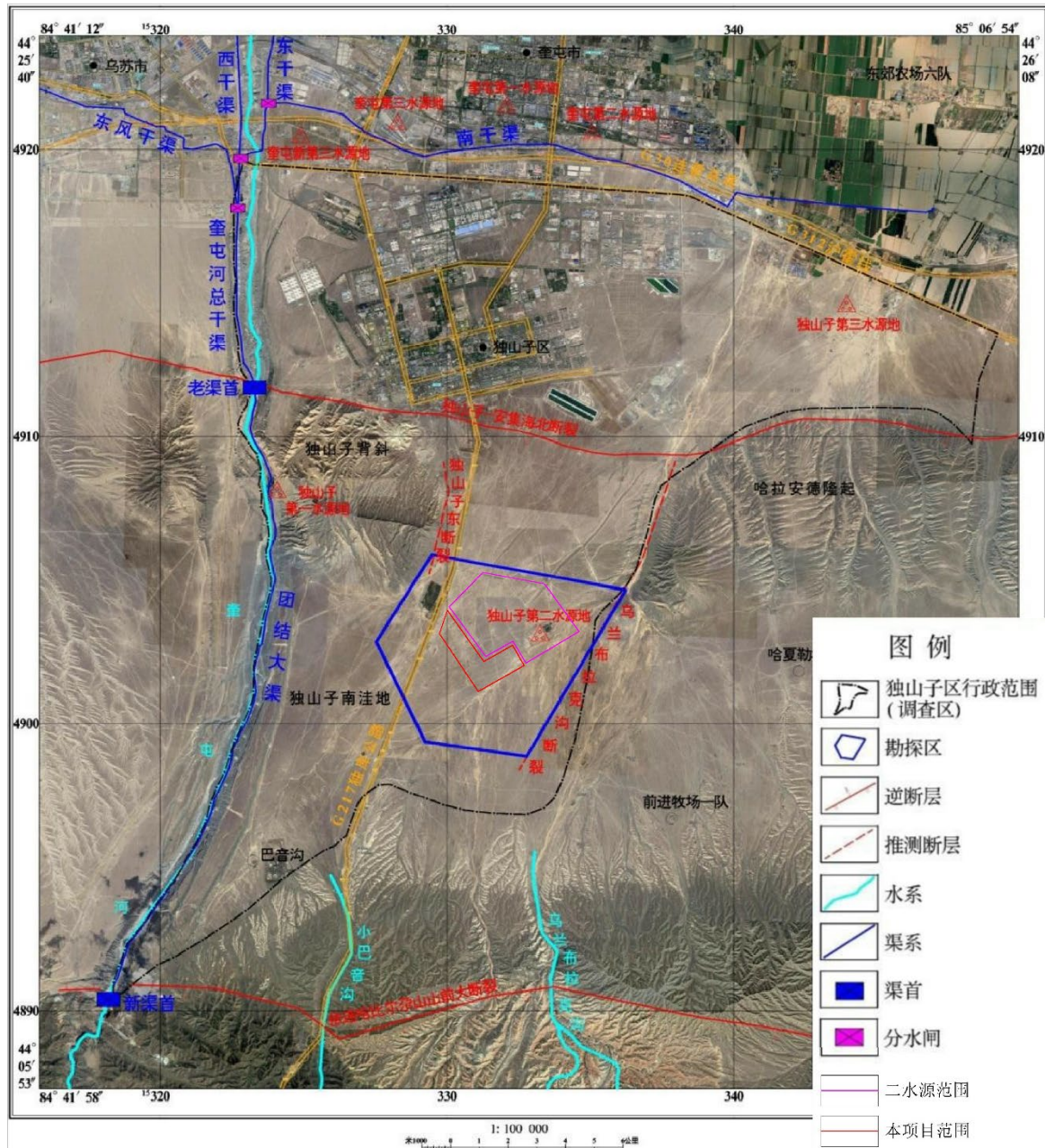
图 4.1-4 区域水系分布图
