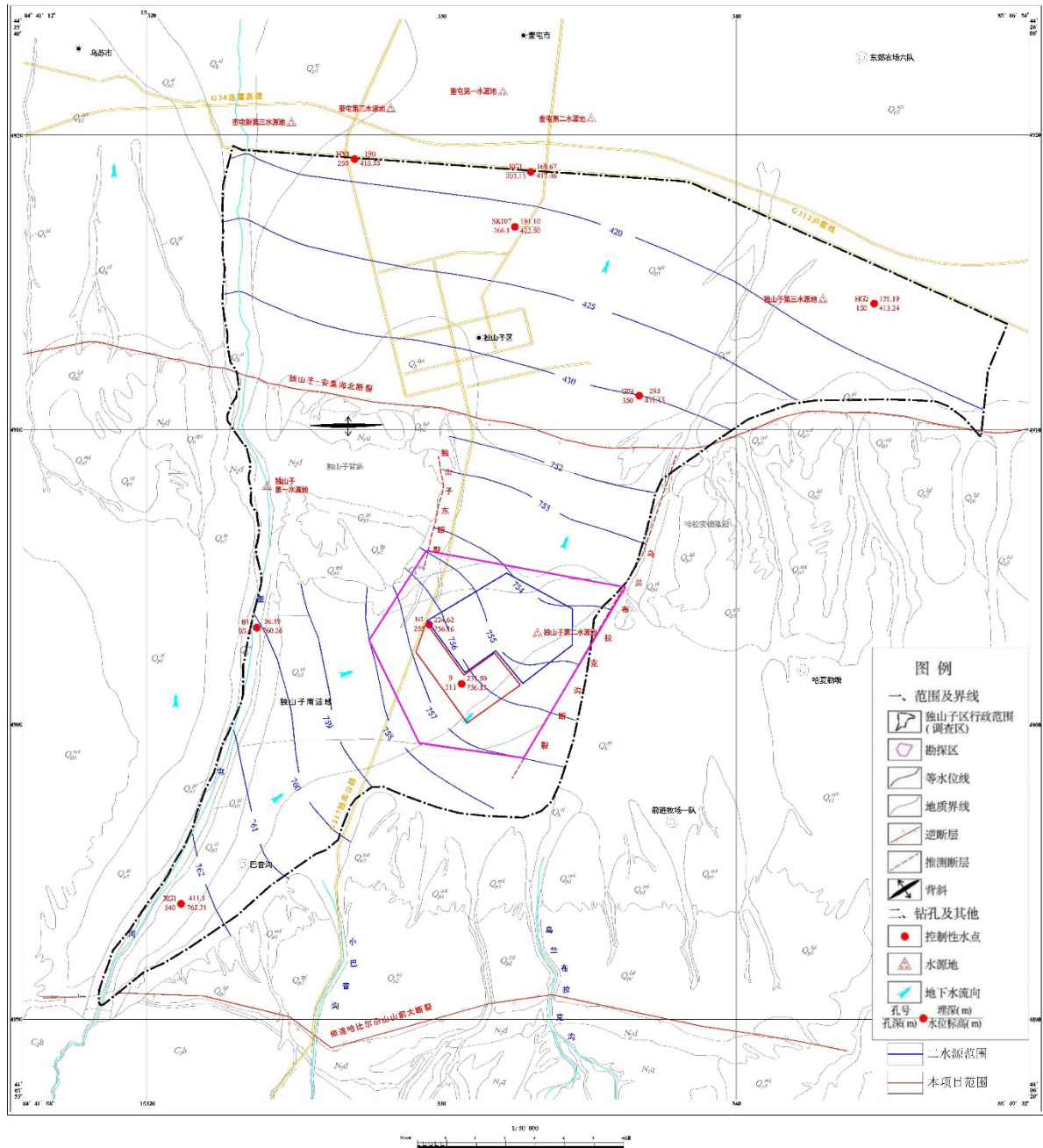
图 5.2-6 区域等水位线图
