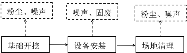
图 3.3-1 施工期工艺流程及产污节点图
