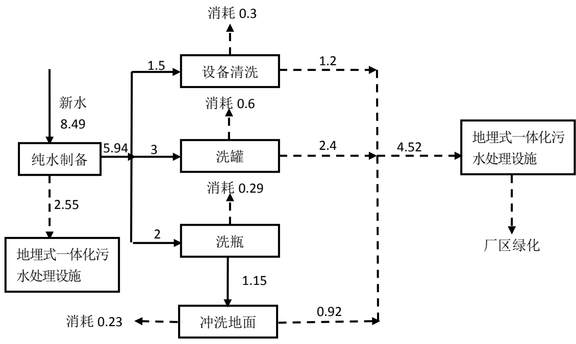
图 3.4-8 非榨汁季工程水平衡图 单位: m 3 /d
