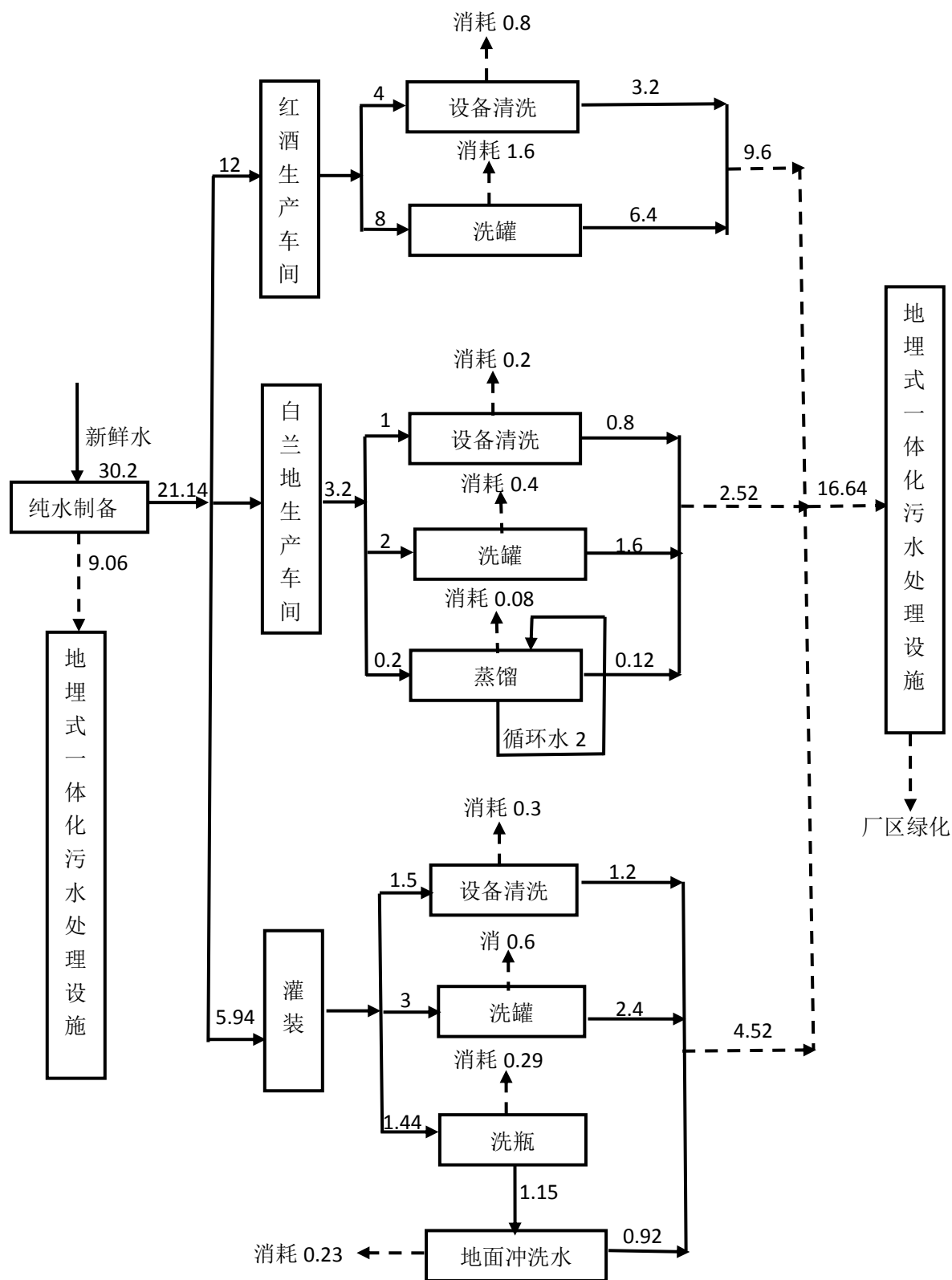
图 3.4-9 榨汁季工程水平衡图 单位: \text{m}^3/\text{d}
