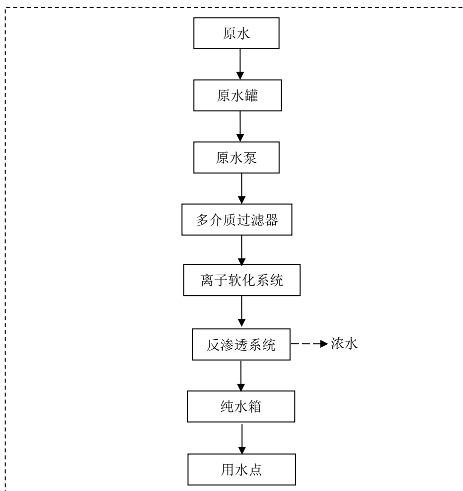
图 3.4-3 纯水工艺流程及产污节点图
