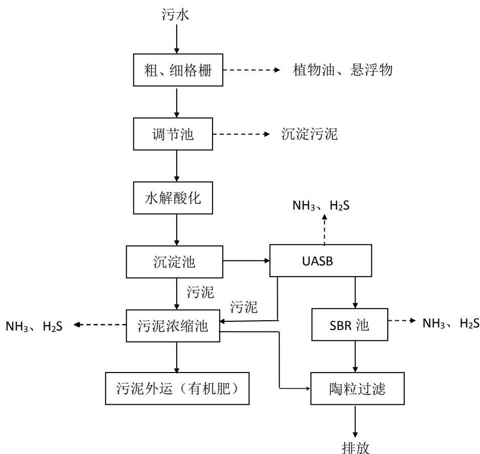
图 3.4-4 废水处理工艺流程图
