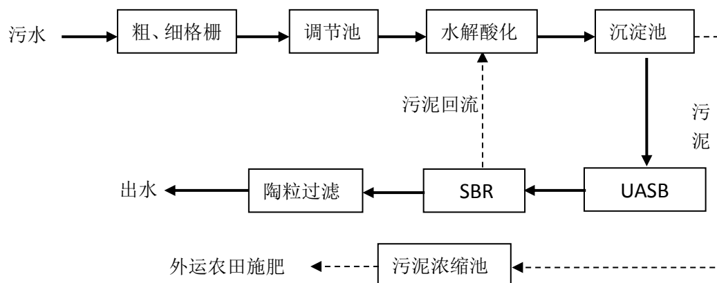
图 6.2-1 污水处理工艺流程
