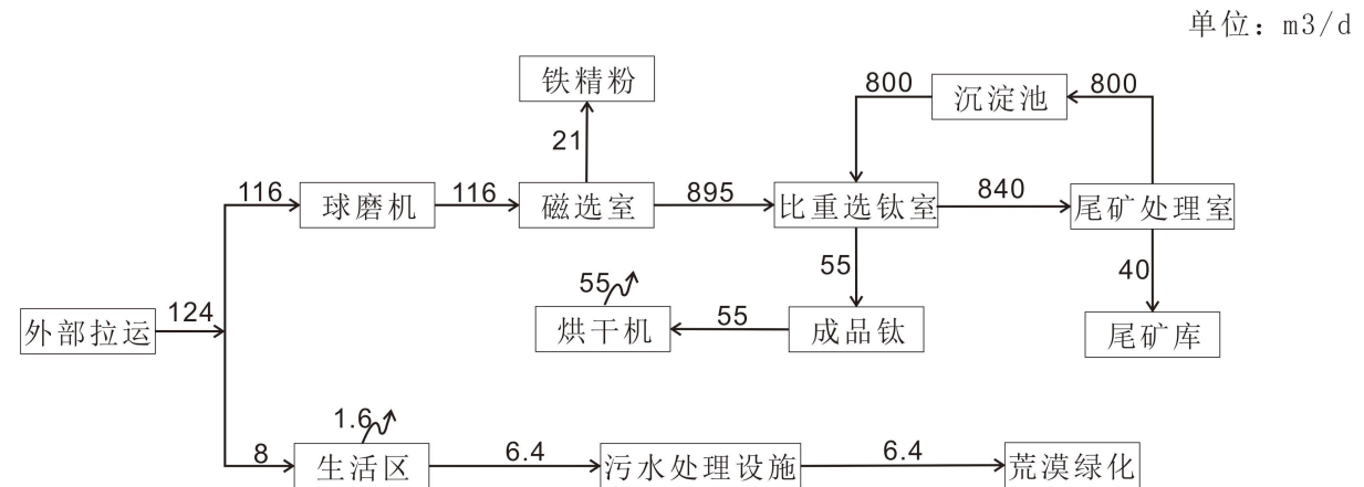
图 3.2-1 项目水平衡图 (m 3 /d)
