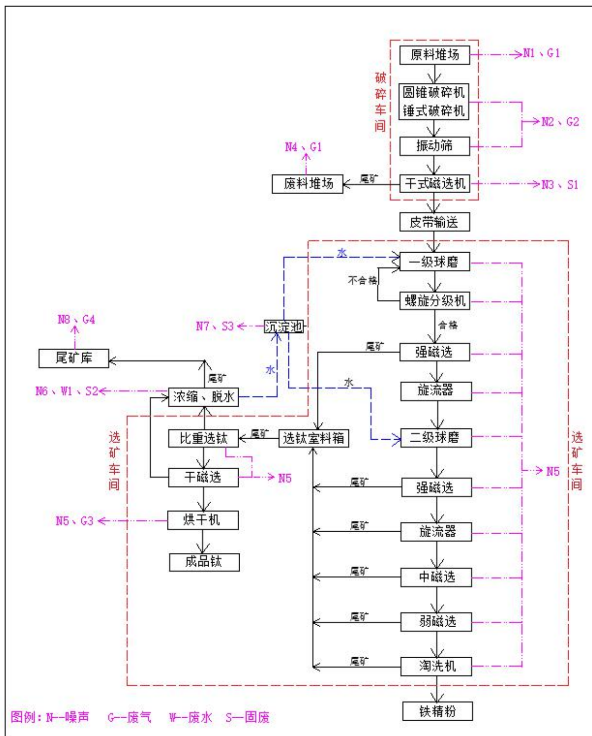
图 3.1-1 工艺流程及产污环节图
