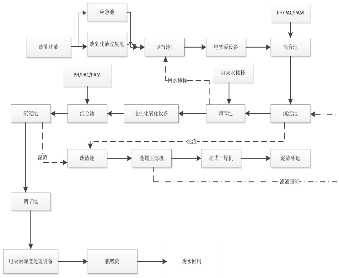
图 3.3-6 废乳化液处理工艺及产污流程图
