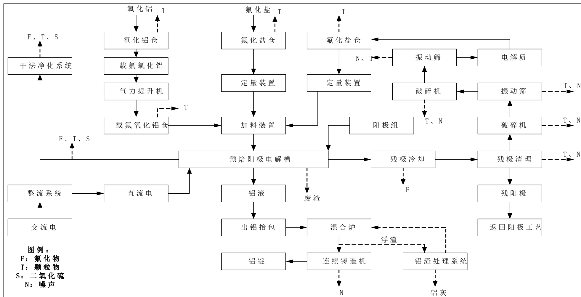
图 3-1-1 电解铝工程生产工艺及产污环节图
