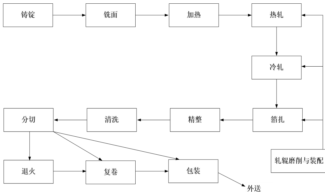
图 3-1-2 铝箔生产工艺及产污环节图
