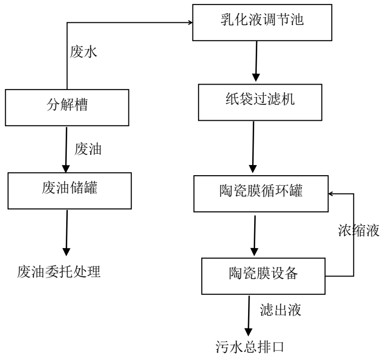
图 3-1-3 现有乳化液处理工艺
