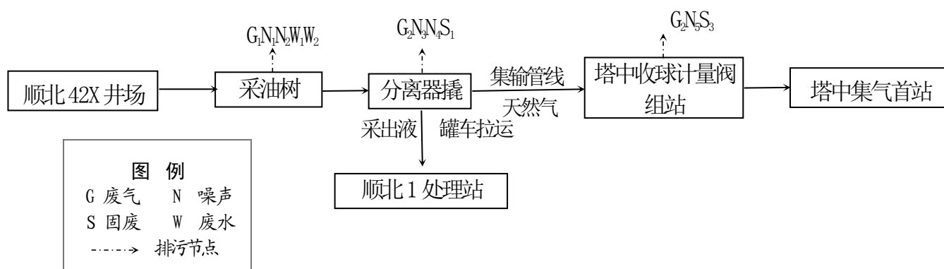
图 3.4-8 油气开采及集输工艺流程图
