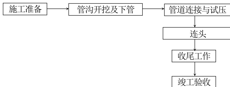
图3.4-4 管道工程施工阶段工艺流程图
