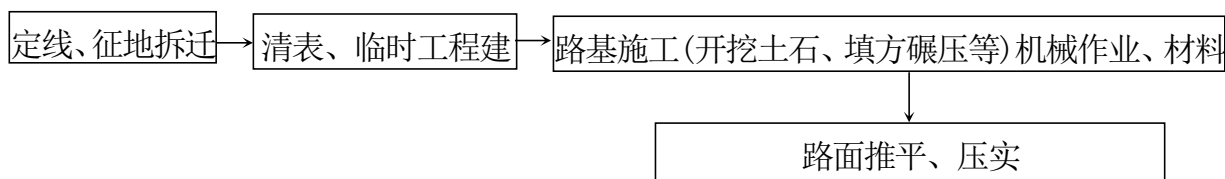
图 3.4-7 道路施工工艺流程图
