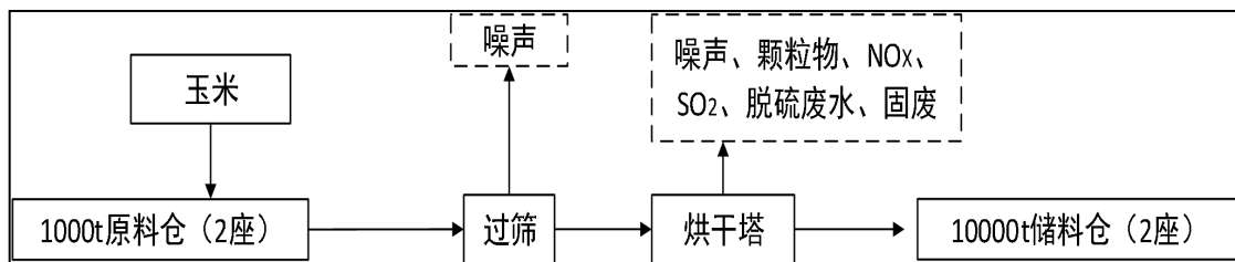
图 3.2-4 饲料加工工艺流程及产污环节示意图
