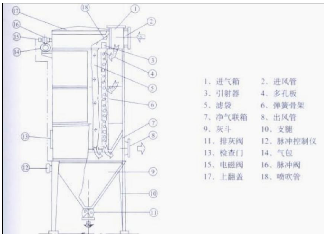
图 6.2-2 布袋除尘器的工作原理图
