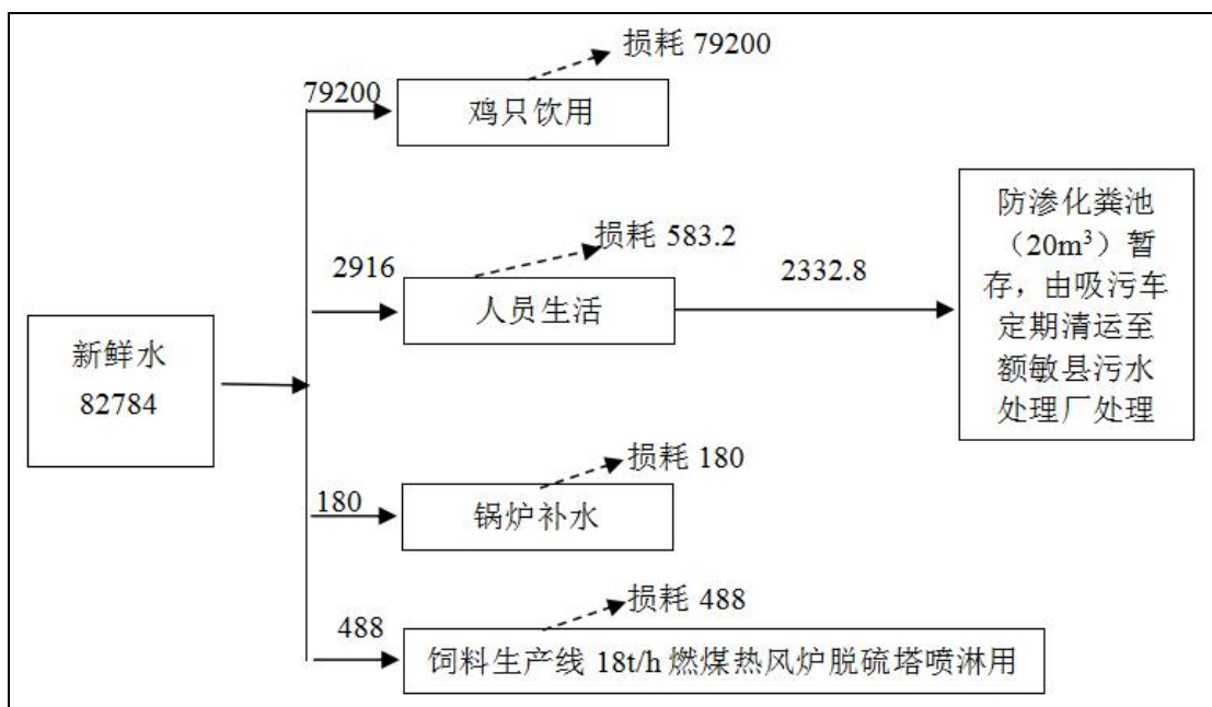
图 3.1-2 项目水平衡图 (单位: m³/a)
