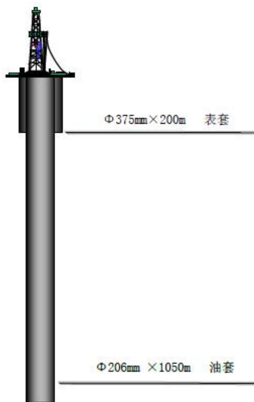
图 3.2-5 马 8 井块头屯河组井身结构示意图
