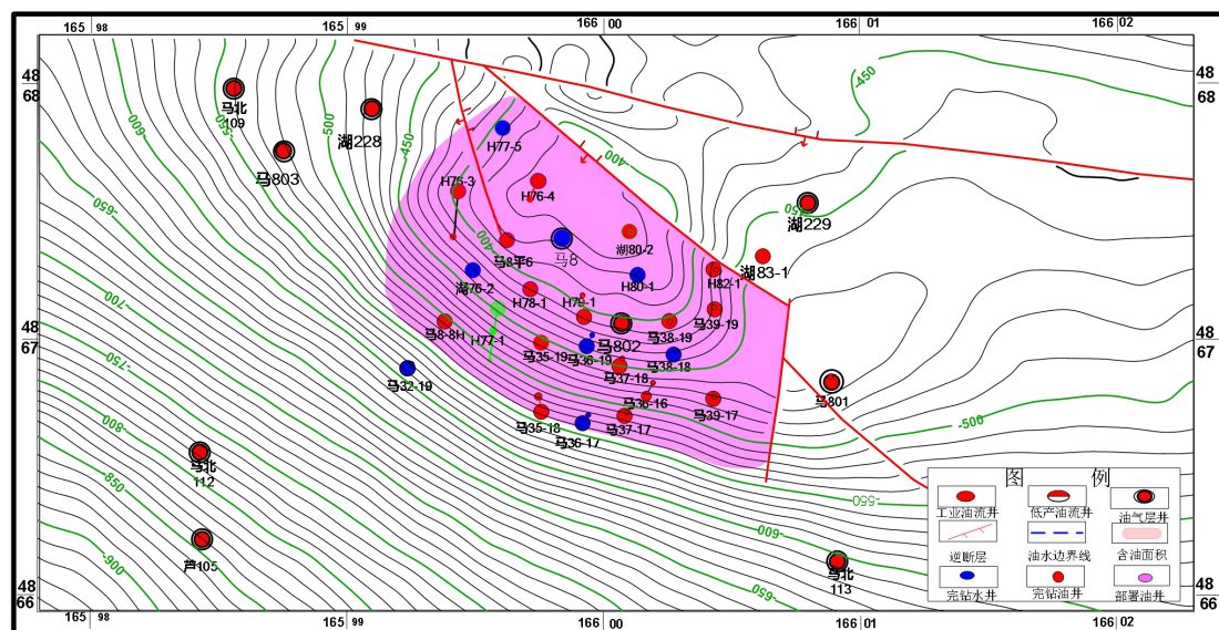
图 3.2-3 三塘湖油田马8井块头屯河组（一段）油藏底界构造井位图
