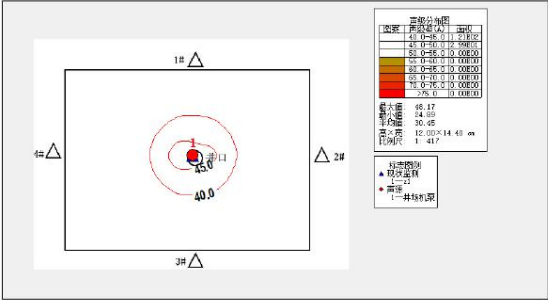
图 5.4-1 单井井场噪声预测结果图 由预测结果可知，井场厂界四周噪声值均满足《工业企业厂界环境噪声排放标准》（GB12348-2008）2 类标准限值要求，且周边无环境敏感点，因此工程实施后不会对周围声环境产生明显影响。
