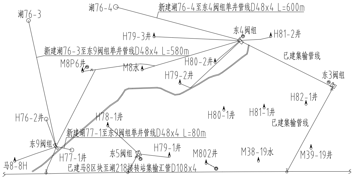
图 3.2-7 马 8 井区单井管线走向图
