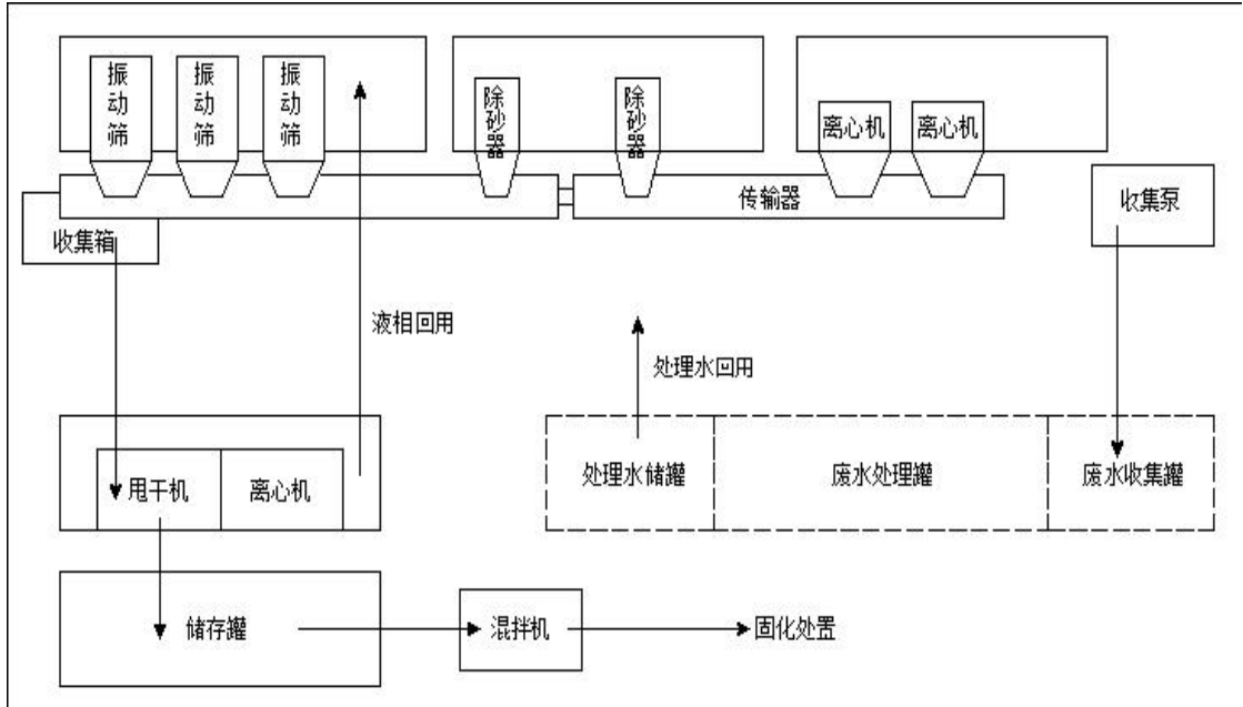
图 6.3-1 钻井废弃物不落地处理工艺流程示意图
