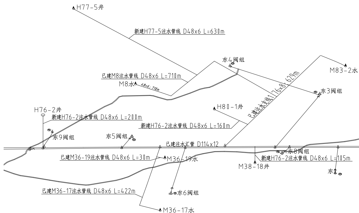
图 3.2-8 马8块注水管网图
