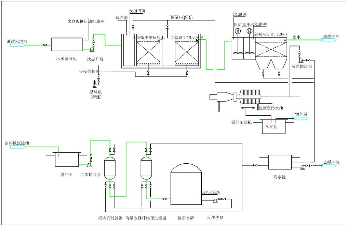
图 3.2-12 牛圈湖联合站污水处理工艺流程图
