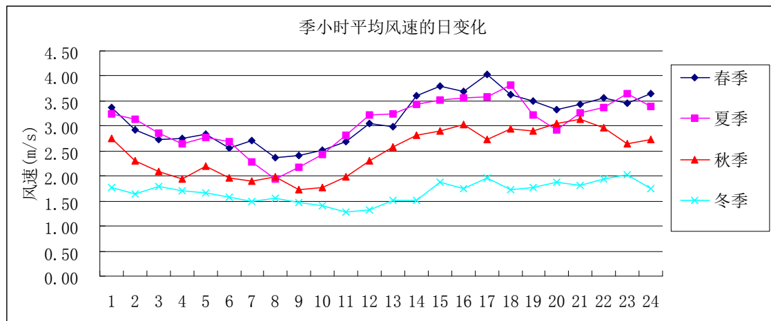
图 5.1-3 巴里坤哈萨克自治县 2018 年各季小时风速的日变化曲线
