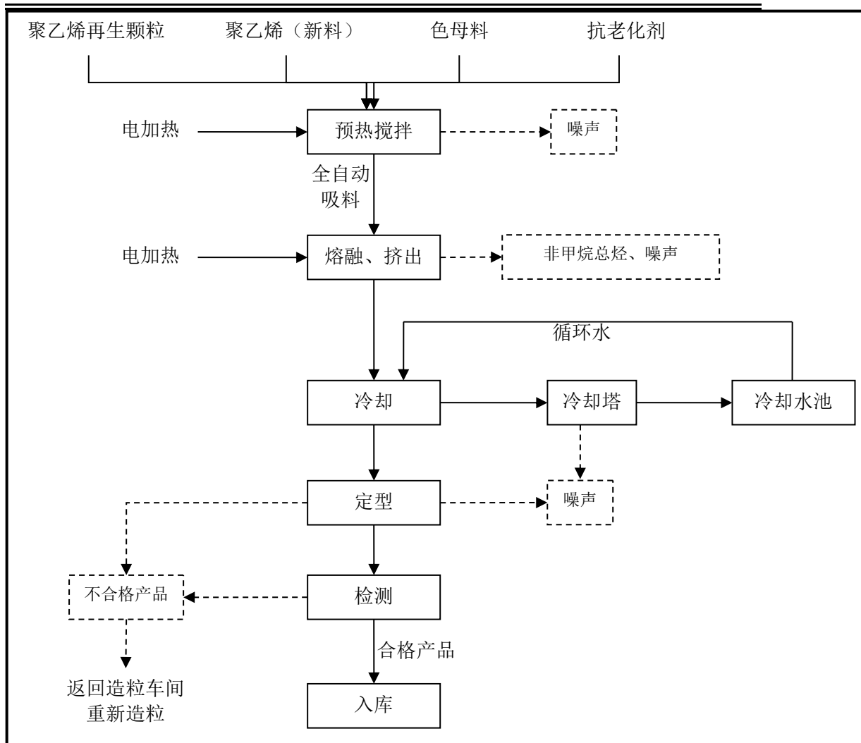
图 2.2-2 滴灌带、软管生产线工艺流程及产污节点图
