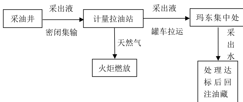
图 3.3-8 夏盐 19 井区集输工艺流程图
