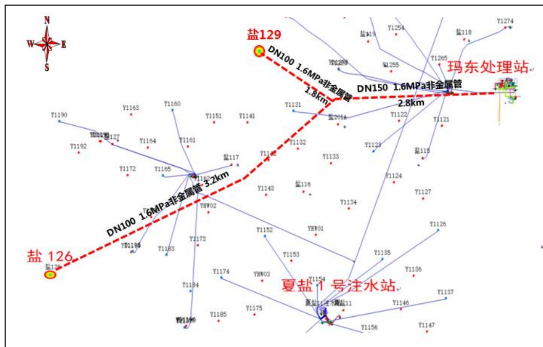
图3.2-8 注水管网平面布置图
