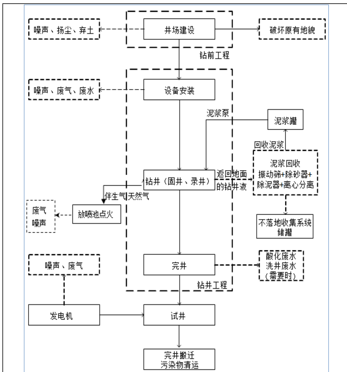
图 4-2 工艺流程和产污环节示意图
