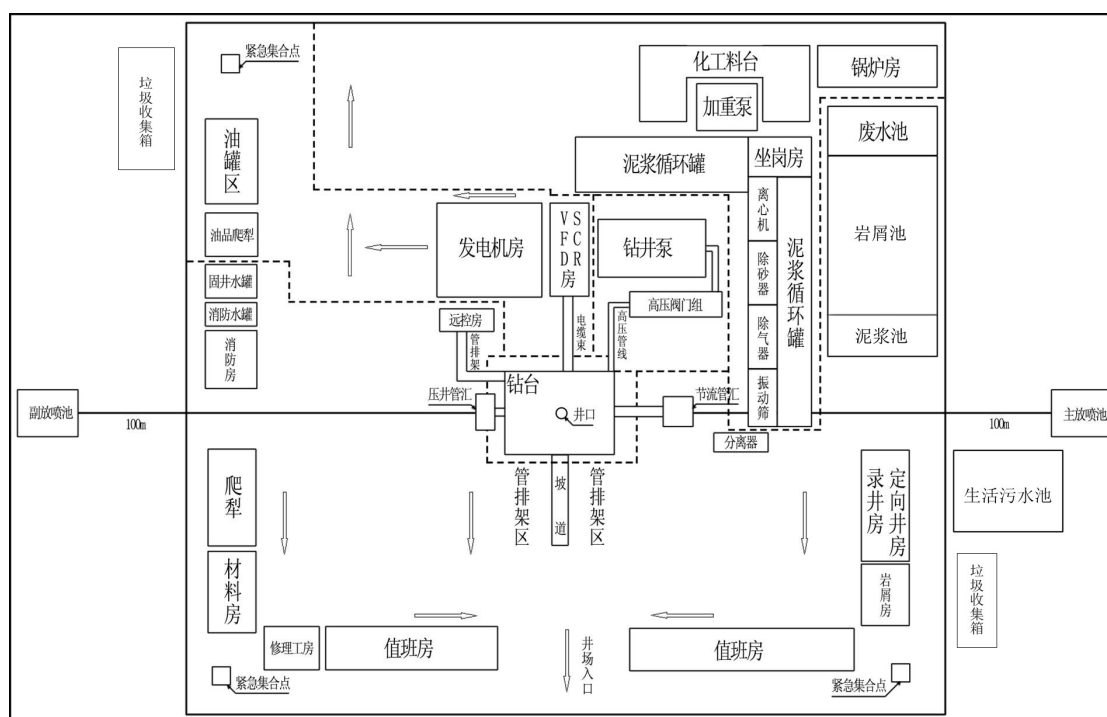
图 4-4 钻井井场平面布置图
