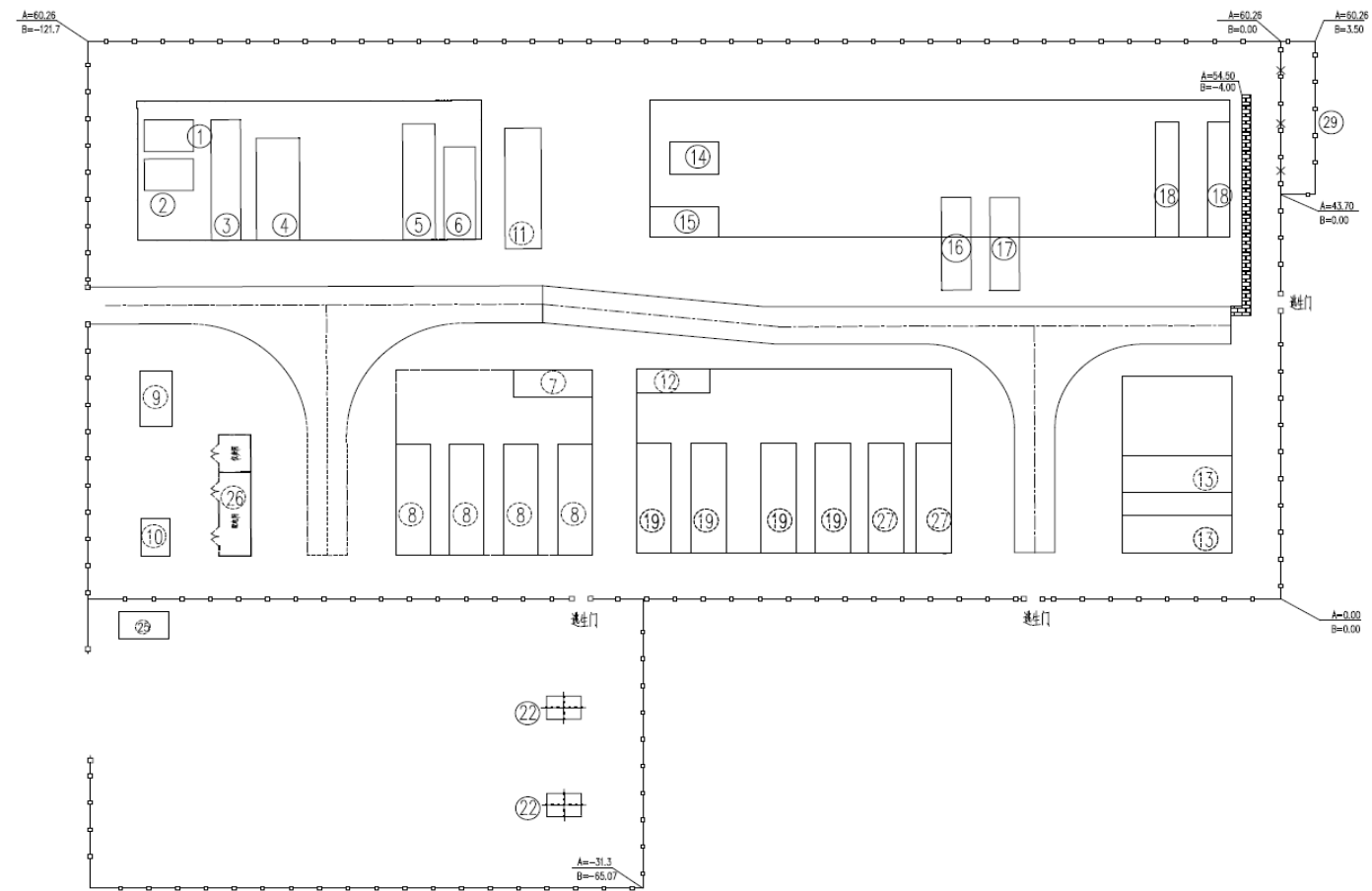
图 3.1-1 博孜1集气站现状平面布置图
